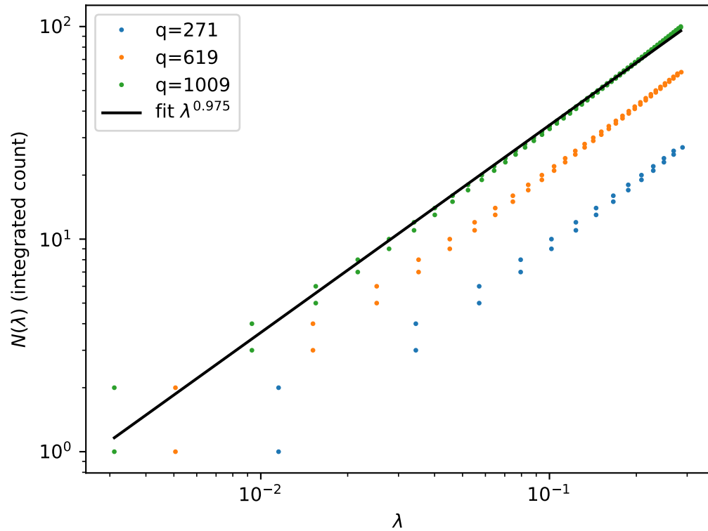
Edge integrated DOS
