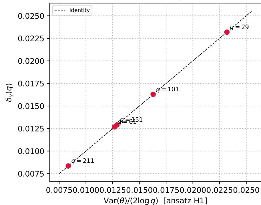
(D) Ansatz check [H1]: \delta_\gamma \approx \text{Var}/(2\log q)
