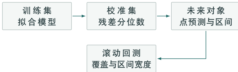
图 7.1 校准集与训练集承担不同任务；未来反馈用于监控适用条件。
