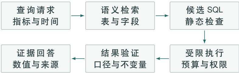
图 3.1 自然语言查询的生成、执行与结果检验
