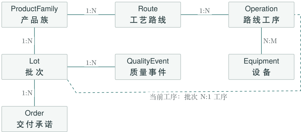
图 2.3 封装对象关系的教学抽象。虚线仅表示当前所在工序，历史流转另由事件表记录；工序与设备通过资格关系连接。
