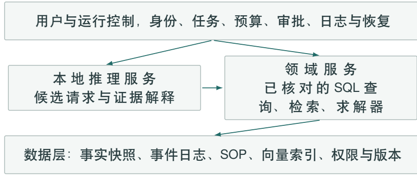
图 10.4 本地部署的数据、模型与运行服务
