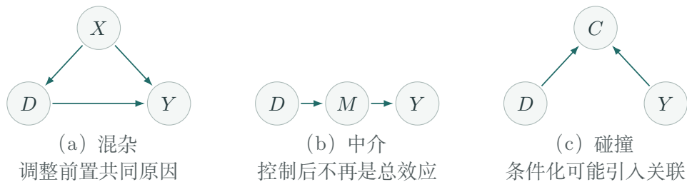
图 8.1 三个最小因果结构。图是业务机制假设，需要知识与证据支持。
