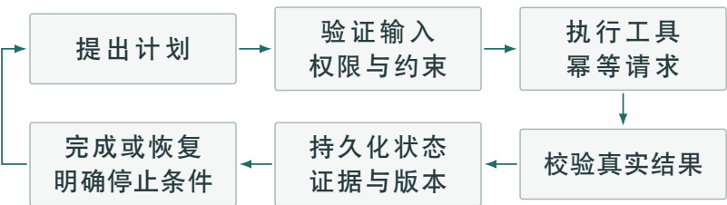
图 10.2 智能体的执行过程与故障恢复
