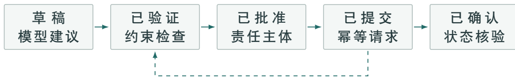
图 10.3 行动状态机的简化示意。提交失败或响应丢失后，先核验实际状态与前置条件。
