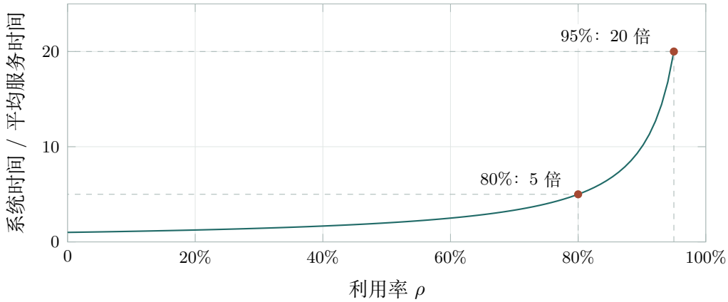
图 5.2 M/M/1 模型的平均系统时间与利用率。纵轴为等待和服务时间之和相对于平均服务时间的倍数。
