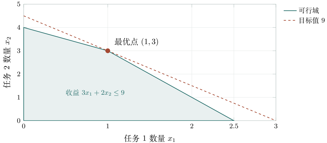
图 9.1 最优点与支持它的等目标线；资源价格提供独立的上界证明。
