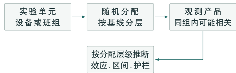
图 6.1 分配单元、观测单元与推断层级须同时声明。
