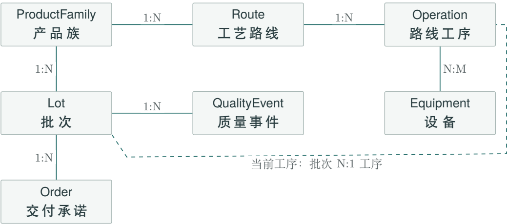
图 2.4 封测对象关系的教学抽象。虚线仅表示当前所在工序，历史流转另由事件表记录；工序与设备通过资格关系连接。
