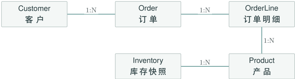
图 2.3 零售对象关系。边上的比值按正文关系读取：客户对订单、订单对明细、产品对明细及库存快照均为一对多；连线不表示事件先后。
