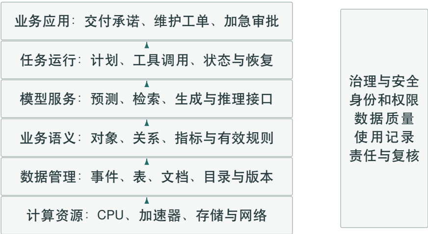
图 2.1 企业人工智能系统的六项技术职能及贯穿其间的治理要求
