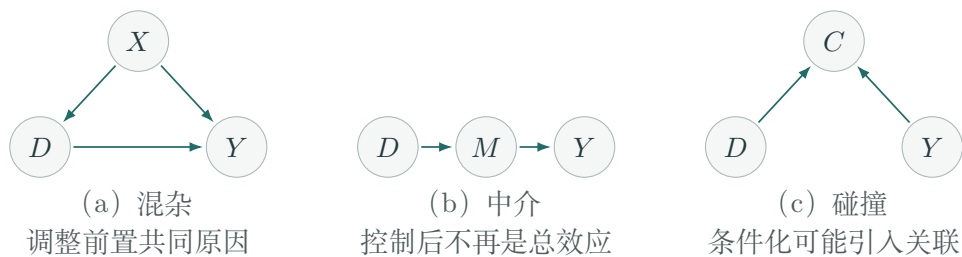
图 8.1 三个最小因果结构。图是业务机制假设，需要知识与证据支持。
