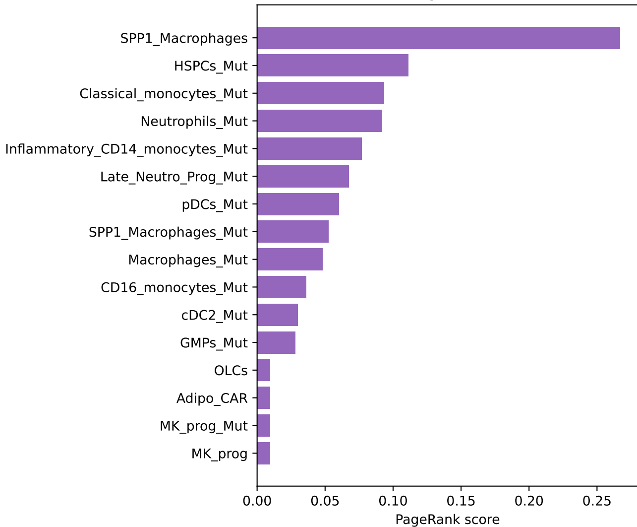
PageRank
