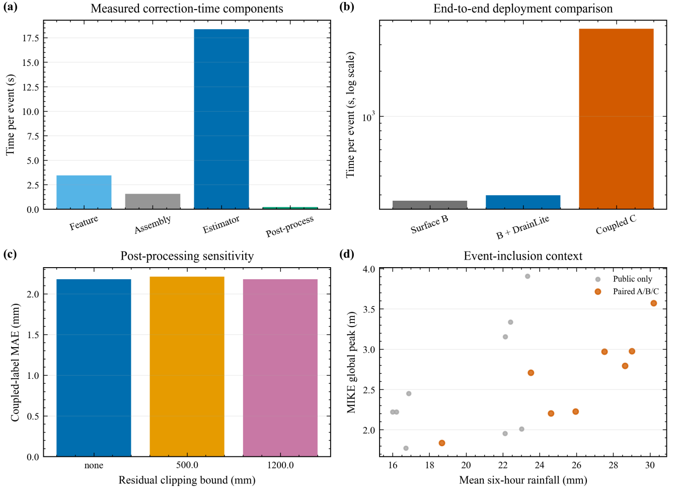
Figure 11. 运行时间、后处理敏感性和事件覆盖。
