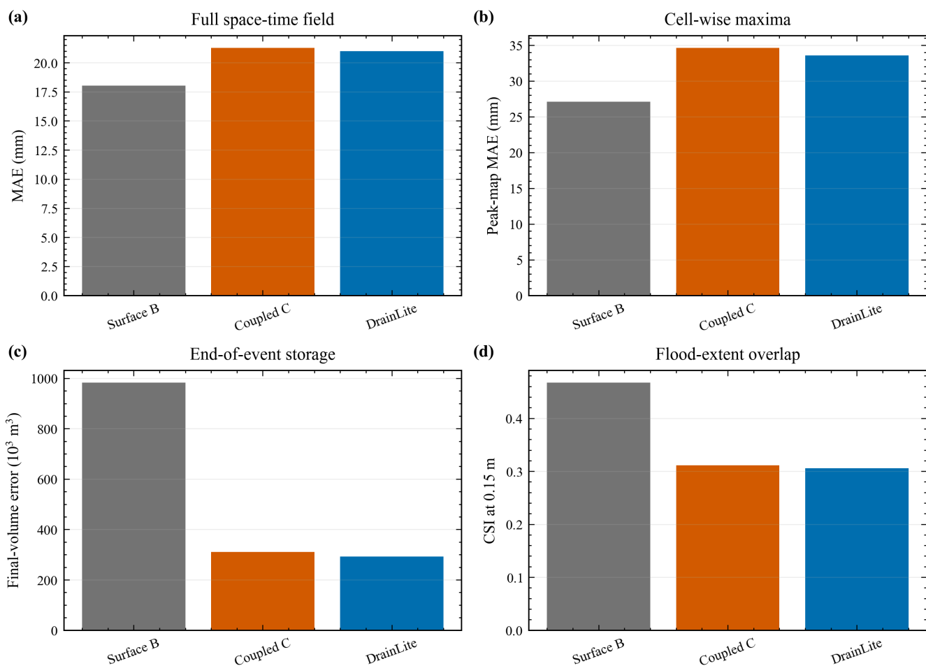
Figure 10. B、C 和 DrainLite 相对 MIKE 的四类指标。
