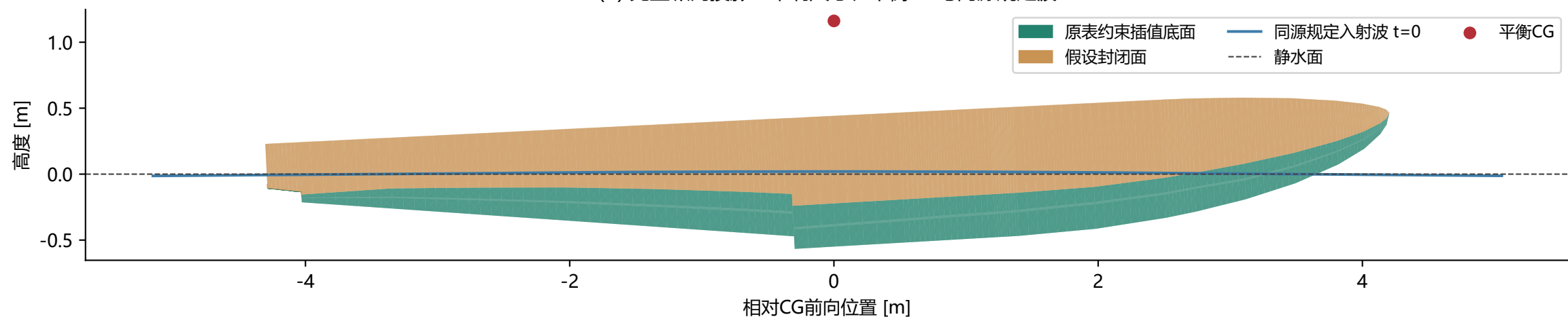
(b) 完整纵向投影: 米制尺寸、平衡CG与同源规定波
