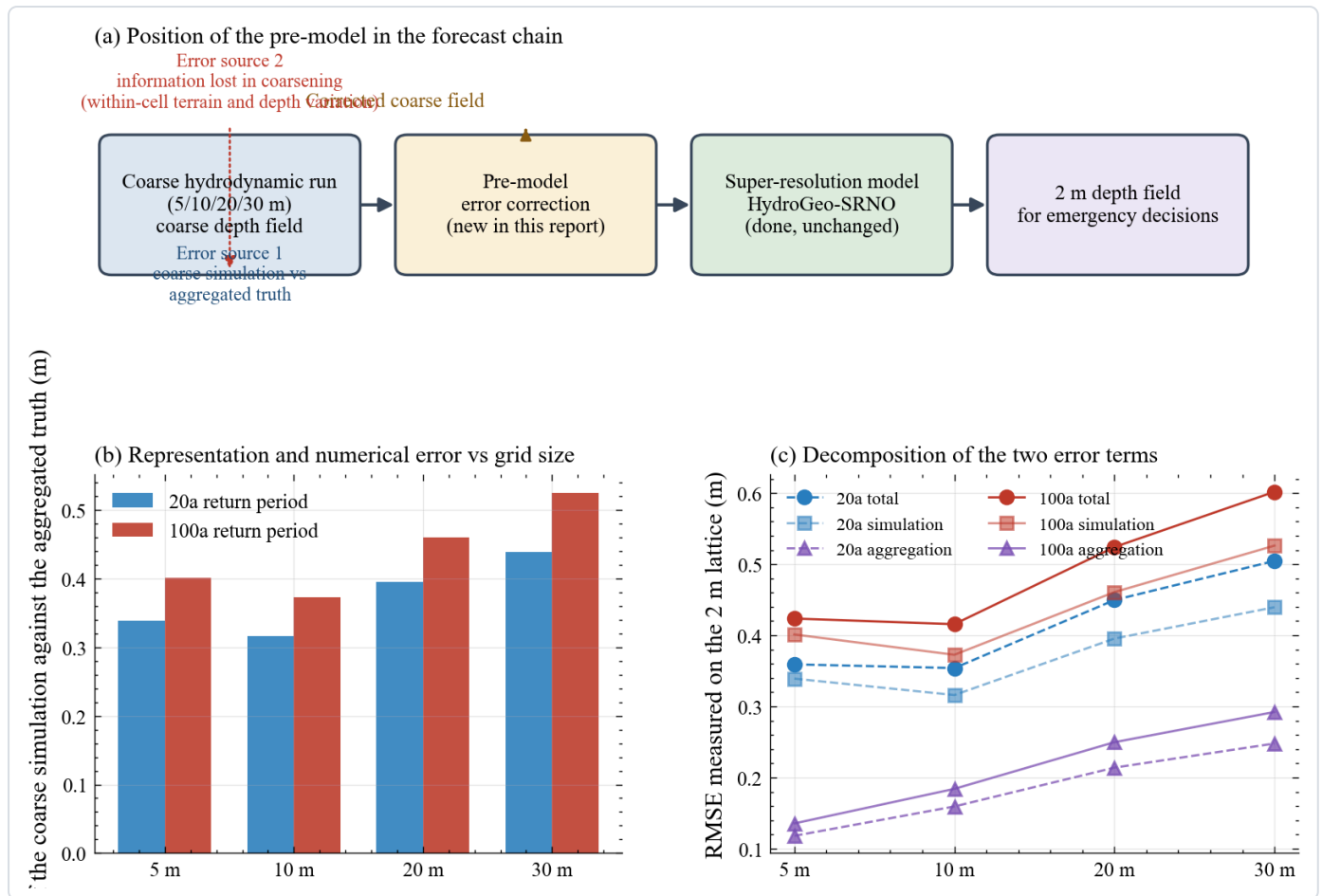
图5 前置模型在整个预报链中的位置与两类误差的量级。子图(a)是一条流程示意。第一个方框是粗网格水动力模拟，它给出边长五米到三十米的粗网格模拟水深场。第二个方框是本章新增的前置模型，它读取粗网格水深场与同一档粗网格上的静态地理特征，输出一个校正后的粗网格场。第三个方框是已经完成的超分辨率模型 HydroGeo-SRNO，本章不对它做任何改动。第四个方框是最终交付的两米水深场。方框之间的箭头表示数据流向，校正后的场同时向上反馈一条虚线，标注的是两类误差的来源。虚线来自粗化本身的信息损失，也就是单元内的地形起伏与水深变化在取平均时被抹平的那一部分。子图(b)是柱状图，横轴是四档网格边长，纵轴是粗网格模拟值相对聚合真值的均方根误差，单位是米，两种颜色对应二十年一遇与一百年一遇两个情景。柱子越高表示粗网格离聚合真值越远。可以读出两个特征，十米处的柱子最低，二十米与三十米处的柱子明显抬升，且一百年一遇情景整体高于二十年一遇。子图(c)把总误差拆成模拟项与聚合项，横轴同样是网格边长，纵轴是在两米格网上量得的均方根误差，单位是米。圆点连线是总误差，方点是模拟项，三角点是聚合项，实线对应一百年一遇，虚线对应二十年一遇。可以读出模拟项始终高于聚合项，且两者都随网格变大而上升，但聚合项上升的速度更快，说明网格越粗，信息损失在总误差里的比重越大。
