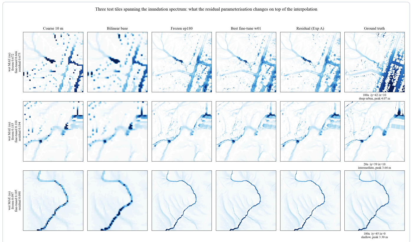
图 56 三种淹没程度瓦片的残差参数化横向对照。三行对应测试瓦片 165（深水城区）、48（中等淹没）与 229（浅水），六列依次是十米粗输入、双线性底图、冻结基线、最优微调臂、残差模型与两米真值。每行共用一套深度色标，行首给出该瓦片三个学习臂的湿区平均绝对误差，行尾给出情景、坐标、瓦片类型与真值峰值水深。每一列都覆盖了从最重的一格到最浅的一格，因此同一列上下三行的差别反映的是淹没程度，同一行左右六列的差别反映的是模型改动。读法是横向比较残差模型那一列与冻结、微调两列在同一格上的深浅起伏，判断残差参数化在哪些格上更贴近真值、在哪些格上被底图带偏。
