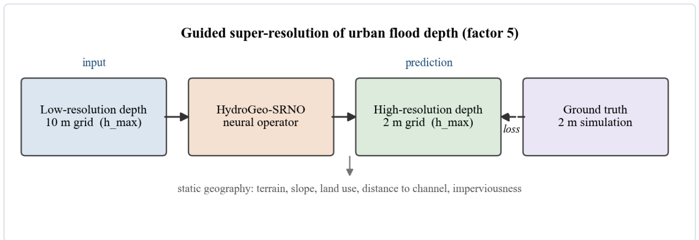
图1 引导式超分辨率任务的输入与输出。 左侧方框是模型的输入，即十米网格上的最大淹没水深场。这里说的最大淹没水深，指的是一场降雨全过程中每个位置达到过的最大水深，它比某个瞬时水深更能代表风险，因为它记录的是最不利的时刻。中间是完成映射的神经网络。右侧是模型输出的两米网格水深，训练时与独立的高分辨率模拟结果逐像素比对。下方箭头表示静态地理信息同时输入模型，它不随降雨情景变化，但对判断水往哪里流至关重要。这类结构与图像超分辨率的差别在于，低分辨率输入是一次完整的水动力求解结果，与高分辨率真值之间没有降采样关系。两者之间也就不存在确定的解析关系，因此模型无法靠套用现成的插值公式得到答案，必须真正理解地形对水流的约束。
