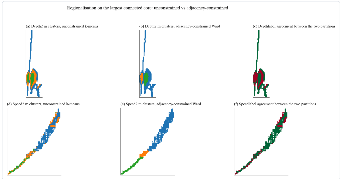
图 27 最大连通核上的区域划分对照。 上排三幅是水深，下排三幅是流速，每排的第一幅是无约束 K 均值划分，第二幅是加入上下左右邻接约束的 ward 层次聚类划分，第三幅用红绿两色标出两种划分标号是否相同，绿色表示相同。两幅划分图共用同一个簇编号色标，编号按单元的平均对数水深排序。核由湿区做一次三乘三闭运算后取最大连通分量得到，水深核有 23317 个单元，流速核有 5047 个。就本图而言，同一个二米水深场上两种划分的 V-measure 只有 0.468，说明无约束 K 均值给出的簇在空间上是碎的，加约束之后簇才连成片。
