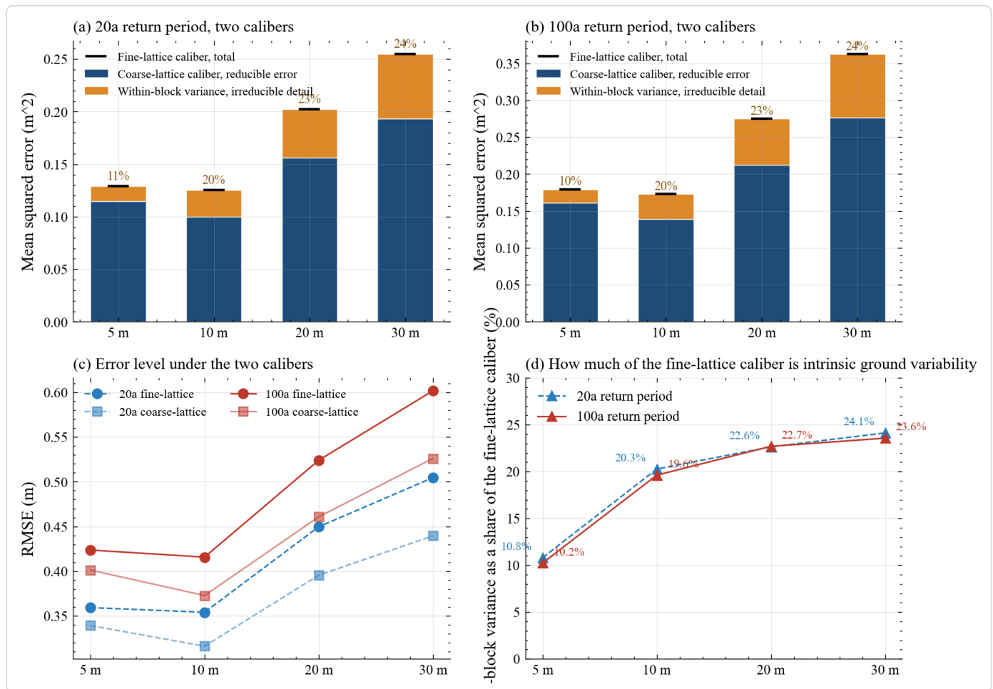
图 11 细网格口径与粗网格口径的对照。 四个子图的横轴都是四档网格边长。子图 (a) 与子图 (b) 是堆叠柱状图，分别对应二十年一遇与一百年一遇情景，纵轴是均方误差，单位是平方米。每根柱子分两段，深蓝段是粗网格口径的均方误差，橙色段是块内方差，柱顶标出的百分数是块内方差占细网格口径的比例，柱顶的黑色短横线是细网格口径的合计。可以读出两段的比例随网格变粗而改变，粗网格口径一段始终更长，块内方差一段从五米处的约百分之十升到三十米处的约四分之一，深蓝与橙色的分界随网格变粗明显上移。子图 (c) 的纵轴换成均方根误差，单位是米，实线对应一百年一遇，虚线对应二十年一遇，圆点是细网格口径，方点是粗网格口径。可以读出同一情景下细网格口径的曲线始终在上方，两条曲线的间距随网格变粗而拉大，三十米处相差百分之十四到百分之十五。子图 (d) 的纵轴是块内方差占细网格口径的比例，单位是百分数，两个情景各一条曲线，每个点旁标注具体取值。可以读出比例从五米处的约百分之十单调升到三十米处的约百分之二十四，说明网格越粗，细网格口径里属于地面本来不均匀的份额越大。需要带走的一条判断是，用细网格口径报告误差会系统性地高估模型的不足，这个间距来自地面本身的不均匀。
