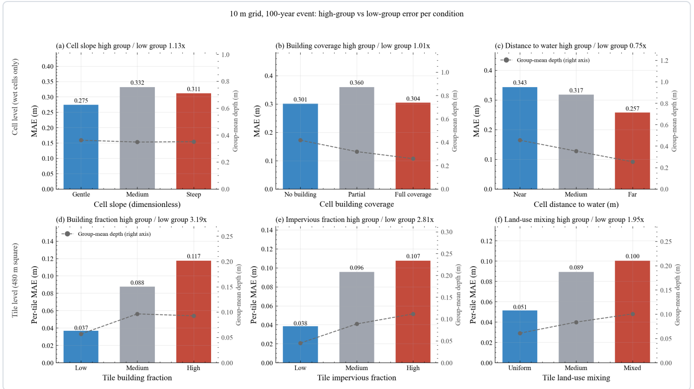
图 12 各条件取值三档之间的误差对照，十米网格。六个子图的横轴都是条件变量的三个取值档，由低到高依次为蓝色、灰色与红色三组柱子，纵轴是平均绝对误差，单位是米，柱顶数字是具体取值。每个子图还配一条灰色虚线，用右侧纵轴读数，表示该组内部的平均水深，单位是米，用来提示各组之间的水深并不相同。上排三个子图是单元一级，只统计有水单元，横轴依次是单元坡度、单元建筑覆盖率与单元到水体的距离，距离的单位是米。下排三个子图是瓦片一级，横轴依次是瓦片内建筑占比、瓦片内不透水面占比与瓦片土地利用混合度。单元建筑覆盖率的三档由二米建筑掩膜按面积加权聚合得到，覆盖率等于零为无建筑，介于零与一之间为部分覆盖，等于一为满覆盖。上排三幅的形状并不一致。坡度一幅的中间档最高，到水体距离一幅随距离单调下降，从靠近水体的 0.343 米降到远离水体的 0.257 米。建筑覆盖率一幅呈中间高两头低，部分覆盖组是 0.360 米，高于无建筑组的 0.301 米与满覆盖组的 0.305 米。下排三幅都呈明显的上升，建筑占比一幅从 0.037 米升到 0.117 米，不透水面一幅从 0.038 米升到 0.108 米，土地利用混合度一幅从 0.051 米升到 0.100 米。再看灰色虚线，上排建筑覆盖率一幅的虚线随横轴下降，说明满覆盖组的平均水深反而浅，从无建筑组的 0.417 米降到满覆盖组的 0.259 米，部分覆盖组居中的 0.320 米。既然误差的主要外部条件集中在建成状况上，校正模型就应当把建筑与地类信息当作主要输入。
