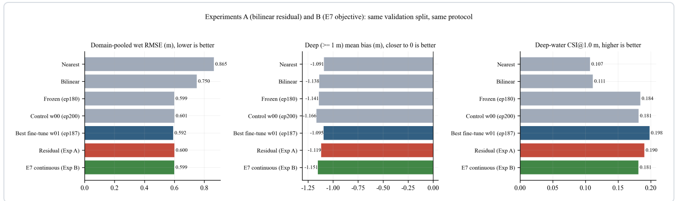
图 59 实验A与实验B在同一协议下的三项关键指标。三个子图分别是域合并湿区均方根误差、深水像元的平均有符号偏差与一米阈值下的深水判定指标。纵轴从上到下按参照类到改动类排列，红色表示残差模型，绿色表示实验B的 E7 臂，深蓝表示最优微调臂，灰色表示插值与冻结基线。三张子图的横轴量纲不同，第一张与第二张越低越好，第三张越高越好，三个子图都不能跨图比较数值。读这张图要先确定参照，也就是最优微调臂与冻结基线，再看改动臂相对它落在哪一侧。
