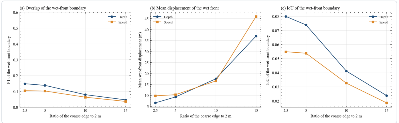
图 22 湿区前缘的重合程度。 掩膜一律由水深场给出，阈值取五厘米，水深用事件最大值，流速取峰值水量那一小时的瞬时水深。边界由形态学腐蚀得到，原掩膜减去腐蚀结果就是一圈边界像元。（a）是两圈边界的 F1，（b）是两条前缘线之间的修正豪斯多夫距离，取两个方向里较大的一个，（c）是边界交并比。水深上前缘 F1 从五米的 0.148 降到三十米的 0.046，修正豪斯多夫距离从 6.58 米升到 36.98 米。流速上前缘 F1 更低，五米是 0.104，三十米是 0.036。就本图而言，区域内部的标号一致性远高于前缘线的一致性，四对前缘 F1 最高只有 0.148。五米与十米这一对在区域内部有 0.714 的 V-measure 与 0.891 的平均交并比，边界比较里没有出现同量级的取值，分辨率的损失主要落在湿区轮廓上。
