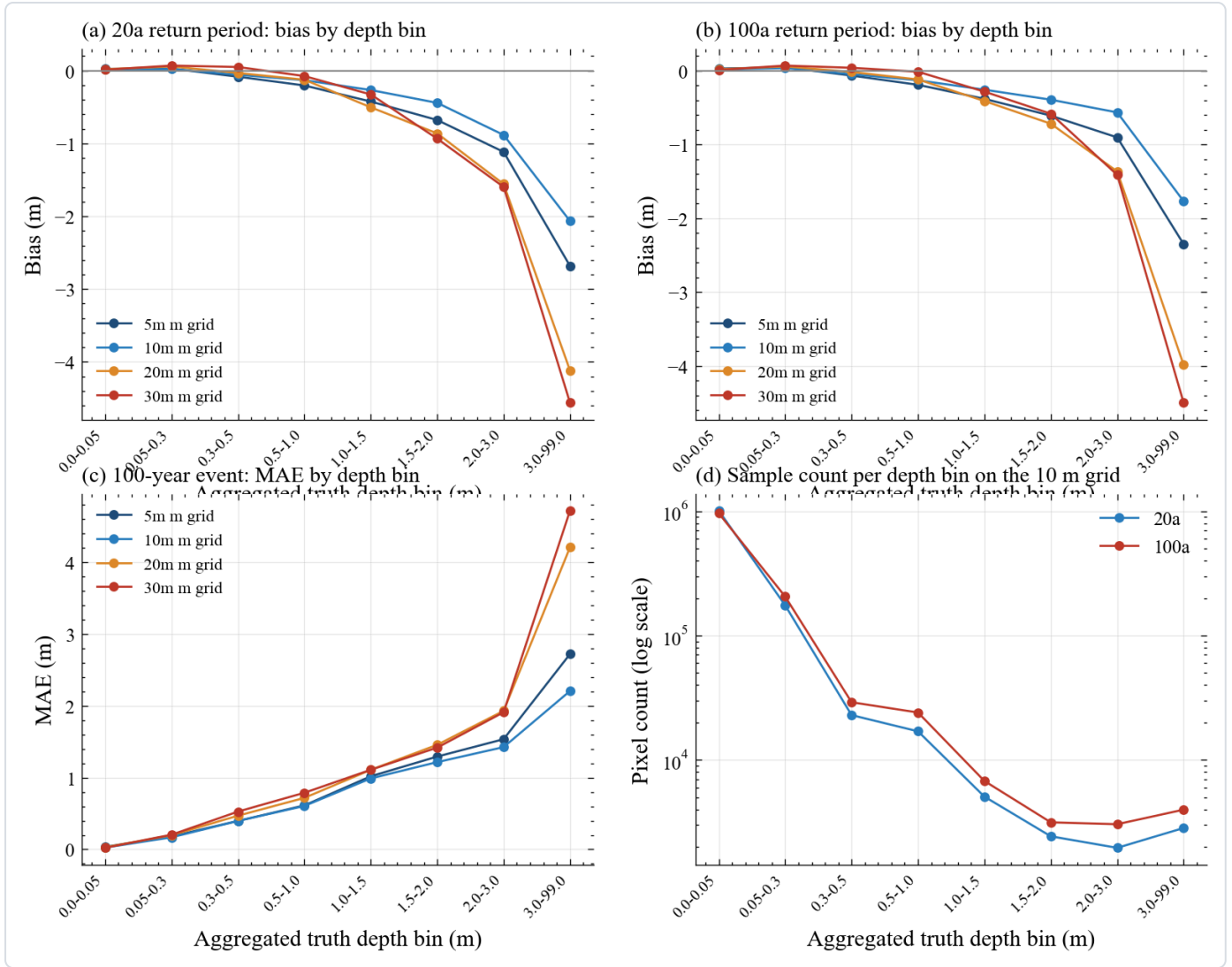
图7 按真值水深分层的误差结构。四个子图的横轴都是聚合真值水深区间，从左到右依次为0至0.05、0.05至0.3、0.3至0.5、0.5至1.0、1.0至1.5、1.5至2.0、2.0至3.0与3.0米以上。单位是米，标签旋转以便阅读。子图(a)与(b)的纵轴是平均偏差，单位是米，横线标出零，颜色对应四档网格，分别是深蓝五米、中蓝十米、橙色二十米与红色三十米，子图(a)是二十年一遇情景，子图(b)是一百年一遇情景。可以读出同一个模式。在最浅的一个区间里偏差为正，粗网格略微高估。从0.3米以上的区间开始偏差转负，此后随水深增加越来越负。在3.0米以上区间，五米网格的偏差约为负2.7米，三十米网格约为负4.6米。四条曲线在浅水区几乎重合，在深水区明显分开，说明网格尺寸的影响主要集中在深水。子图(c)的纵轴换成平均绝对误差，单位是米，只画一百年一遇情景。走势与偏差一致，最浅区间在0.04米以下，最粗的两档在深水区间超过4米。子图(d)的纵轴是单元数，用对数刻度，横轴仍为水深区间，对比两个情景。可以读出样本高度集中在浅水，十米网格的最浅区间接近一百万个单元，同一网格的最深区间不足四千个。这一点决定了深水指标的统计不确定性远大于浅水指标，后文做配对检验时必须把这件事考虑进去。
