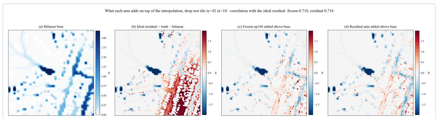
图 57 各臂在底图之上额外加载的残差场与理想残差的对照（深水瓦片 165）。(a) 是双线性底图，色标为水深；(b)(c)(d) 共用一套红蓝对称色标，(b) 是理想残差即真值减底图，(c) 是冻结基线相对底图的净增量，(d) 是残差模型相对底图的净增量。红表示在底图之上加水，蓝表示减水。图题给出两个学习臂的增量场与理想残差的相关系数。读法是先看 (b) 里深水河道应当补多少，再看 (c)(d) 是否把该补的地方补上。这一格上理想残差的深水均值是 1.069 米，而冻结与残差两臂实际在深水处净加的量分别是 0.027 与 0.004 米，两者都远小于需求，说明网络在底图之上几乎是「按兵不动」。
