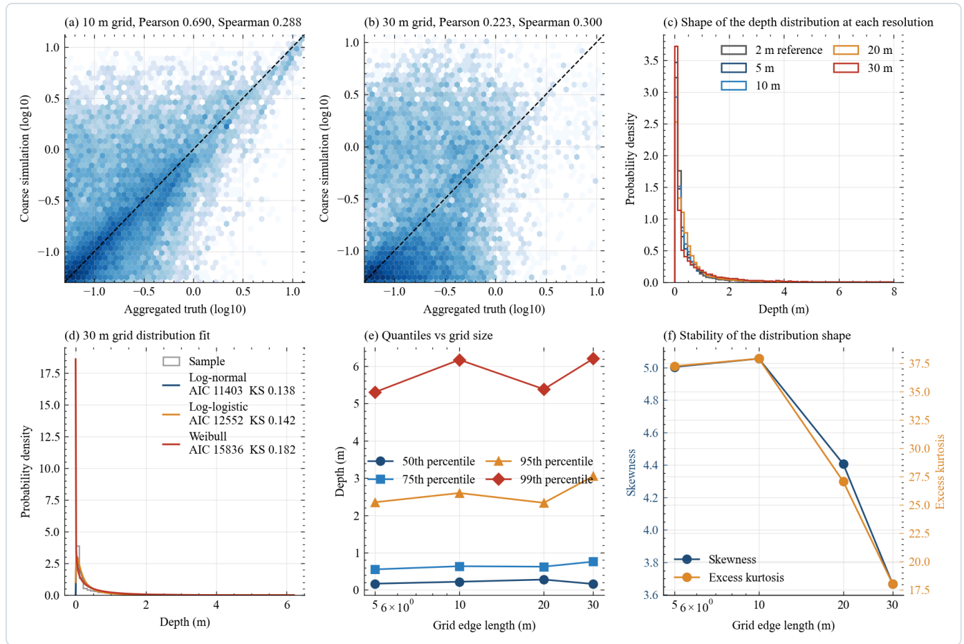
图 16 水深的跨分辨率配对与概率分布。 （a）与（b）是一百年一遇情景下十米与三十米网格的配对散点图，横轴是聚合后的二米真值，纵轴是同一单元上的粗网格模拟值，两个轴都做了十进对数变换以便看清小值区，颜色深浅表示该范围内的单元数。虚线是两者相等的等值线。点云整体沿等值线铺开，随网格变大而变宽，皮尔逊系数因此从十米的 0.690 降到三十米的 0.223。等级相关系数在四档之间保持在 0.23 到 0.30，不随网格继续恶化，但它的绝对值始终不高，说明次序信息在粗网格上也只保住了一小部分。（c）是四档网格与二米参考的水深概率密度，五条曲线都只用湿区单元，横轴截到百分之九十九点五分位。五条曲线的左端几乎重合，粗网格的曲线在中高段略微右移，差别集中在右侧尾部。（d）是三十米网格的分布拟合，灰线是样本直方图，三条彩线是赤池信息量准则最小的三个分布族，图例给出族名、AIC 与 KS 统计量。（e）是四个分位数随网格边长的变化，横轴取对数刻度，曲线整体平坦，只有百分之九十九分位在二十米之后略微抬升。（f）是偏度与超额峰度随网格的变化，两个量的量级相差很多，因此用左右两条纵轴。两条曲线都随网格下降，说明粗化把分布的尾部削轻了。
