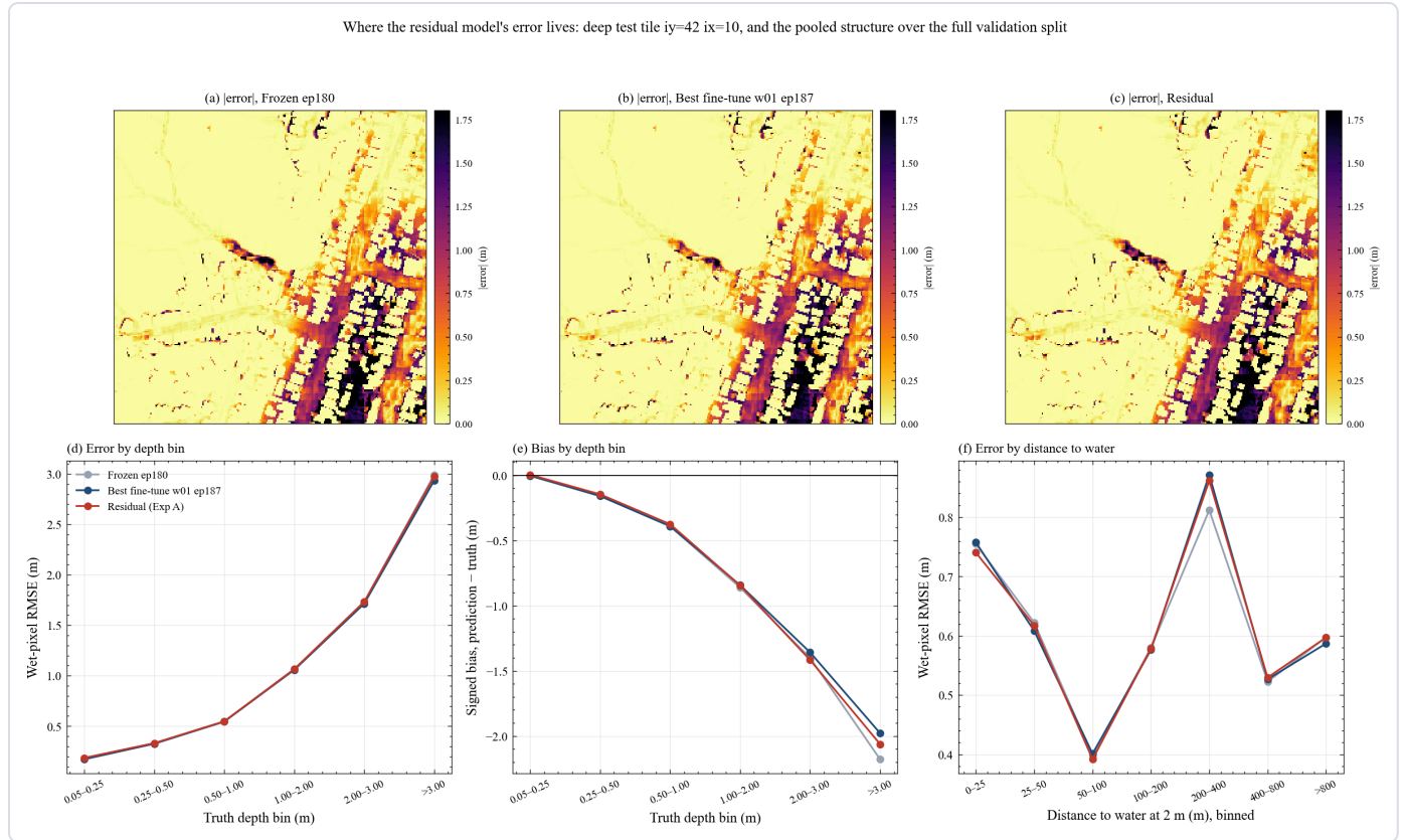
图 58 残差模型的误差空间结构（瓦片 165）与全量验证集的分箱误差。上排 (a)(b)(c) 是冻结基线、最优微调臂与残差模型在深水瓦片上的绝对误差分布，共用一套误差色标。下排 (d)(e) 是按真值水深分箱的湿区均方根误差与平均有符号偏差，(f) 是按到水体距离分箱的湿区均方根误差，三者都在全部 182 块验证瓦片上汇总，横轴分箱与第二章一致。读法是先看上排误差是否沿同一条河道成片出现，再看下排三条曲线随水深与距离的走势，判断残差模型的增益或损失是否集中在水深较大、靠近水体的那些地方。
