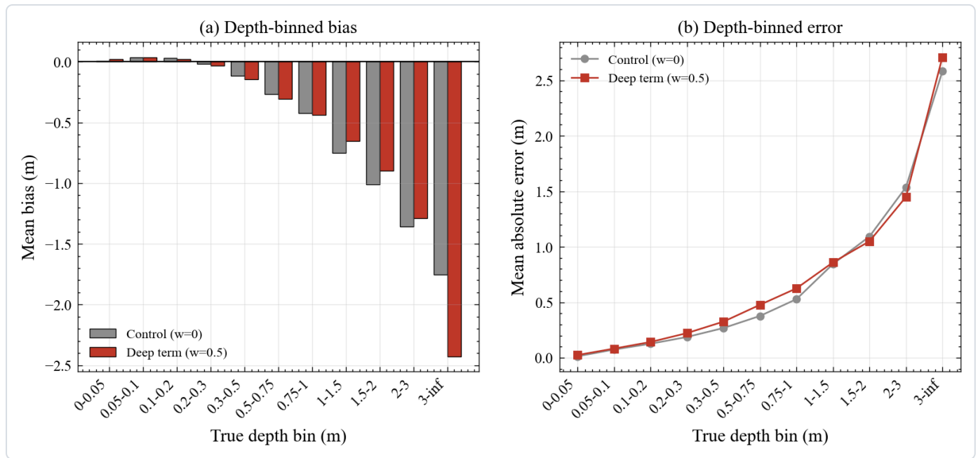
图 35 按真实水深分层的误差结构（从头训练的对照组）。这张图是把一个总体的误差数字拆成十一段来看。两个子图共享横轴，即真实水深的十一个区间，从零到 0.05 米一直延伸到三米以上，区间按深度递增排列，因此横轴从左向右代表水越来越深。左子图 (a) 是平均偏差，也就是预测值减真值的平均值，柱子向上表示高估，向下表示低估，柱子的长度就是偏差的绝对大小。右子图 (b) 是平均绝对误差，用折线表示，它先把误差取绝对值再求平均，因此只看错多少，不看错的方向。两个子图放在同一张图上，是为了把方向与幅度分开看，这是判断误差性质的基本方法。读到这里可以定，偏差与绝对误差同向上升，说明误差的主导成分是系统性低估，随机噪声只占次要位置。
