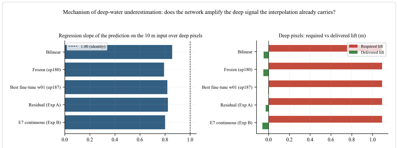
图 60 深水欠估的机制：网络是否放大了插值已携带的深水信号。左子图是深水像元上预测对十米输入的回归斜率，横轴虚线是斜率等于一，表示预测完全跟随十米输入。阶段二在被诊断的单格瓦片上量到的冻结基线与双线性是 0.39 与 0.72，本图在全量验证集上重算，因此绝对值与单格数值不同，两处只能比较相对高低，不能互相引用。右子图把深水像元相对十米输入需要的平均抬升与实际给出的平均抬升并列。斜率越接近一、实际抬升越接近需求抬升，表示模型越充分地把插值的深水信号传递到输出。
