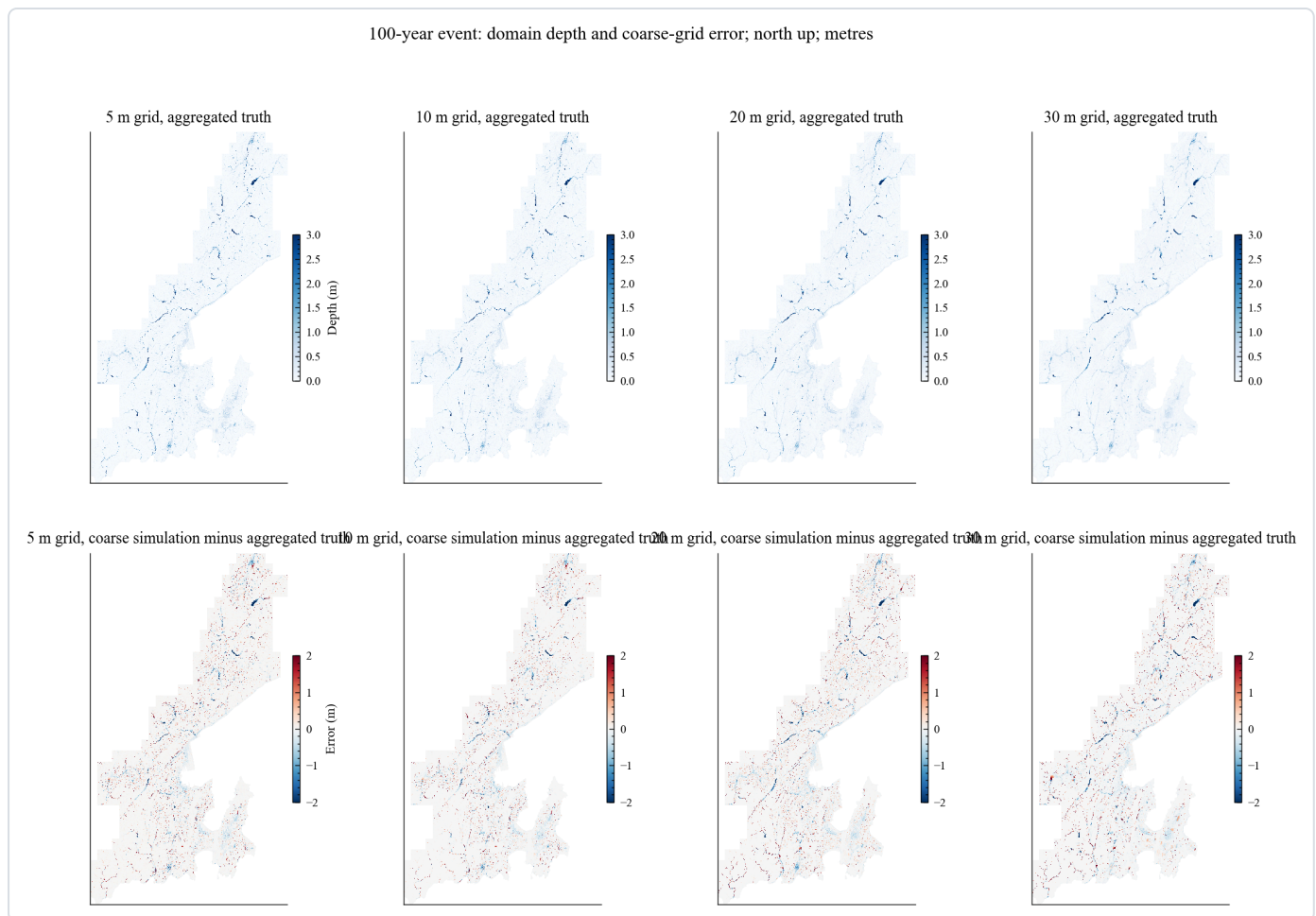
图9 一百年一遇情景下全域水深与粗网格误差的空间分布。图分上下两排，每排四幅，自左向右依次是五米、十米、二十米与三十米网格。上排是聚合后的二米真值的水深场，颜色由浅蓝到深蓝表示水深由小到大，色标范围固定在零到三米，超出三米的部分按最深色显示，每一幅配一条独立色标，单位是米。纵横坐标是格网行列号，北在上方，为了便于印刷未标注刻度数值。可以读出淹水集中在中部与南部的河谷与低洼街区，随网格变粗，同一片水域的颜色变得更均匀，细密的支流消失。下排是图4所说第三笔账的误差场，也就是粗网格模拟值减聚合真值，颜色用发散色标，红表示粗网格算深了，蓝表示算浅了，色标范围对称固定在负二米到正二米，单位是米。可以读出误差不是逐点随机的，它沿河道与地形陡变带成片出现。五米网格上的红色斑块最碎，随网格变粗逐渐连成大片，三十米网格上的蓝色条带几乎完整覆盖主要河道。把上下两排对照，可以确认蓝色条带的位置与上排的深蓝色河道位置重合，说明欠估发生在水最深的地方。
