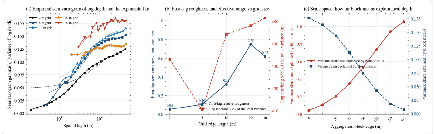
图 26 水深场的半变异函数与尺度空间。子图 (a) 是五档分辨率的对数水深实验半变异函数，横轴是空间滞后，取对数刻度，单位是米，纵轴是半方差，单位是对数水深的方差，虚线是一元指数模型的拟合曲线。子图 (b) 的左轴是首档半方差与样本总方差之比，右轴是达到总方差 95% 的滞后，单位是米，两条轴分别用蓝红两色标明。子图 (c) 把二米场按边长 4 米到 512 米的方块做面积平均再返回二米网格，左轴是块均值没有解释的方差份额，右轴是块均值自身保留的方差份额。就本图而言，三十米网格的首档相对粗糙度达到 0.618，而二米只有 0.053，达到总方差 95% 的滞后却停在 410 米到 452 米之间，块均值在 256 米上仍未解释 0.941 的局部方差。
