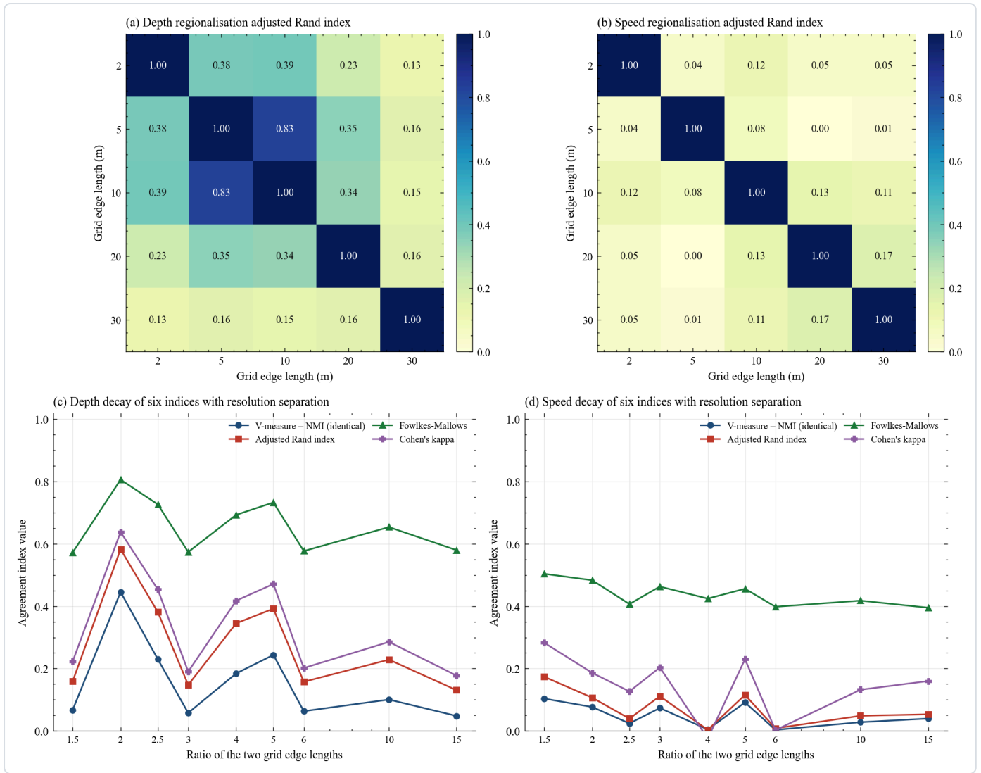
图 20 机会校正后的区域划分一致性。（a）与（b）是水深与流速的调整兰德指数矩阵，行列都是五档分辨率，对角线取一。每个矩阵里只有一个明亮的格子，水深是五米与十米这一对，取值 0.830。（c）与（d）把六类指标按两档网格的边长之比排列，横轴是对数刻度，纵轴是取值范围。信息论那条曲线是 V-measure 与归一化互信息，两者在算术归一化下恒等，图上完全重合，调整互信息与它们的差落在小数点后第五位，因此只画一条。四条曲线在排序上互相印证，水深五米与十米这一档的调整兰德指数是 0.830、Fowlkes-Mallows 是 0.922、科恩卡帕是 0.870。二米与三十米这一档只剩 0.131、0.580 与 0.178。Fowlkes-Mallows 的绝对水平最高，因为它在簇占比不均时的随机期望值就达到 0.516。就本图而言，扣除机会水平之后，二米与三十米的 Fowlkes-Mallows 只剩 0.064 的净超出，水深的区域结构只在五米与十米之间真正留存。
