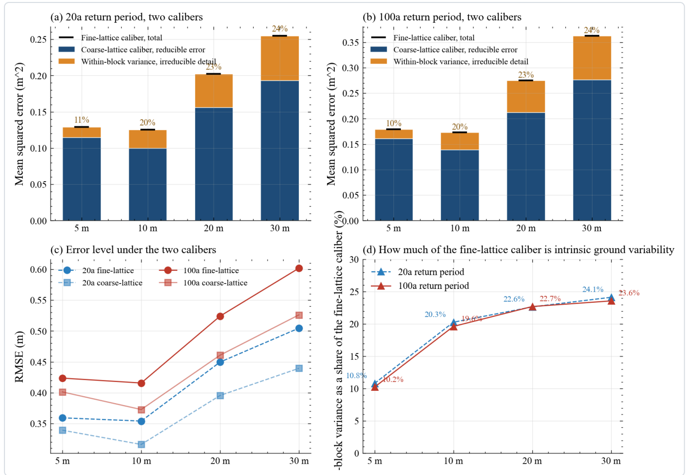
图5 细网格口径与粗网格口径的对照。子图(a)与(b)是两种口径的均方误差堆叠柱,深蓝段是粗网格口径,橙色段是块内方差。子图(c)给出两种口径的均方根误差,细网格口径的曲线始终在上方。块内方差占细网格口径的比例从五米的约10%升到三十米的约24%,两种口径在30米方格上的均方根相差14%到15%。
