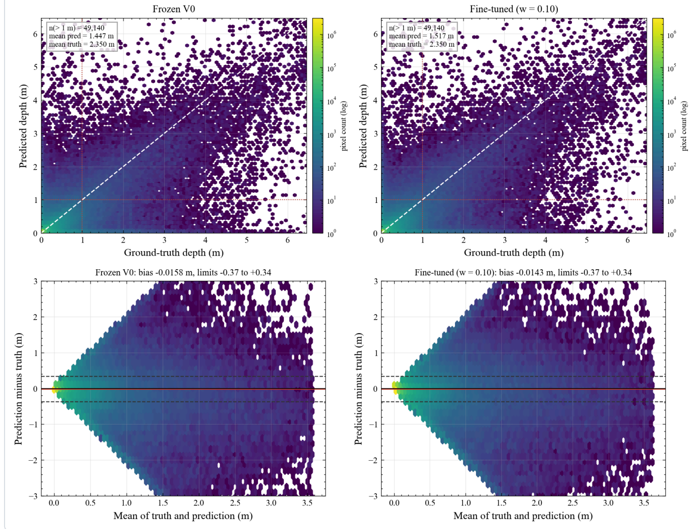
图 15 全测试集的点对点一致性。上排是预测水深与真值水深的二维密度图，白色虚线是一比一参考线，红色点线标出一米位置。下排是偏差结构图，红色实线是平均偏差，两条黑虚线是一点九六倍标准差界限。水深超过一米的像元占总像元的 1.2%，却承载全部水量的 40.4%，冻结基线在这一区间低估 84% 的像元，平均偏差负 0.903 米。
