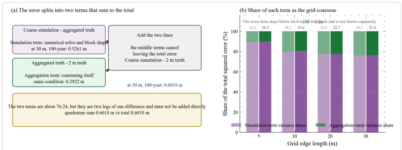
图 3 误差的三笔账与两笔账的份额。 子图 (a) 用 30 米网格、一百年一遇情景的真实数值演示加法关系。子图 (b) 把两笔账的份额画成堆叠柱状图，紫色段是模拟项，绿色段是聚合项。30 米网格上模拟项与聚合项的均方根分别是 0.5261 米与 0.2922 米，合计 0.6018 米，聚合项份额从五米的约 10% 升到三十米的约 24%。
