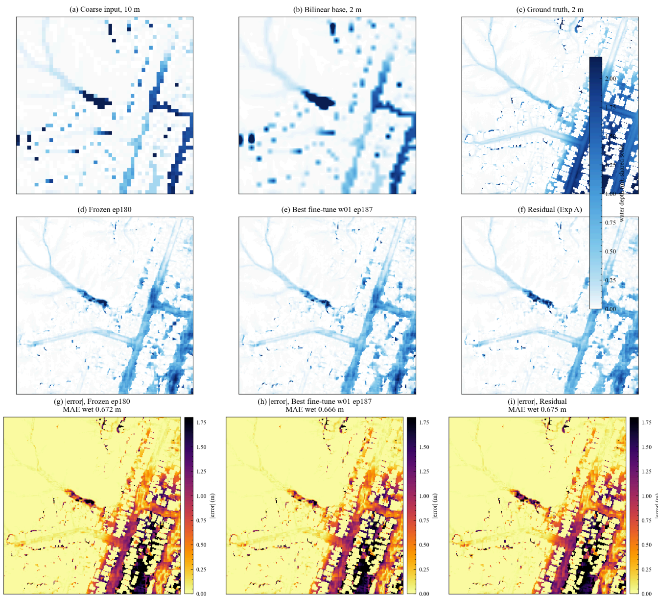
图 24 残差跨分辨率学习在深水瓦片上的逐格解剖。完整报告第六章把残差参数化提升为独立章节，给出与前几章一致的空间结果。这里只放最深一格。前两行六个面板共用一套深度色标，依次是十米粗输入、双线性底图、两米真值、冻结基线、最优微调臂与残差模型；第三行是三个学习臂相对真值的绝对误差。读法是先确定深水在哪，再看残差模型相对两个直接参数化臂是否更贴近真值。结论是残差参数化改善了深水的方向，没有改善整体量级，域合并湿区误差仍高于最优微调臂。完整的逐瓦片、误差结构与定量对比见完整报告第六章。
