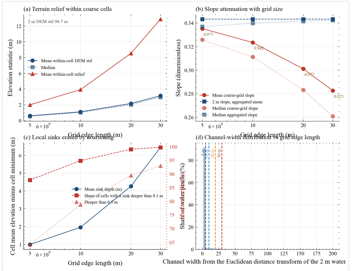
图7 地形失真随网格尺寸的变化。四个子图分别给出单元内高程统计量、坡度、洼地深度与水道宽度分布。单元内高程标准差均值从0.589米升到3.145米，单元内高差均值从1.99米升到12.87米。坡度比从0.977降到0.823，洼地深度均值从0.993米升到6.443米，洼地的丢失在20米档已基本完成。
