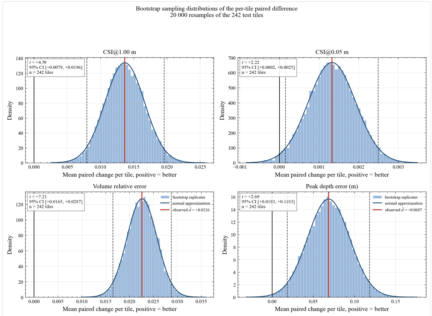
图 45 逐瓦片配对差值的自助法抽样分布。四个子图 (a) 至 (d) 分别对应深水判定指标、整体判定指标、体积相对误差与峰值深度误差。这里把配对单位换成了瓦片，也就是拿同一块地面在两个模型上的表现相比，两百四十二块测试瓦片因此给出两百四十二对数值。横轴是两个模型在这批瓦片上的平均差值，所有指标都已统一符号，正值表示微调更好，负值表示更差，这样四个子图的方向可以放在一起看。柱状图是对瓦片有放回地重新抽样两万次得到的均值分布，它刻画的是这个平均差值在换一批瓦片时会有多大波动。深色曲线是均值与标准差相同的正态分布，用来检查自助分布在有限样本下是否仍然接近正态，两者贴合说明用正态区间不会失真。黑色实线在零处，红色实线是实测均值，两条虚线夹出的范围是自助法给出的百分之九十五置信区间。各子图左上角的文本框给出统计量、置信区间与配对样本量。四个子图的小结分成两组。深水判定指标与体积相对误差的平均改善分别是正零点零一三七与零点零二二六，置信区间都不跨零，方向可靠。整体判定指标的平均改善只有零点零零一三，区间的宽度已经超过均值本身，改善存在但边缘。峰值深度误差的方向最不稳定。把四个指标放在一起，最稳的两个都落在深水与水量上，本报告的改动价值也正集中于此。
