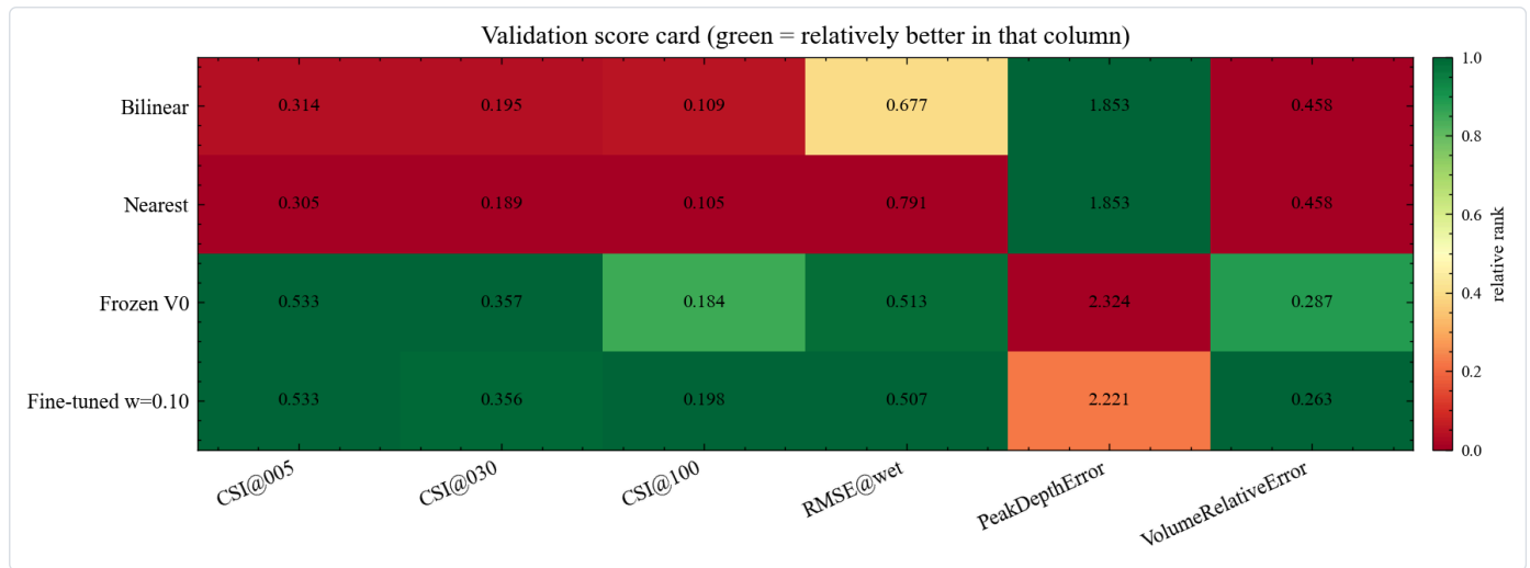
图 48 四个模型在验证集上的指标得分卡。得分卡是把多个模型在多个指标上的取值排成一张表，再用颜色标出每个模型在同一列中的相对位置。纵轴是四个模型，从上到下依次是双线性插值、最近邻插值、冻结基线与微调后模型，这样排列是为了让不做学习的方法在上、学习模型在下，便于对照。横轴是六个指标，前三列依次是 0.05 米、0.30 米与 1.00 米三档阈值下的临界成功指数，后三列依次是湿区均方根误差、峰值深度误差与体积相对误差这三个数值指标。格内数字是原始取值，读者可以直接读到具体数值，不必从颜色反推。颜色表示该模型在该列内的相对位置，绿色靠近该列最好的一端，红色靠近最差的一端。这里要特别注意颜色的比较范围只限同一列，跨列比较颜色没有意义，因为不同指标的量纲与优劣方向并不相同。按列读下来，微调模型在三档判定指标与三个数值指标上都落在绿色一端，冻结基线居中，两种插值最靠红色一端。峰值深度误差一列是例外，双线性插值在这一列反而偏绿，说明该指标单独使用时容易误导。
