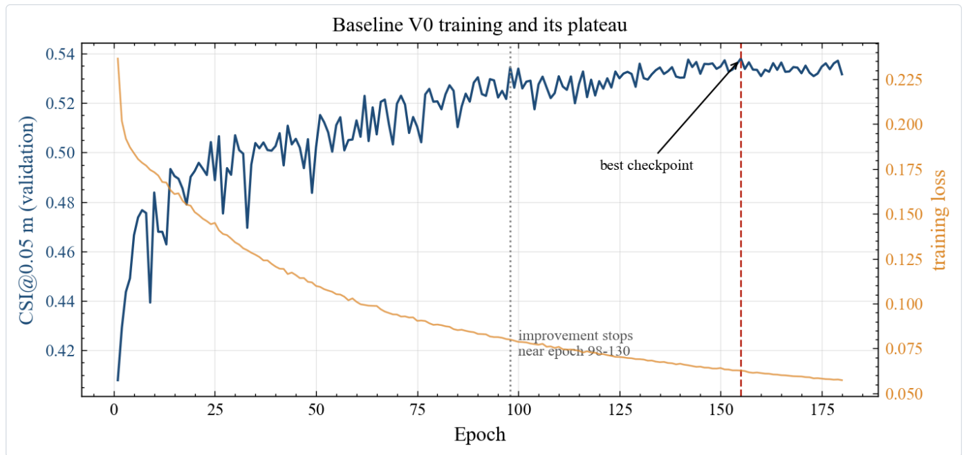
图 34 基线模型的训练曲线与饱和现象。 横轴是训练轮次，也就是模型把训练集完整看过多少遍。这张图用了左右两个纵轴，读的时候必须先确认曲线对应哪一根轴，否则会两条线的交叉误读成某种关系。左纵轴是验证集上 0.05 米阈值下的临界成功指数，蓝色实线对应此轴，看的是模型判对积水范围的能力。右纵轴是训练损失，橙色细线对应此轴，看的是模型在训练数据上的错误数值。灰色点线标在第一百轮次，红色虚线标在第一百五十五轮次，也就是验证指标最高、被选为最佳权重的那一轮。两条曲线在第一百五十五轮次前后分道，训练损失仍在缓慢下降，验证指标却停在一段很窄的区间里。此后继续训练不再提高淹没制图的质量，这一分离把问题指向损失函数与评价指标之间的偏差。
