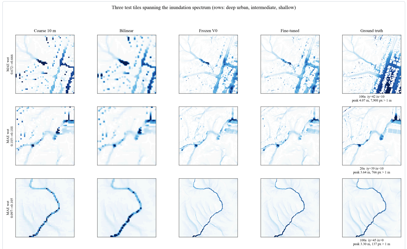
图 41 三个瓦片跨越淹没程度区间的对比。这张图的用意是检验改善是否与积水程度有关。三行按积水程度由深到浅排列，由上到下分别是深水城市瓦片、中等淹没瓦片与浅水瓦片，这样排列便于纵向追寻同一列在图上的变化。每一行从左到右依次是十米粗输入、双线性插值、冻结基线预测、微调后预测以及两米真值。读法是先看最右一列的真值，记住该瓦片的实际水深格局，再回到左边看各方法重建得如何。十米输入与双线性插值两列的作用是给出不做学习的下限，用于判断模型是否真的学到了结构。每一行单独设定色标量程，因此在同一行内比较颜色是有效的，跨行比较颜色深浅则没有意义，这一点与得分卡的限制相同。行首标注该瓦片的湿区平均绝对误差在冻结与微调两个模型下的数值，读者可以直接读出这一格的误差变化，不必从颜色估算。三行放在一起指向同一条结论，改善与积水程度没有简单的对应。深水判定指标在第二行与第三行上都上升，而这两行的深水像元数分别是七百六十六与一百三十七，都远小于第一行，说明改善既不依赖瓦片的水量，也不依赖某一类特定的积水格局。平均绝对误差与峰值深度误差则涨落不一，后者在十万像素里只由最深的一个决定。
