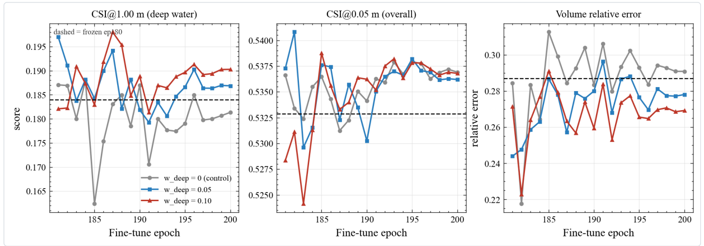
图 44 三个微调实验臂在全验证集上的逐轮表现。三个子图共享横轴，即微调轮次，从第一百八十一轮到第二百零轮，共二十个点，每点是一次全量评估的结果。左子图 (a) 是深水指标，也就是一米阈值下的临界成功指数。中子图 (b) 是整体指标，也就是五厘米阈值下的临界成功指数。右子图 (c) 是体积相对误差，衡量全图总水量的相对偏差，数值越小越好。三个子图中，灰色圆点是权重为零的对照臂，蓝色方块是权重 0.05 的实验臂，红色三角是权重 0.10 的实验臂。两条虚线是冻结基线在对应指标上的水平，作为参考，用来判断微调之后的模型相对微调之前处在什么位置。读这张图的方法是先看同一条线自己的走势，判断训练是否稳定。再在同一个轮次上比较三条线，判断深水项是否带来层次。最后看三个子图的层次是否一致，判断改善与代价的关系。三个子图给出的阶段性结论是深水项确实建立了层次，深水指标随权重升高而抬升，整体指标与体积误差的代价却被压在很小的幅度内，两个成功的权重都没有让整体精度明显退化。
