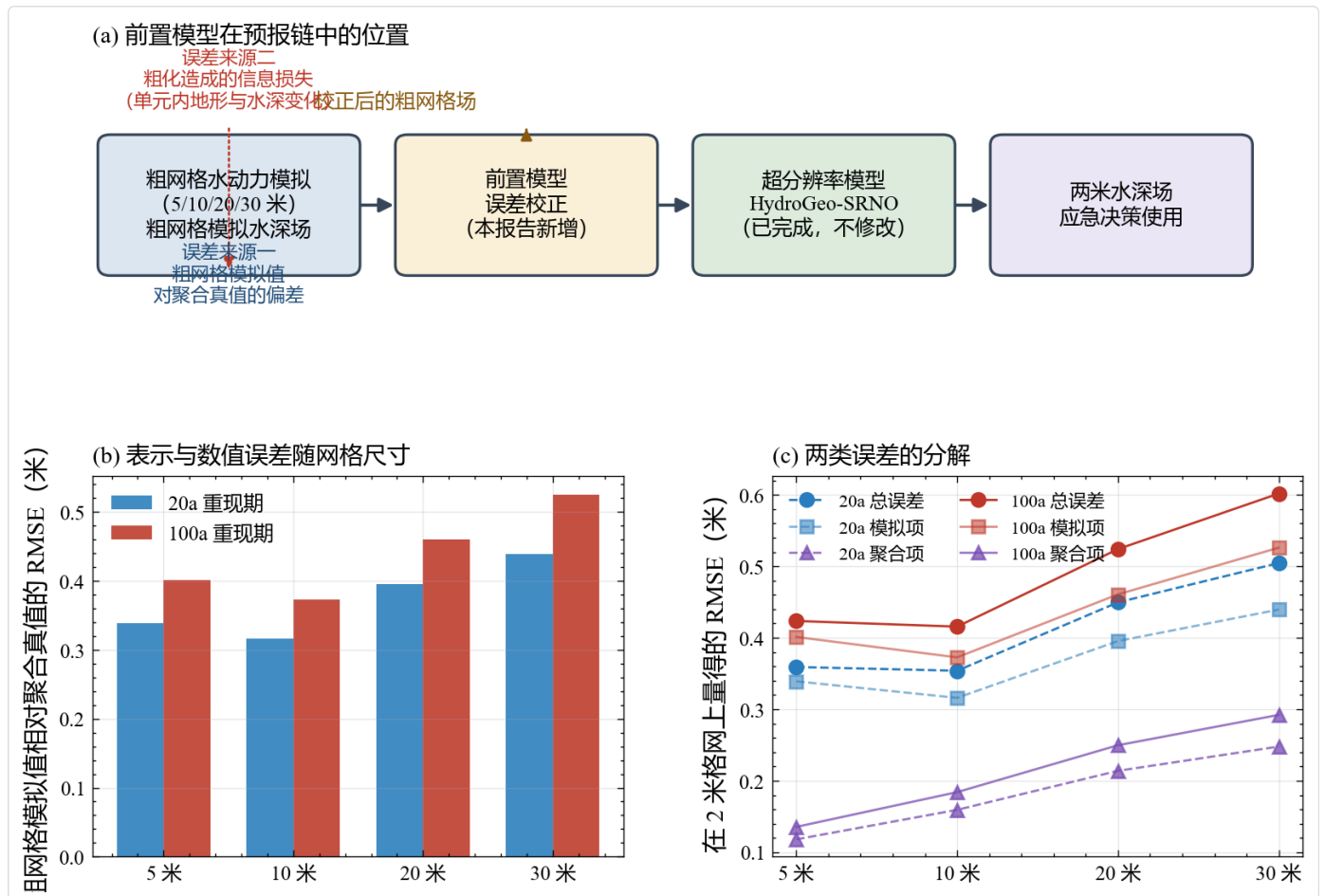
图5 前置模型在整个预报链中的位置与两类误差的量级。子图(a)是一条流程示意。第一个方框是粗网格水力模拟,它给出边长五米到三十米的粗网格模拟水深场。第二个方框是本章新增的前置模型,它读取粗网格水深场与同一档粗网格上的静态地理特征,输出一个校正后的粗网格场。第三个方框是已经完成的超分辨率模型 HydroGeo-SRNO,本章不对它做任何改动。第四个方框是最终交付的两米水深场。方框之间的箭头表示数据流向,校正后的场同时向上反馈一条虚线,标注的是两类误差的来源。虚线来自粗化本身的信息损失,也就是单元内地形起伏与水深变化在取平均时被抹平的那一部分。子图(b)是柱状图,横轴是四档网格边长,纵轴是粗网格模拟值相对聚合真值的均方根误差,单位是米,两种颜色对应二十年一遇与一百年一遇两个情景。柱子越高表示粗网格离聚合真值越远。可以读出两个特征,十米处的柱子最低,二十米与三十米处的柱子明显抬升,且一百年一遇情景整体高于二十年一遇。子图(c)把总误差拆成模拟项与聚合项,横轴同样是网格边长,纵轴是在两米格网上量得的均方根误差,单位是米。圆点连线是总误差,方点是模拟项,三角点是聚合项,实线对应一百年一遇,虚线对应二十年一遇。可以读出模拟项始终高于聚合项,且两者都随网格变大而上升,但聚合项上升的速度更快,说明网格越粗,信息损失在总误差里的比重越大。
