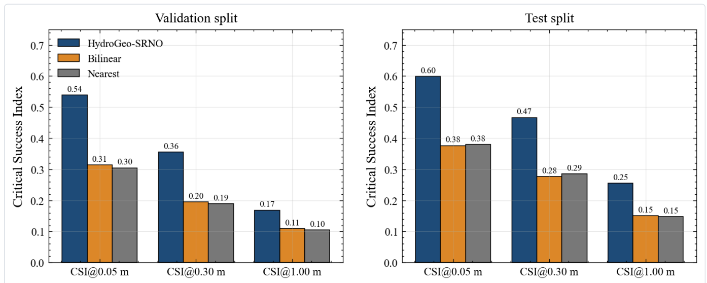
图 43 模型与两种传统插值方法的指标对比。左子图 (a) 是验证集，右子图 (b) 是测试集，两个子图的结构完全一致，可以左右对照着读。每组内三根柱子依次是模型、双线性插值与最近邻插值，柱子的颜色区分方法。纵轴是临界成功指数，取值在零到一之间，越高越好。横轴是三档判定阈值，从左到右依次升高，阈值越高表示判定积水的门槛越严。柱顶数字是具体取值。这张图的作用是给出一个背景基线，回答学习模型相比不做学习的插值方法到底好多少，好在哪个阈值上，以及这个优势是否在不同数据集上稳定。三档阈值上模型的柱子都高于两种插值，验证集与测试集给出的次序完全一致，说明学习模型相对几何插值的优势在独立数据上可以复现。
