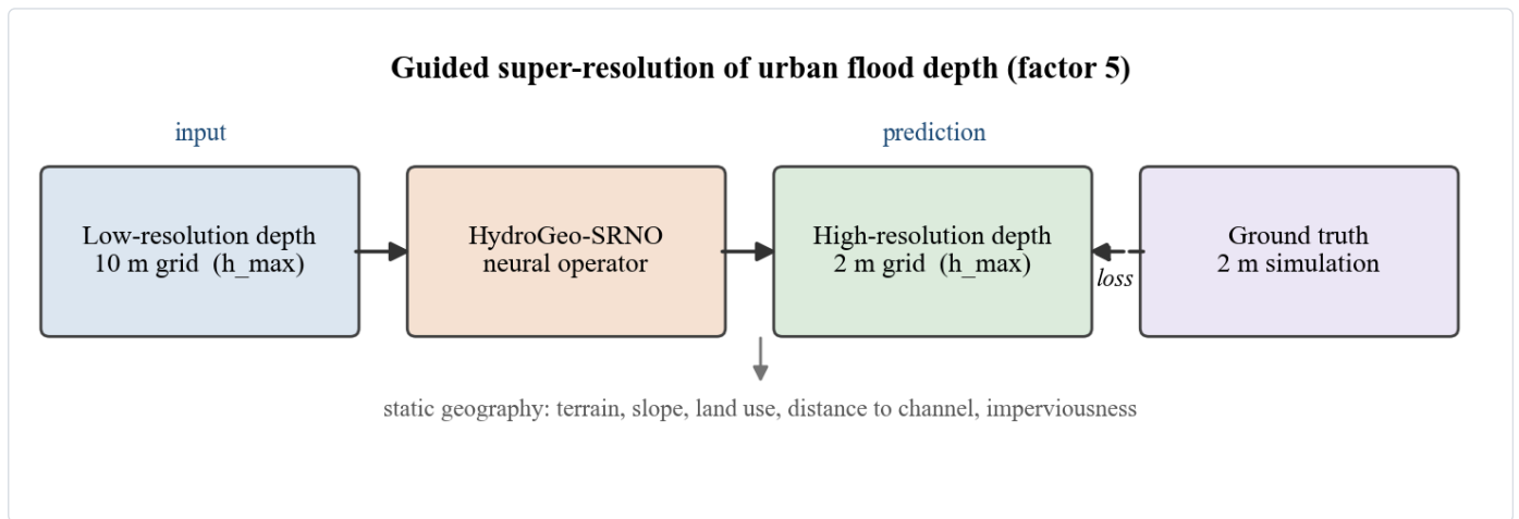
图1 引导式超分辨率任务的输入与输出。左侧方框是模型的输入，即十米网格上的最大淹没水深场。这里说的最大淹没水深，指的是一场降雨全过程中每个位置达到过的最大水深，它比某个瞬时水深更能代表风险，因为它记录的是最不利的时刻。中间是完成映射的神经网络。右侧是模型输出的两米网格水深，训练时与独立的高分辨率模拟结果逐像素比对。下方箭头表示静态地理信息同时输入模型，它不随降雨情景变化，但对判断水往哪里流至关重要。这类结构与图像超分辨率的差别在于，低分辨率输入是一次完整的水动力求解结果，与高分辨率真值之间没有降采样关系。两者之间也就不存在确定的解析关系，因此模型无法靠套用现成的插值公式得到答案，必须真正理解地形对水流的约束。
