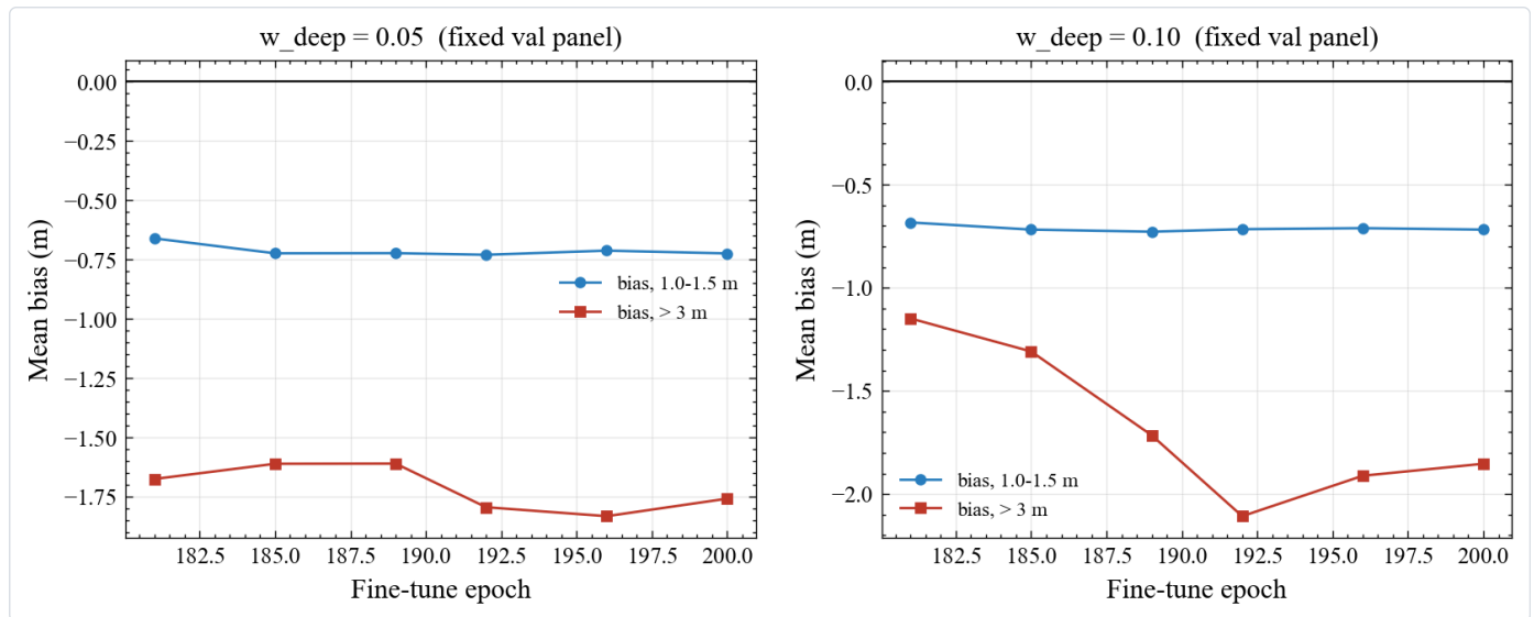
图 52 深水偏差随微调轮次的变化（固定验证瓦片）。左右两个子图分别是权重 0.05 与 0.10 的实验臂，两个子图的结构完全一致，可以左右对照。横轴是微调轮次，从第一百八十一轮到第二百零轮。纵轴是平均偏差，单位为米，零线表示无偏差，曲线落在零线以下代表低估，越低表示低估越严重。蓝线是水深一至一点五米区间，红线是三米以上区间，两个区间分别代表深水的入口与最深处。这张图的作用是把最终指标拆回到训练过程中，回答改善是在什么时候、以什么方式出现的。固定面板上的读数给出一个必须报告的负面信息。三米以上区间的偏差在权重 0.10 下没有改善，反而从负 1.15 恶化到负 1.85 附近。微调让最深区域整体上更接近真值，却没有解决它系统性偏浅的方向问题，这两件事必须分开表述。
