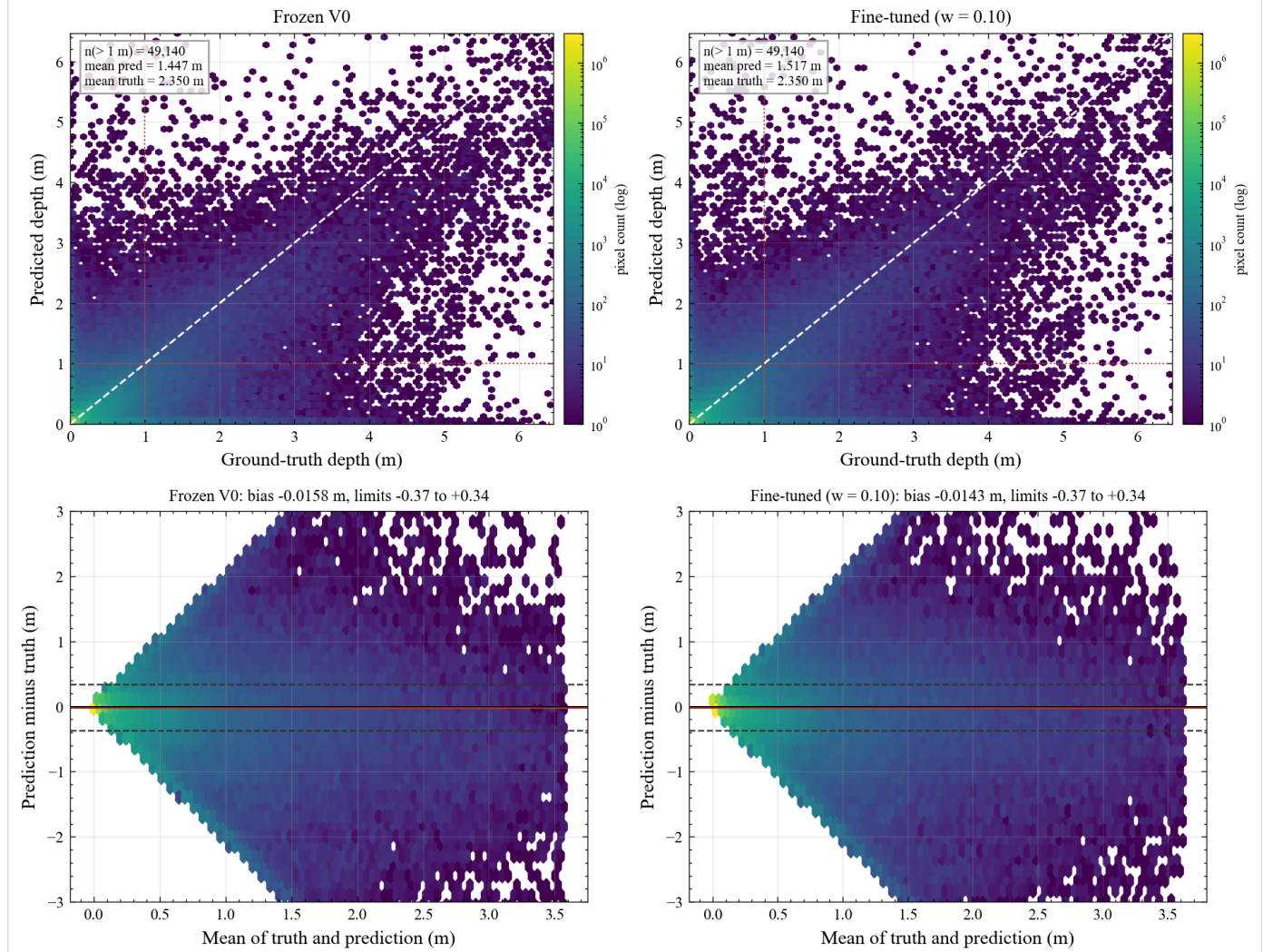
图 42 全测试集的点点对一致性。 这张图回答的是预测与真值在数值上对不对得上。上排是预测水深与真值水深的二维密度图，横轴是真值，纵轴是预测，颜色深浅表示落在该处的像元数，采用对数标度以便同时显示密集区与稀疏区。白色虚线是一比一参考线，点落在这条线上表示预测与真值相等，落在下方表示预测偏浅。红色点线标出一米位置，用来圈定深水区段。左下角文本框给出深水像元个数以及该区间上预测与真值的均值，可以直接读出偏差的量级。下排是偏差结构图，横轴是预测与真值的平均，纵轴是预测减真值，这类图用来判断偏差是否随水深变化。红色实线是平均偏差，两条黑色虚线是一点九六倍标准差给出的界限，黑色实线在零处。读法是先在上排看密度带相对对角线的位置，再在下排看漏斗是否张开。本图要留给读者的一句判断是，深水在像元数是少数、在水量上是多数。水深超过一米的像元只占总像元的百分之一二，却承载了全部水量的百分之四十点四，因此以像元平均为基础的指标被浅水区主导，深水的偏差在平均时被稀释。
