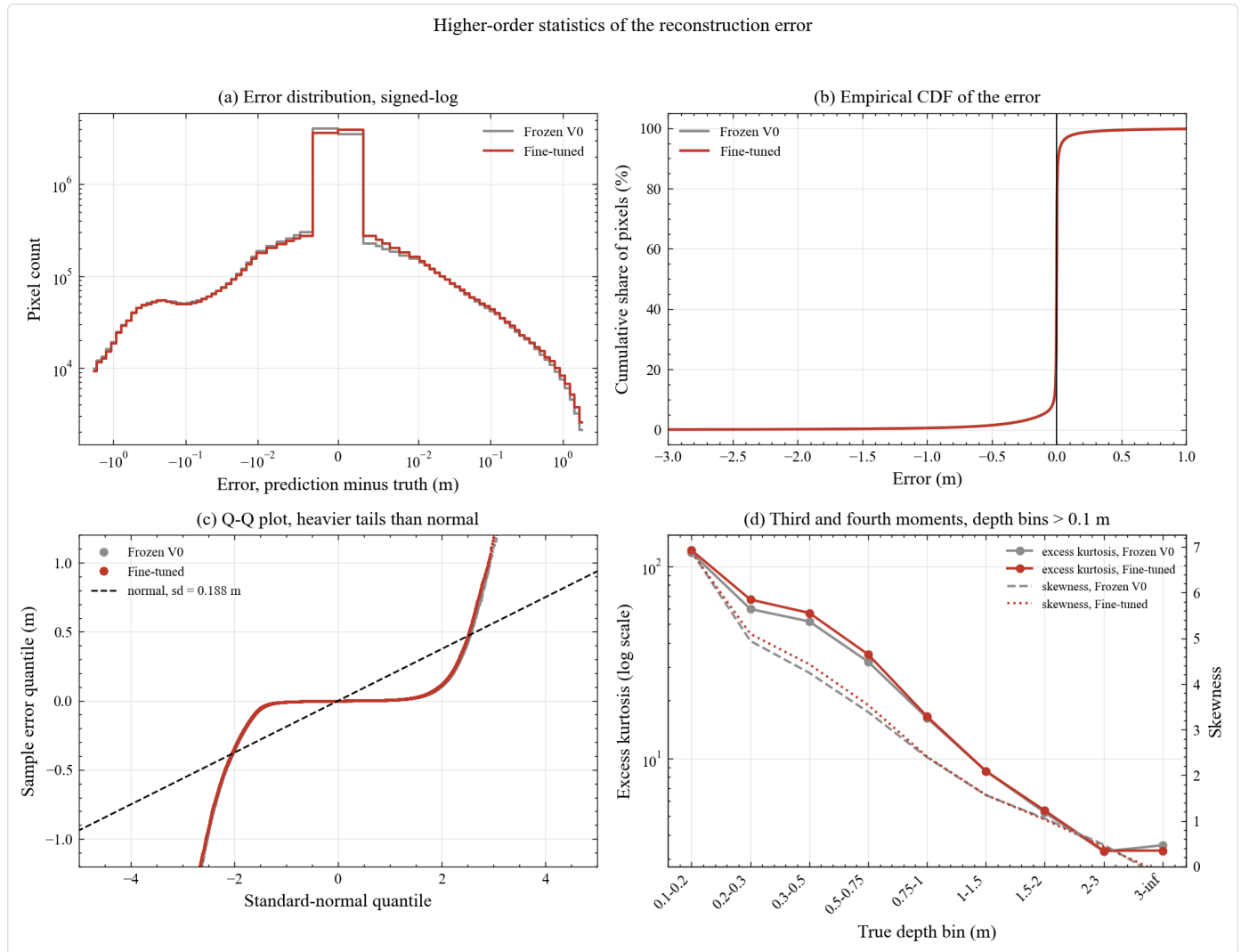
图 49 重构误差的分布与高阶矩。 这一组子图把误差当成一个分布来考察，关注的是它的形状而不只是平均值。(a) 是两个模型误差的频次分布，横轴采用对称对数标度以便同时展示零附近的密集区与两侧的长尾，纵轴为对数标度。(b) 是误差的经验累积分布，横轴是误差取值，纵轴表示误差不超过给定值的像素占比，曲线越陡说明误差越集中，曲线在某一侧拖长说明该侧出现大误差的机会更多。(c) 是分位数对分位数图。它的做法是把实测误差与一个标准差相同的正态分布按同样的累积概率逐点配对，如果误差服从正态分布，所有点就会落在黑色虚线上，散点偏离该线越远说明尾部越重。(d) 是分水深区间的偏度与超额峰度，峰度用对数纵轴，偏度用右侧纵轴，最浅的两个区间因为真值接近零、分布退化，未纳入该子图。读的顺序是先看 (a) 判断整体形状，再看 (b) 定位大误差出现在哪一侧，然后用 (c) 检验尾部是否偏离正态，最后用 (d) 看不同水深上的形状差异。四幅子图给出的阶段性结论是误差分布接近拉普拉斯形状，左尾很厚。两个模型的分布曲线几乎完全重合，说明微调没有改变误差的总体形状，只挪动了少量质量。用正态假设去推断深水误差的置信区间会严重低估风险。
