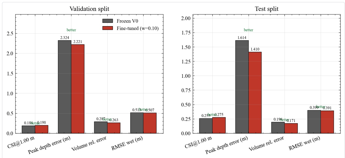
图 47 冻结基线与微调模型的逐项对比。这张图的用意是把改动前后放在一起，让读者一眼看清哪几项动了、哪几项没动。左子图 (a) 是验证集，右子图 (b) 是测试集，两个子图的结构完全一致，可以左右对照。每组内左柱是冻结基线，也就是微调之前的模型，右柱是微调之后的模型。四个指标依次是深水指标、峰值深度误差、体积相对误差与湿区均方根误差。读这张图要先分清方向，深水指标越大越好，后三项越小越好，因此后三项的柱高降低才代表改善。柱间的文字标出该项是变好还是变差，不确定方向时可以依赖这个标注。两个子图都给出是为了确认改善能在独立区域上复现，这一点在第 5.9 节有专门讨论。四组柱子读下来的结论只有一句，改善集中在与深水直接相关的三项上。深水指标从 0.184 升到 0.198，峰值深度误差从 2.32 米降到 2.22 米，体积误差从 0.287 降到 0.263，测试集上的降幅比验证集更大，说明修正具有普遍性，不是对验证集地理特点的适配。
