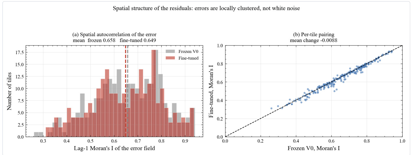
图 50 误差场的空间自相关。 空间自相关衡量的是相邻位置上的数值是否倾向于同向，它是判断误差属于随机噪声还是成片结构的关键工具。(a)是逐瓦片 lag-1 空间自相关指标的分布。lag-1 表示只比较一个像元与它紧邻像元的关系，不涉及更远的距离。横轴是指标取值，纵轴是落在该取值的瓦片个数，两条曲线分别对应冻结基线与微调模型。(b)是同一瓦片在两个模型下的配对散点，横轴是冻结基线的指标取值，纵轴是微调模型的取值，对角虚线是两者相等的参考线，点落在虚线下方说明微调之后自相关下降。指标采用莫兰指数，定义在有效像元上、使用四邻域权重，取值接近一时表示相邻像元的误差高度同向，接近零时表示误差在空间上随机，为负则表示相邻像元误差反向。所有瓦片的有效像元数相同，因此不同瓦片之间可以直接比较。本图要给出的一条判断是，重构误差在空间上高度成片，并非逐点独立的噪声。两个模型的指数都集中在零点五到零点七之间，二百四十二个瓦片中有两百零五个的冻结基线指数超过零点五。微调模型的自相关平均下降零点零零八八，配对统计量为负六点一八，说明下降是系统性的，误差被摊得更均匀，但成片程度并没有根本改变。
