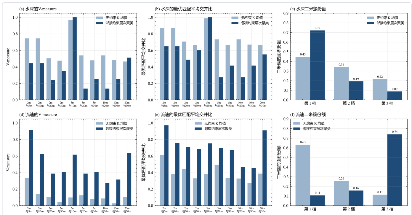
图 28 连通核上的无约束与邻接约束划分对比。上排是水深，下排是流速。左列是十个分辨率组合的 V-measure，中列是最优匹配平均交并比，两列的横轴都是分辨率组合，蓝色柱为无约束，深蓝色柱为邻接约束。右列是二米划分三个簇的面积份额，横轴是簇编号，两组柱并列。就本图而言，水深处五米与十米的 V-measure 由 0.969 升到 1.000，十米与二十米由 0.538 降到 0.137。流速上五米与十米由 0.098 升到 0.617，约束把水深最大一簇的份额从 0.446 抬到 0.721。
