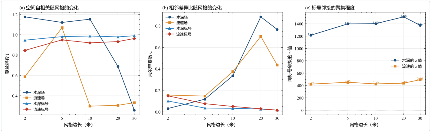
图 23 水深场与标号的空间自相关。权重矩阵在二米湿区上按上下左右四邻构造，取二值权重且不按行标准化，莫兰指数的上界因此高于一，它的零期望值是负的 1/(n-1) ，本图样本上约等于零。（a）是莫兰指数，（b）是吉尔里系数，两条曲线都按网格边长排列，横轴取对数刻度。（c）是同标号邻接的计数检验，纵轴是置换检验的 z 值，柱标给出观测值与期望值之比。水深场的莫兰指数从二米的 1.175 降到三十米的 0.257，吉尔里系数从 0.030 升到 0.767。同一批数据上的标号莫兰指数五档全在 0.946 到 0.989 之间，同标号邻接比值从 1.61 升到 2.16，置换检验的 z 值都在 1200 以上。就本图而言，三十米水深场的莫兰指数只剩 0.257，而标号莫兰指数还有 0.989，说明落差来自每一片边界位置的移动，而非成片程度的下降。
