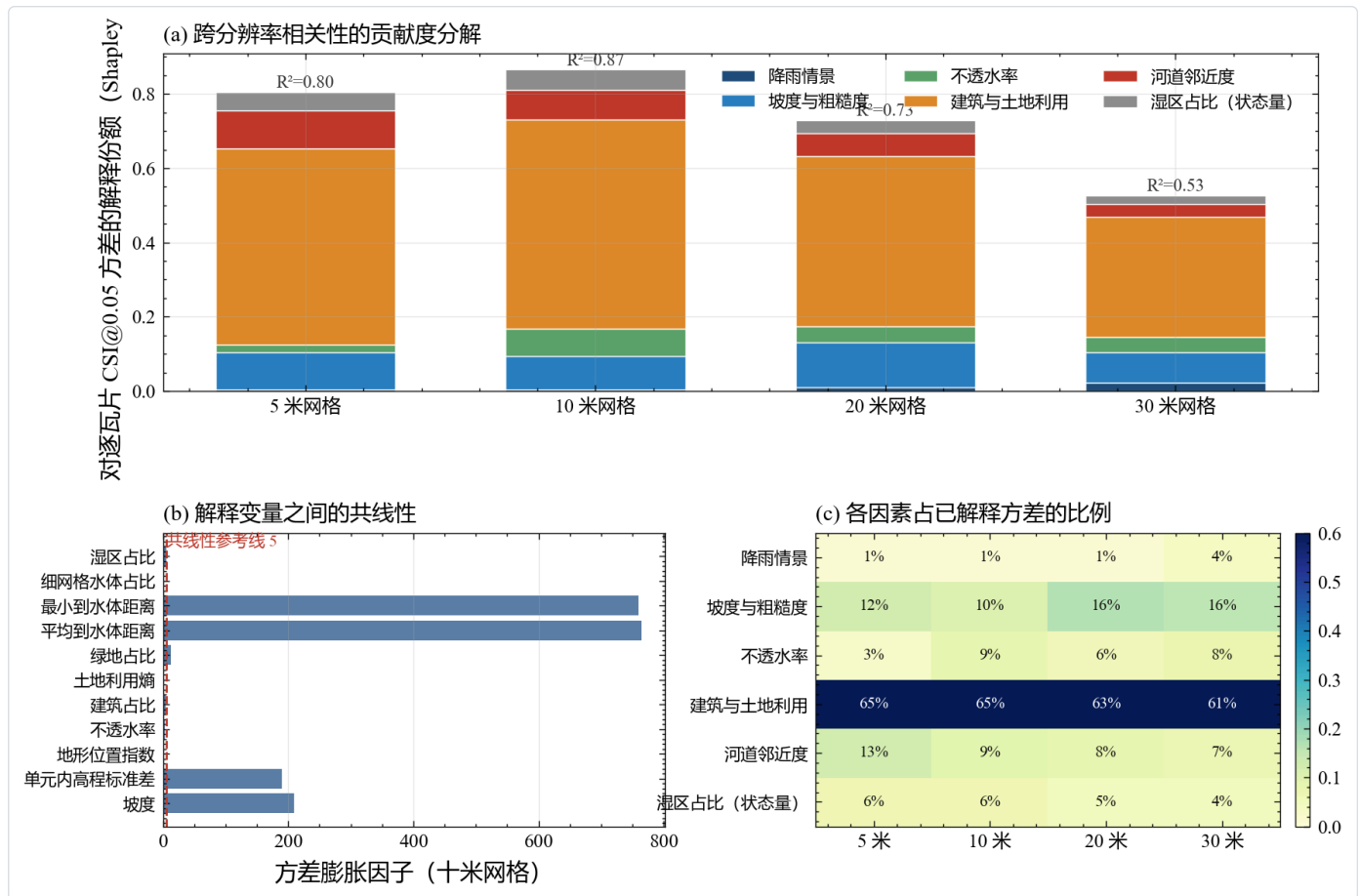
图 31 逐瓦片匹配度的贡献度分解与共线性诊断。子图 (a) 是堆叠柱状图，横轴是四档粗网格的边长，纵轴是各因素对逐瓦片临界成功指数方差的解释份额，也就是分组 Shapley 值。六段颜色对应六组变量，堆叠段之和等于全模型的决定系数，柱顶标注的 R^2 就是这个和。可以读出建筑与土地利用一段在四档网格上都最长，占已解释方差的六成以上，坡度与粗糙度、河道邻近度两段次之，降雨情景一段最短。总高度从十米的 0.865 降到三十米的 0.527，柱子随之明显变矮。子图 (b) 是水平条形图，横轴是方差膨胀因子，纵轴是十米网格用到的十一个解释变量，红色虚线画在 5 的位置作为参考。可以读出坡度与单元内高程标准差两根条最长，都超过 190，两个到水体距离变量都超过 750，说明组内变量高度重合。子图 (c) 是热力图，横轴同样是四档网格，纵轴是六组变量，颜色深浅表示该组占已解释方差的比例，格内的百分数是具体取值，色标范围固定在 0 到 0.6，因此列与列之间可以直接比较。可以读出建筑与土地利用一列在十米处最深，向右逐格变浅，与子图 (a) 中 R^2 的下降方向一致。三个子图合起来的结论是解释力主要来自建筑与土地利用，它在四档网格上都占已解释方差的六成以上。共线性诊断则给出另一条提醒，坡度与单元内高程标准差、两个到水体距离变量高度重合，输入特征应当按组挑选，逐个堆积只会让同一份信息重复计数。
