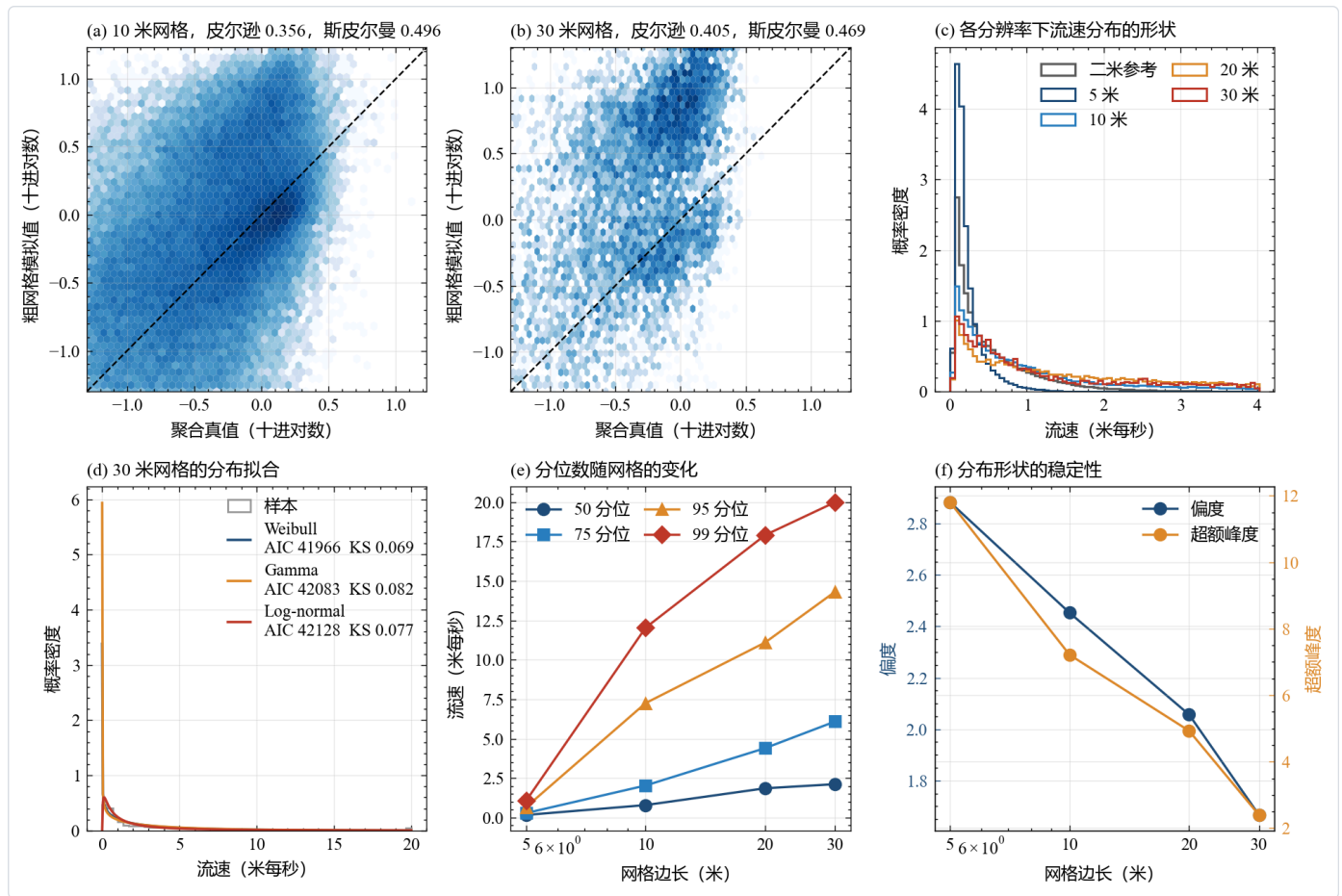
图 17 流速的跨分辨率配对与概率分布。六个子图的排布与图 16 相同，比较对象换成派生流速，时刻仍是全域水量最大的那个整点。（a）与（b）可以读出上层的一条长带，那是水深极小、派生流速极大的单元，它们把皮尔逊系数拉低，却基本不影响等级相关系数。（c）的密度曲线在靠近零的位置有一个很高的峰，尾部一直拖到十米每秒以上，四档网格的曲线位置接近，尾部的差别比水深明显。（d）是三十米网格的分布拟合，最优族与水深不同，厚尾使对数逻辑斯蒂分布与三参数韦布尔分布更有竞争力。（e）与（f）分别给出分位数与矩随网格的变化，分位数曲线在十米处有一个台阶，偏度从五米的 2.88 降到三十米的 1.67，超额峰度从 11.8 降到 2.4。（f）中两条曲线的量级差别很大，读的时候注意纵轴刻度。这张图的小结落在一句话上，流速的失配集中在少数被除法放大的单元。粗化削掉的是流速分布的厚尾，次序结构没有随网格单调恶化，评测流速时因此以等级相关系数为主，皮尔逊系数仅作参考。
