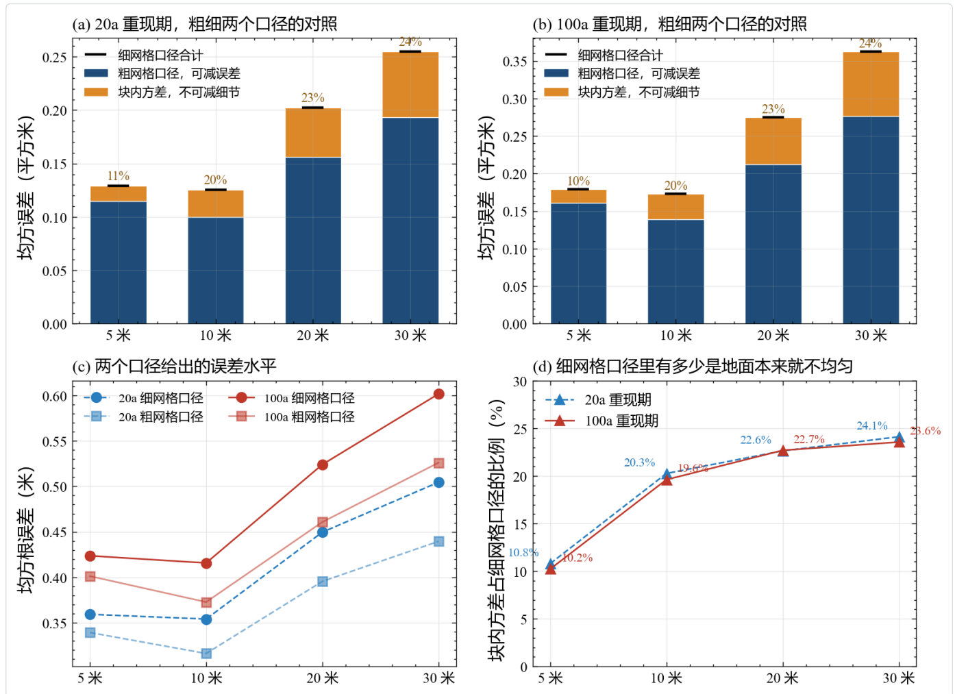
图 11 细网格口径与粗网格口径的对照。四个子图的横轴都是四档网格边长。子图 (a) 与子图 (b) 是堆叠柱状图，分别对应二十年一遇与一百年一遇情景，纵轴是均方误差，单位是平方米。每根柱子分两段，深蓝段是粗网格口径的均方误差，橙色段是块内方差，柱顶标出的百分数是块内方差占细网格口径的比例，柱顶的黑色短横线是细网格口径的合计。可以读出两段的比随网格变粗而改变，粗网格口径一段始终更长，块内方差一段从五米处的约百分之十升到三十米处的约四分之一，深蓝与橙色的分界随网格变粗明显上移。子图 (c) 的纵轴换成均方根误差，单位是米，实线对应一百年一遇，虚线对应二十年一遇，圆点是细网格口径，方点是粗网格口径。可以读出同一情景下细网格口径的曲线始终在上方，两条曲线的间距随网格变粗而拉大，三十米处相差百分之十四到百分之十五。子图 (d) 的纵轴是块内方差占细网格口径的比例，单位是百分数，两个情景各一条曲线，每个点旁标注具体取值。可以读出比例从五米处的约百分之十单调升到三十米处的约百分之二十四，说明网格越粗，细网格口径里属于地面本来不均匀的份额越大。需要带走的一条判断是，用细网格口径报告误差会系统性地高估模型的不足，这个间距来自地面本身的不均匀。
