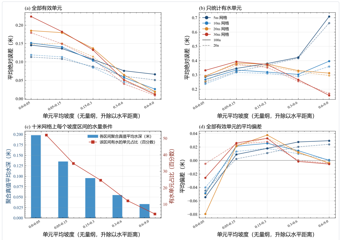
图8 按单元平均坡度分层的误差结构。四个子图的横轴都是单元平均坡度区间，依次为0至0.05、0.05至0.15、0.15至0.3、0.3至0.6、0.6至9.0。单位为无量纲，坡度按垂直高差除以水平距离定义，因此0.3表示水平前进一米上升三十厘米。子图(a)是全部有效单元的平均绝对误差，单位是米，颜色对应四档网格，实线是一百年一遇情景，虚线是二十年一遇情景。可以读出一个下降的走势。十米网格、一百年一遇情景下五个区间的数值依次是0.1515、0.1406、0.1036、0.0575与0.0260米，从最平坦到最陡一路变小，最陡区间只有最平坦区间的六分之一。子图(b)把统计范围收窄到有水单元，纵轴仍是平均绝对误差，单位是米，颜色与线型规则同前。可以读出走势变了样。十米网格、一百年一遇情景下五个区间的数值变成0.268、0.334、0.319、0.304与0.396米，最陡区间比最平坦区间高约五成，中间三段几乎持平，没有单调的走向。子图(c)解释了两条数列为什么不同，横轴同为坡度区间，蓝色柱子是各区间聚合真值的平均水深，用左轴读数，单位是米，红色方点线是该区间有水单元的占比，用右轴读数，单位是百分数。可以读出最平坦区间有五成二的单元有水，平均水深0.198米，最陡区间只有百分之四有水，平均水深0.033米。干湿比例随坡度急剧下降，这正是子图(a)那条下降曲线的来源。子图(d)是全部有效单元的平均偏差，单位是米，横线标出零，规则同子图(a)。可以读出偏差在五个区间上都很小，最平坦区间为负0.049米，其余四个区间落在正负0.03米以内，坡度分层没有给出像水深分层那样清晰的方向。读分层统计时先看清每个区间里有多少水，坡度本身不足以决定误差的大小。
