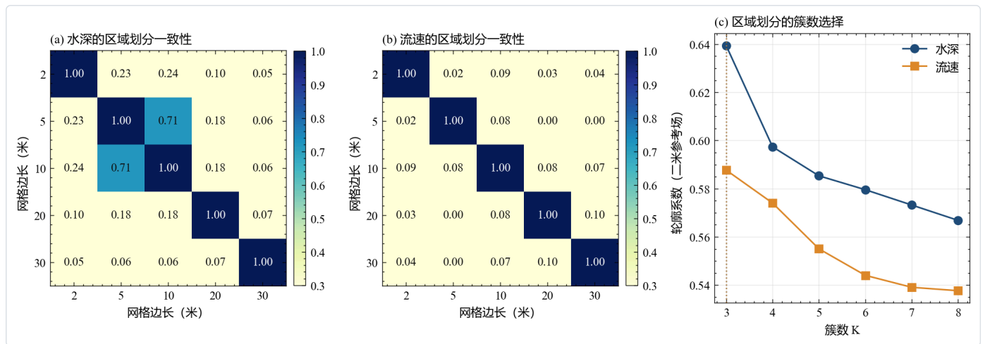
图 18 跨分辨率空间模式相似性矩阵。（a）与（b）分别是水深与流速的区域划分一致性矩阵，行列都是五档分辨率，格子内的数字是两档划分之间的 V-measure，五米与十米两档之间的共同结构保留得最多。（c）是簇数选择，横轴是 K 均值聚类的簇数，纵轴是二米参考场上的轮廓系数，两条曲线的最高点都在三，也就是后面统一使用的簇数。两个矩阵的对角线都是 1。水深矩阵里五米与十米这一格深达 0.71，十米与二十米掉到 0.18，二十米与三十米只剩 0.07，说明区域结构只在相邻的分辨率之间留得住。流速矩阵整体更浅，最深的非对角元也只有 0.10。把同质性与完备性分开看，两个分量几乎相等，四档上的差值都在 0.02 以内，说明一致性的损失没有偏向哪一侧。三个子图合起来只支持一条结论，区域划分只能在与两米相邻的那一档之间传递。水深矩阵里五米与十米这一格达到 0.71，十米与二十米掉到 0.18，二十米与三十米只剩 0.07，流速矩阵最深的非对角元也只有 0.10，簇数则在两个变量上都选在三。
