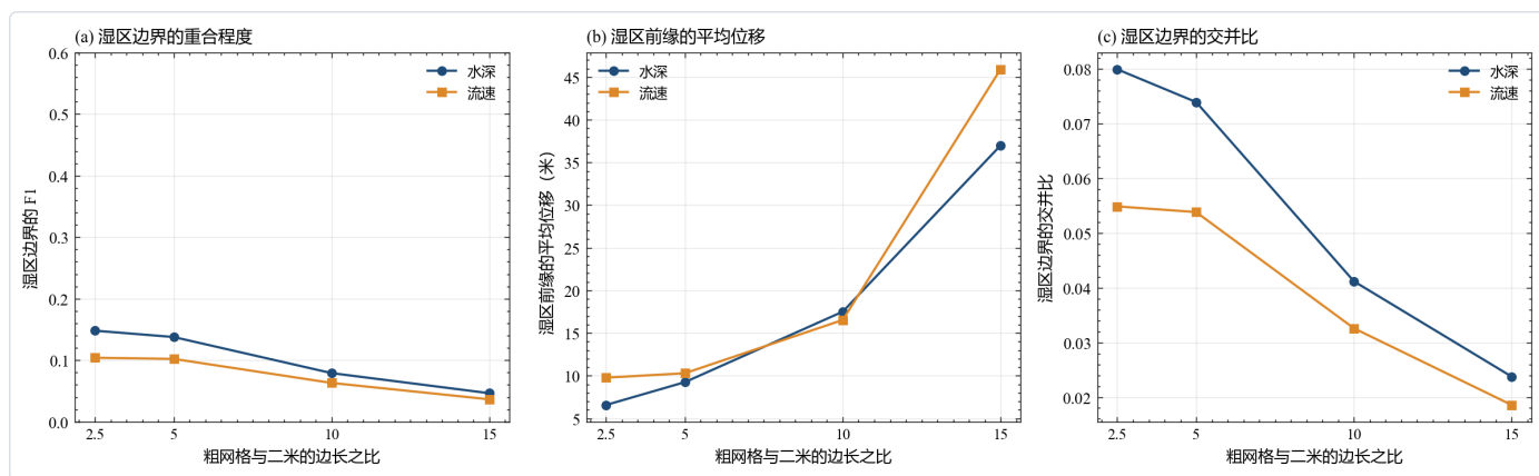
图 22 湿区前缘的重合程度。掩膜一律由水深场给出, 阈值取五厘米, 水深用事件最大值, 流速取峰值水量那一小时的瞬时水深。边界由形态学腐蚀得到, 原掩膜减去腐蚀结果就是一圈边界像元。(a) 是两圈边界的 F1, (b) 是两条前缘线之间的修正豪斯多夫距离, 取两个方向里较大的一个, (c) 是边界交并比。水深上前缘 F1 从五米的 0.148 降到三十米的 0.046, 修正豪斯多夫距离从 6.58 米升到 36.98 米。流速上前缘 F1 更低, 五米是 0.104, 三十米是 0.036。就本图而言, 区域内部的标号一致性远高于前缘线的一致性, 四对前缘 F1 最高只有 0.148。五米与十米这一对在区域内部有 0.714 的 V-measure 与 0.891 的平均交并比, 边界比较里没有出现同量级的取值, 分辨率的损失主要落在湿区轮廓上。
