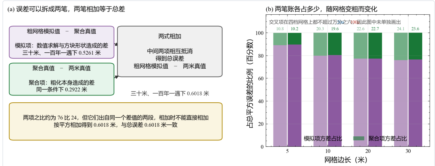
图 4 误差的三笔账与两笔账的份额。子图 (a) 是一张加法示意，用三十米网格、一百年一遇情景的真实数值作例子。上两个方框分别写出第一笔与第二笔，第一个方框是粗网格模拟值减去聚合真值，对应数值求解与方块形状造成的差，方框内注明这一项在两米格网上的均方根是 0.5261 米。第二个方框是聚合真值减去两米真值，对应粗化本身造成的差，同一条件下的数值是 0.2922 米。右侧方框指出两式相加时中间的聚合真值一正一负相互抵消，于是得到第三个方框，也就是粗网格模拟值减去两米真值，数值是 0.6018 米。最下方一条黄色方框写的是读法提醒，两个分项出自同一个差值的两段，不能直接相加，只有先平方再相加才能还原总数，按这个做法算得 0.6018 米，与总误差一致。子图 (b) 把两笔账的份额画成堆叠柱状图，横轴是四档网格边长，纵轴是占总平方误差的比例，百分数。每一档有左右两根柱子，左侧是二十年一遇情景，右侧是一百年一遇情景，紫色段是模拟项，绿色段是聚合项，绿色段上方的数字是聚合项的具体份额。可以读出三件事。模拟项在每一档上都占大头，最少也有约四分之三。聚合项的份额随网格变粗而上升，从五米的约百分之十升到三十米的约百分之二十四。交叉项在四档网格上都不超过万分之六，因此图中不单独画出。一旦网格继续放粗，粗化造成的信息损失在总误差里的比重还会上升，这时单靠改进数值格式已经收效不大。
