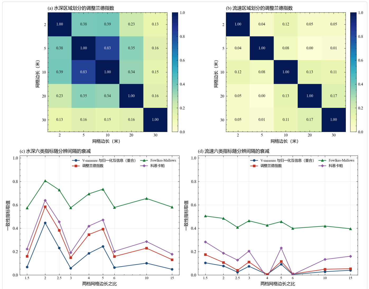
图 20 机会校正后的区域划分一致性。(a) 与 (b) 是水深与流速的调整兰德指数矩阵，行列都是五档分辨率，对角线取一。每个矩阵里只有一个明亮的格子，水深是五米与十米这一对，取值 0.830。(c) 与 (d) 把六类指标按两档网格的边长之比排列，横轴是对数刻度，纵轴是取值范围。信息论那条曲线是 V-measure 与归一化互信息，两者在算术归一化下恒等，图上完全重合，调整互信息与它们的差落在小数点后第五位，因此只画一条。四条曲线在排序上互相印证，水深五米与十米这一档的调整兰德指数是 0.830、Fowlkes-Mallows 是 0.922、科恩卡帕是 0.870。二米与三十米这一档只剩 0.131、0.580 与 0.178。Fowlkes-Mallows 的绝对水平最高，因为它在簇占比不均时的随机期望值就达到 0.516。就本图而言，扣除机会水平之后，二米与三十米的 Fowlkes-Mallows 只剩 0.064 的净超出，水深的区域结构只在五米与十米之间真正留存。
