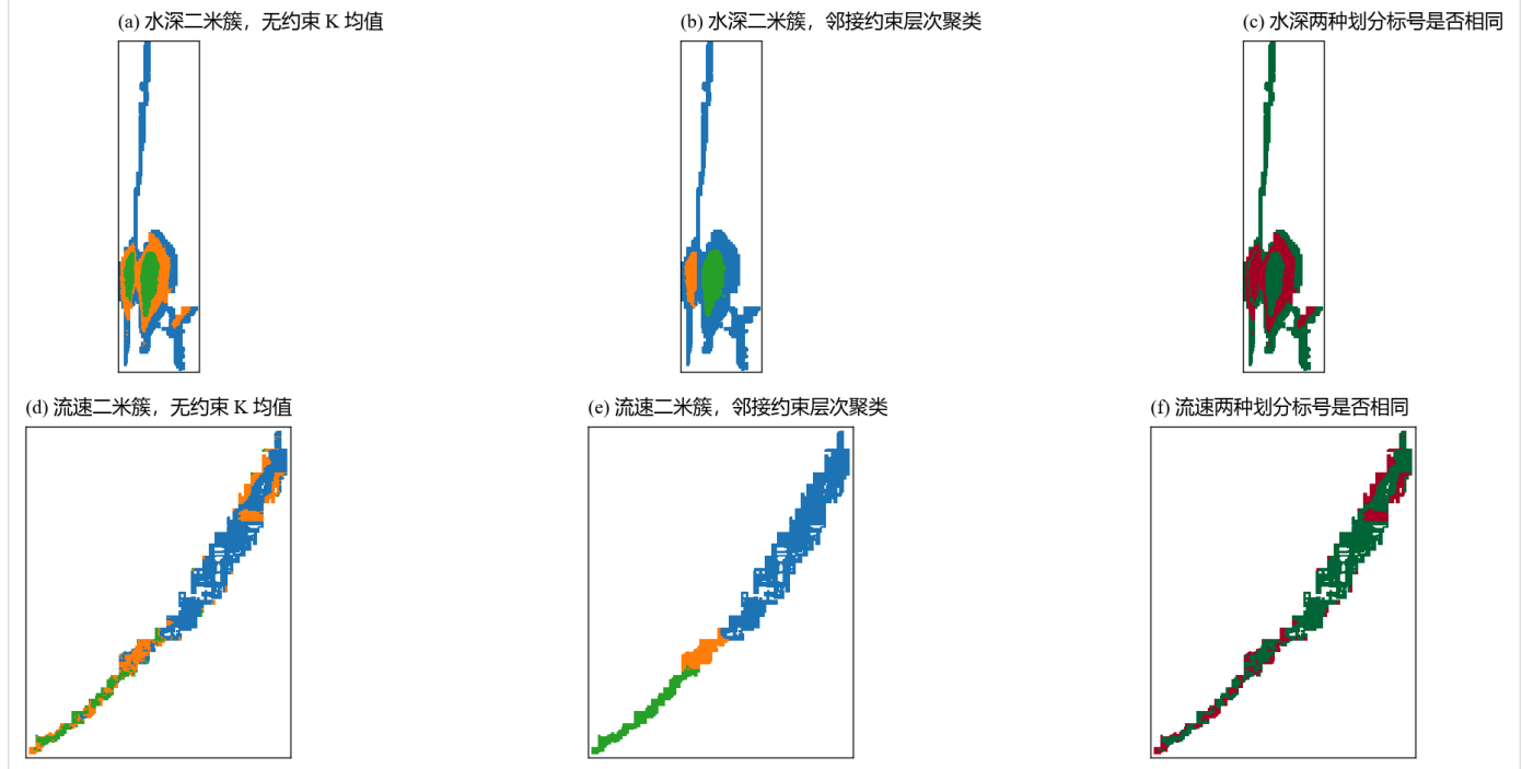
图 27 最大连通核上的区域划分对照。上排三幅是水深，下排三幅是流速，每排的第一幅是无约束 K 均值划分，第二幅是加入上下左右邻接约束的 ward 层次聚类划分，第三幅用红绿两色标出两种划分标号是否相同，绿色表示相同。两幅划分图共用一个簇编号色标，编号按单元的平均对数水深排序。核由湿区做一次三乘三闭运算后取最大连通分量得到，水深核有 23317 个单元，流速核有 5047 个。就本图而言，同一个二米水深场上两种划分的 V-measure 只有 0.468，说明无约束 K 均值给出的簇在空间上是碎的，加约束之后簇才连成片。
