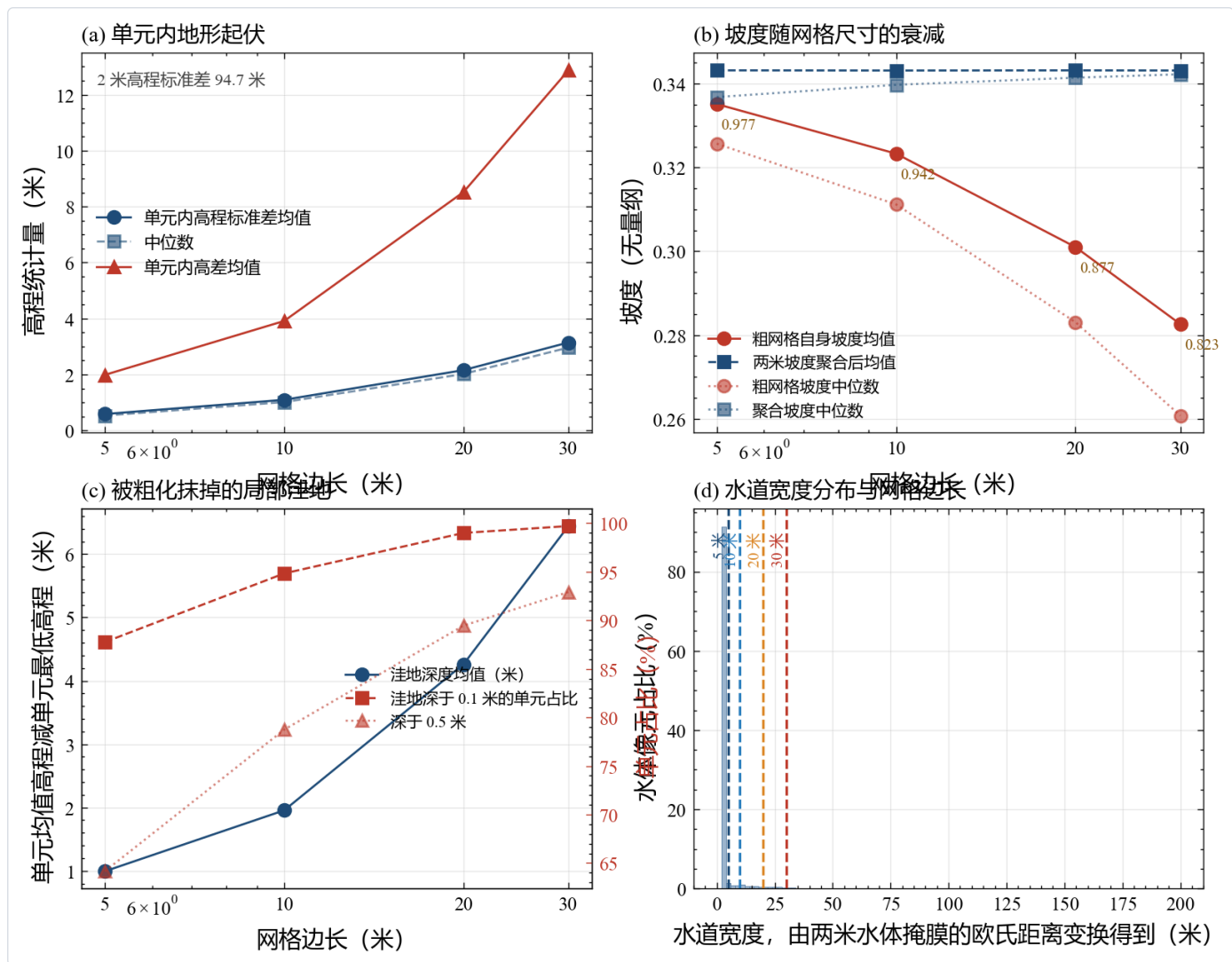
图 13 地形失真随网格尺寸的变化。四个子图的横轴都是网格边长，取五、十、二十、三十米四个值并按对数刻度摆放。子图 (a) 的纵轴是高程统计量，单位是米，深蓝实线圆点是单元内高程标准差的均值，深蓝虚线方点是同一量的中位数，红色三角实线是单元内高差均值。可以读出三条曲线都随边长线性上升，标准差均值从 0.589 米升到 3.145 米，高差均值从 1.99 米升到 12.87 米。中位数始终低于均值，说明分布右偏，少数单元内部的起伏远大于平均水平。图内左上角的文字给出两米全域的高程标准差，用来提示单元内的量远小于全域名。子图 (b) 的纵轴是坡度，无量纲，红色圆点实线是粗网格自身算出的坡度均值，深蓝方点虚线是把两米坡度聚合到同一网格后的均值，两条细点线是对应的中位数。可以读出聚合曲线在四档上都停在 0.343，而粗网格模拟的曲线从 0.335 单调降到 0.283。曲线旁的注释给出两者的比值，从 0.977 降到 0.823。比值小于一表示粗网格把地形看缓。子图 (c) 使用双纵轴。左轴是单元内高程均值减单元内最低高程，单位是米，对应蓝色圆点实线，它从 0.99 米升到 6.44 米。右轴是满足深度条件的单元占比，单位是百分数，对应两条红色虚线，深于零点一米的占比从 87.8% 升到 99.7%，深于零点五米的从 64.2% 升到 92.9%。可以读出两条占比曲线在二十米之后接近饱和，说明局部洼地的丢失在二十米档已经基本完成。子图 (d) 的横轴是水道宽度，单位是米，由两米水体掩膜的欧氏距离变换得到，纵轴是水体像元占比，单位是百分数。浅蓝色直方图是宽度分布，四条竖虚线标出四档网格边长，分别写在竖线顶端。可以读出直方图集中在最小分辨宽度附近，绝大多数水体像元的宽度落在第一条竖线的左侧，也就是比五米网格还要窄。粗网格无法分辨城市里的细窄水道，读这张图时先看曲线随边长的走向，再看竖线与直方图的相对位置。四幅子图给出的阶段性结论是粗化同时放大了单元内的起伏、削平了坡度、填掉了局部洼地。其中洼地的丢失在二十米档已经基本完成，因此前置校正使用地形派生特征时，这部分损失只能从外部估计，无法在数值格式里修正。
