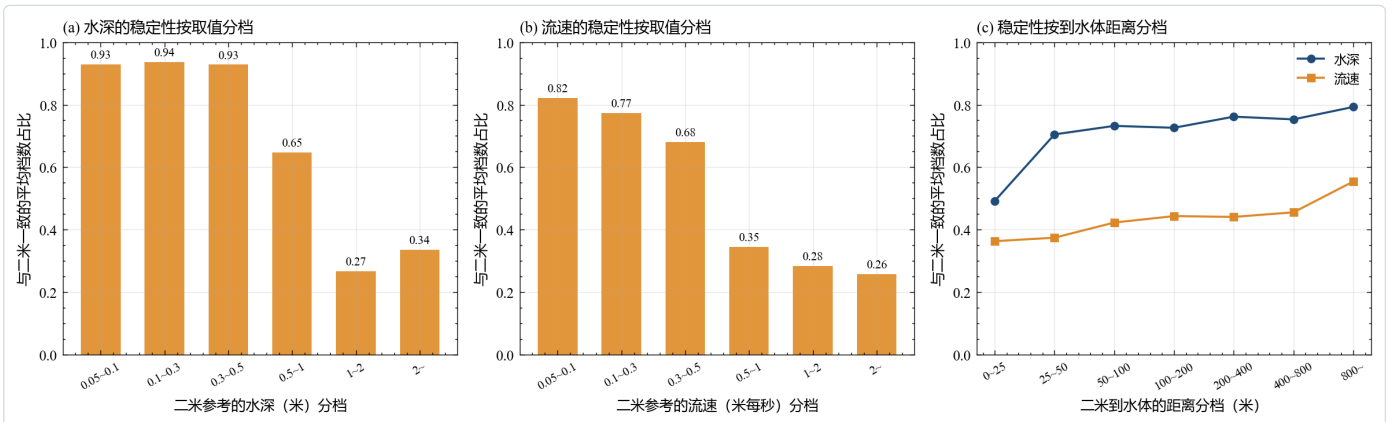
图 24 一致性按取值与到水体距离拆开。稳定档占比按二米参考的标号统计，把四档粗网格的簇各自按重叠面积映射到参考簇之后，逐单元数出四档里有几档给出与参考相同的标号，再除以四。（a）与（b）是水深与流速按取值分档的结果，横轴是二米参考自己的取值区间。（c）是两条曲线按到水体距离分档的结果，横轴是二米到最近水体的距离区间。水深在五厘米到半米之间的三个档，稳定档占比都在 0.93 上下，半米到一米降到 0.647，一到两米只有 0.267。到水体的距离给出同样的方向，零到二十五米这一档只有 0.492，四百米到八百米升到 0.753，八百米之外是 0.793。流速的规律相同而水平更低，两米以上的流速档只有 0.258。就本图而言，稳定档占比在半米以内都在 0.93 上下，一到两米只剩 0.267，零到二十五米这一档只有 0.492，跨分辨率的一致集中在浅水区与远离河道的位置。
