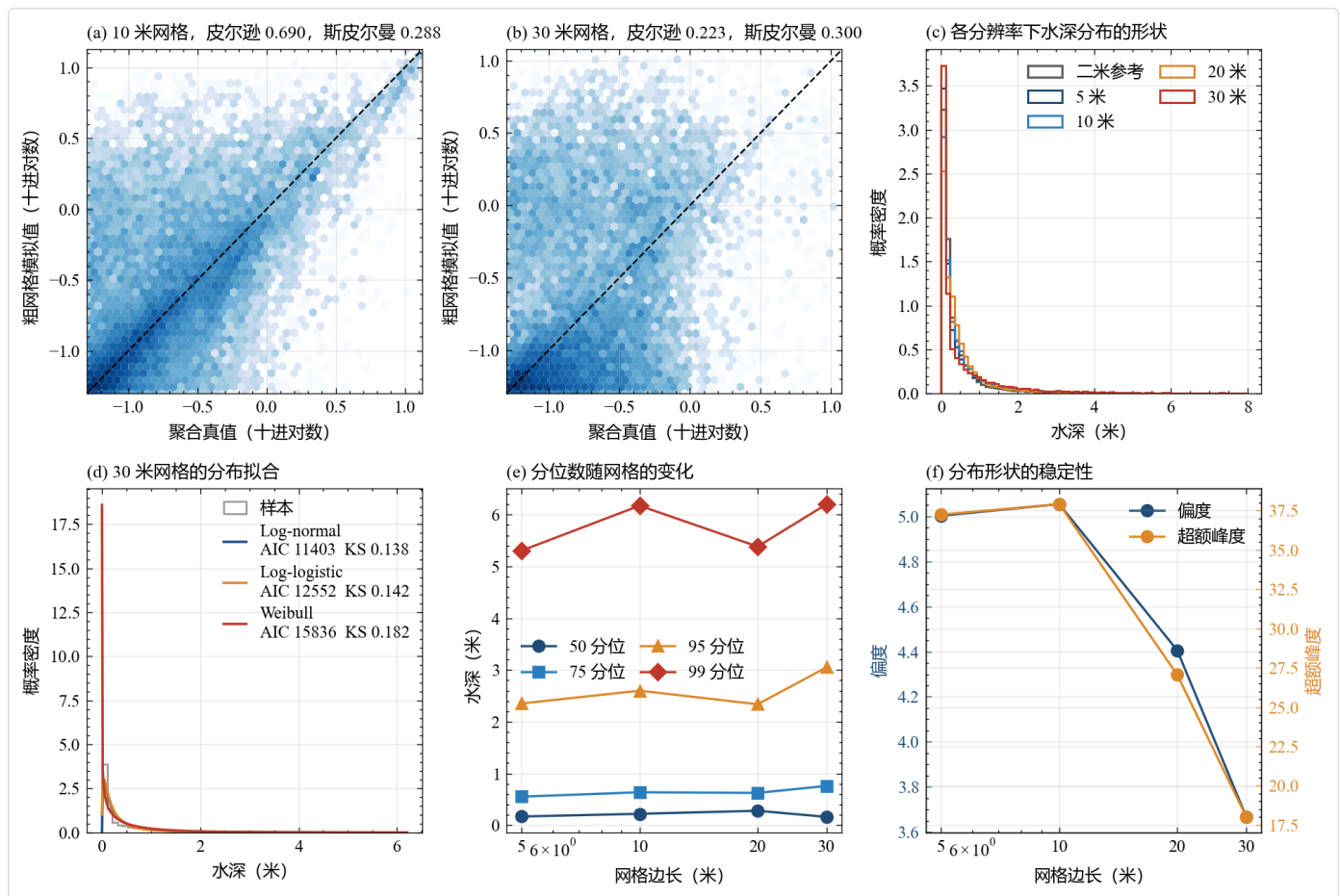
图 16 水深的跨分辨率配对与概率分布。(a) 与 (b) 是一百年一遇情景下十米与三十米网格的配对散点图, 横轴是聚合后的二米真值, 纵轴是同一单元上的粗网格模拟值, 两个轴都做了十进对数变换以便看清小值区, 颜色深浅表示该范围内的单元数。虚线是两者相等的等值线。点云整体沿等值线铺开, 随网格变大而变宽, 皮尔逊系数因此从十米的 0.690 降到三十米的 0.223。等级相关系数在四档之间保持在 0.23 到 0.30, 不随网格继续恶化, 但它的绝对值始终不高, 说明次序信息在粗网格上也只保住了一小部分。(c) 是四档网格与二米参考的水深概率密度, 五条曲线都只用湿区单元, 横轴截到百分之九十九点五分位。五条曲线的左端几乎重合, 粗网格的曲线在中高段略微右移, 差别集中在右侧尾部。(d) 是三十米网格的分布拟合, 灰线是样本直方图, 三条彩线是赤池信息量准则最小的三个分布族, 图例给出族名、AIC 与 KS 统计量。(e) 是四个分位数随网格边长的变化, 横轴取对数刻度, 曲线整体平坦, 只有百分之九十九分位在二十米之后略微抬升。(f) 是偏度与超额峰度随网格的变化, 两个量的量级相差很多, 因此用左右两条纵轴。两条曲线都随网格下降, 说明粗化把分布的尾部削轻了。
