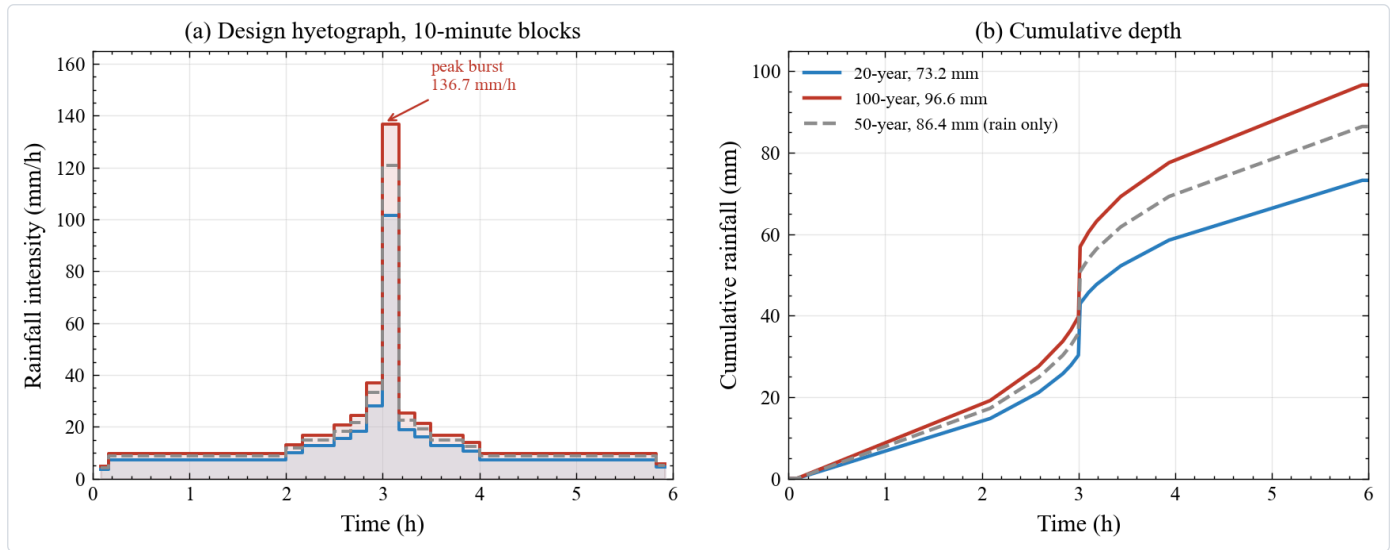
图 33 三个重现期的设计暴雨时程。两个子图共用同一个横轴，即从零到六小时的降雨历时，单位是小时。左子图 (a) 是十分钟区块的降雨强度，纵轴单位是每小时毫米。曲线画成阶梯形而不是平滑曲线，原因是原始雨型由分段常数构成，每个十分钟区块内强度保持不变，阶梯画法如实反映了这一点。右子图 (b) 是累计降雨深度随时间的变化，纵轴单位是毫米，它等于左子图曲线到当前时刻的积分面积。三条曲线的重现期分别是二十年、五十年与一百年，其中五十年只有降雨过程而没有对应的洪水模拟结果，因此用虚线区分，只作为强度参照，不参与建模。本图只作雨型展示，不承担分析结论。需要记住的一点是，五十年一遇一档只有降雨过程，没有对应的洪水模拟结果，因此本报告的洪水结论只覆盖二十年与一百年两档。
