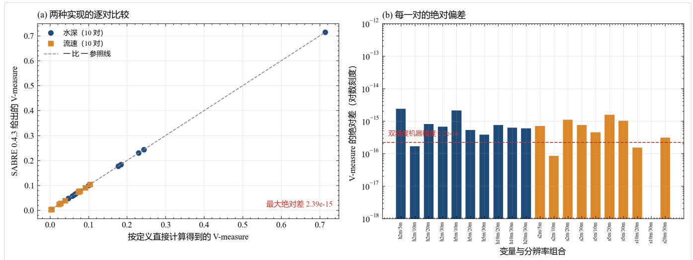
图 25 SABRE 0.4.3 与直接计算的逐对对照。子图 (a) 的横轴是按定义直接算出的 V-measure，纵轴是 R 语言 SABRE 包给出的 V-measure，颜色区分水深与流速，圆点与方块各代表一本变量上的十个分辨率组合，虚线是一比一参照线。子图 (b) 把每一对上的绝对差单独画出，横轴按变量与分辨率组合排列，纵轴取对数刻度，红色虚线标出双精度机器精度。本图用的是 K 等于三、随机种子 20260921 的同一批标号栅格，Python 侧写入 GeoTIFF，R 侧读入后按多边形区域划分计算。就本图而言，二十对数值全部落在参照线上，最大绝对差只有 2.39\text{e-}15 ，约为双精度机器精度 2.22\text{e-}16 的十一倍，处在浮点累加舍入的量级，两种实现给出的是同一个量。
