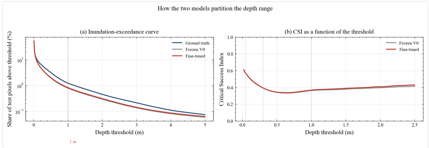
图 51 淹没超限曲线与阈值敏感性。 超限曲线在水文学中用来描述超过某一量级的事件有多普遍，这里把水深当作量级，曲线上的每一点表示水深超过该阈值的像元占全部像元的多大比例。(a)是这一比例随水深阈值的变化，横轴是水深阈值，单位是米，纵轴是像元占比，采用对数标度，因为占比从百分之十量级迅速衰减到千分之几，线性纵轴会把深水段压成一条贴底的直线，看不出差别。三条曲线分别是真值、冻结基线与微调。红色点线标出一米位置，是深水与浅水的分界，也是本报告最关心的区段。(b)是判定指标随水深阈值的变化，横轴同为阈值，纵轴是取值在零到一之间的临界成功指数。灰色点线标出零点零五、零点三零与一米三个常用阈值。两个子图必须合起来读，(a)说明有多少水面被漏掉，(b)说明在什么水深上最容易判错，前者是后果，后者是原因。两个子图合起来指向同一个要点，低阈值下的判定指标会掩盖后果。零点零五米阈值处的取值在零点五六附近，但同一阈值下淹没面积已经比真值少百分之八，而在更受关注的高水深区间，面积缺失接近四成。由此可以定下一条汇报要求，给出指标时必须同时给出阈值与对应的面积偏差。
