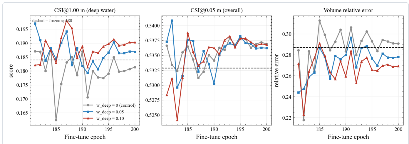
图 19 三个微调实验臂在全验证集上的逐轮表现。三个子图共享横轴，即第一百八十一轮到第二百零轮，每点是全量评估结果。灰色圆点是权重为零的对照臂，蓝色方块是权重 0.05 的臂，红色三角是权重 0.10 的臂，两条虚线是冻结基线的水平。权重 0.10 的微调臂把深水指标抬高 0.014，整体指标只变化 0.0004，两个代价都被压在很小的幅度内。
