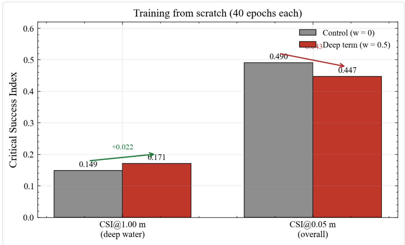
图 18 从头训练时深水权重的收益与代价。横轴分成深水指标与整体指标两组，每组内左柱是权重为零的对照臂，右柱是权重 0.5 的实验臂。两组柱子的走向相反，这正说明深水与整体之间存在取舍关系。从头训练把深水权重提到 0.50，深水指标升 0.022，整体指标却降 0.043，代价约为收益的两倍。
