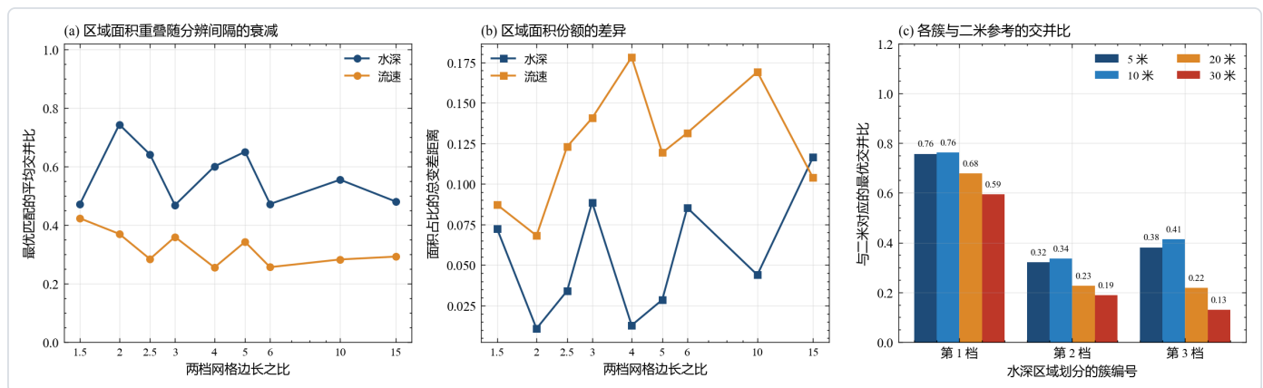
图 13 区域面积的重叠与份额差异。子图 (a) 是最优匹配平均交并比，匹配由匈牙利算法在交并比矩阵上求最大总收益得到。子图 (b) 是各簇面积占比的总变差距离，子图 (c) 把逐簇交并比按簇编号拆开。水深五米与十米的平均交并比是 0.891，二米与三十米降到 0.480，主体簇仍有 0.594 而最小簇只剩 0.130，面积的损失先落在小簇上。
