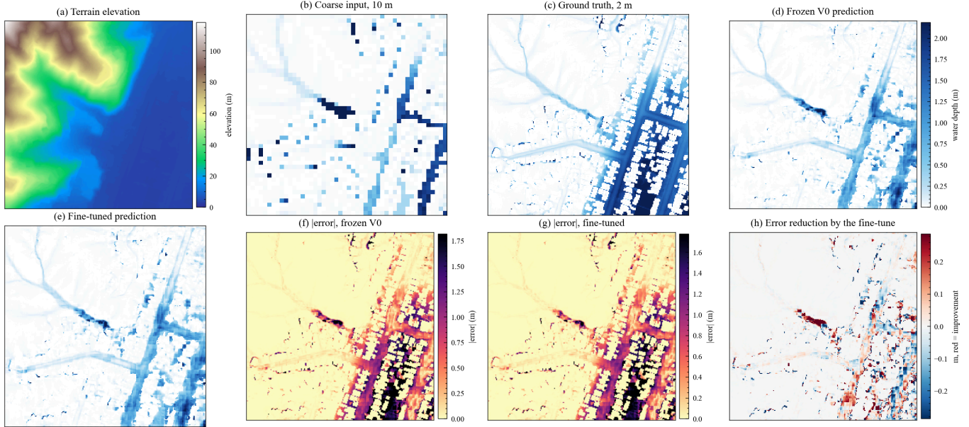
图 17 测试集中深水像元最多的瓦片，八面板逐格对比。该瓦片属于一百年重现期情景，位于网格第四十二行第十列，真值峰值 4.07 米，水深超过一米的像元有 7908 个。上排是地形、粗输入、真值与冻结基线预测，下排是微调预测、两张绝对误差图与误差削减量。这一格的平均绝对误差从 0.672 米降到 0.666 米，深水判定指标从 0.201 降到 0.189，45.4% 的像元误差变小。
