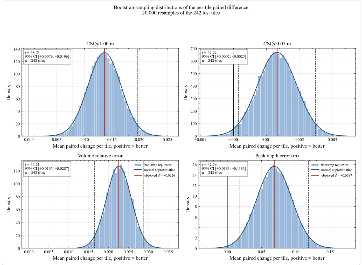
图 20 逐瓦片配对差值的自助法抽样分布。四个子图分别对应深水判定指标、整体判定指标、体积相对误差与峰值深度误差。所有指标都已统一符号，正值表示微调更好。柱状图是对瓦片有放回地重抽样得到的均值分布。深水判定指标与体积相对误差的平均改善分别是 0.0137 与 0.0226，普通自助法区间都不跨零，整体判定指标只有 0.0013，区间宽度超过均值本身。但这套区间假定瓦片之间可以互相替换，忽略了误差的空间自相关，区间因此偏窄，重估后的结论以图 21 之后的说明为准。
