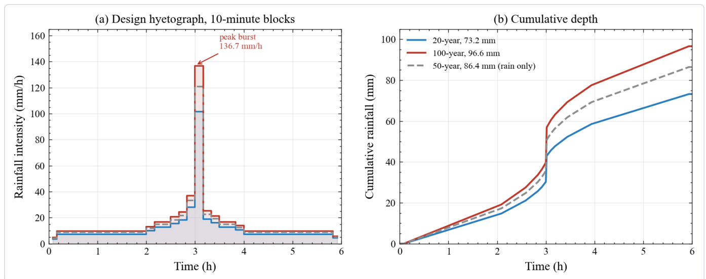
图2 三个重现期的设计暴雨时程。左子图是十分钟区块的降雨强度，曲线画成阶梯形，因为原始雨型由分段常数构成。右子图是累计降雨深度，等于左曲线到当前时刻的积分面积。五十年一遇一档只有降雨过程，因此本报告的洪水结论只覆盖20年与100年两档。
