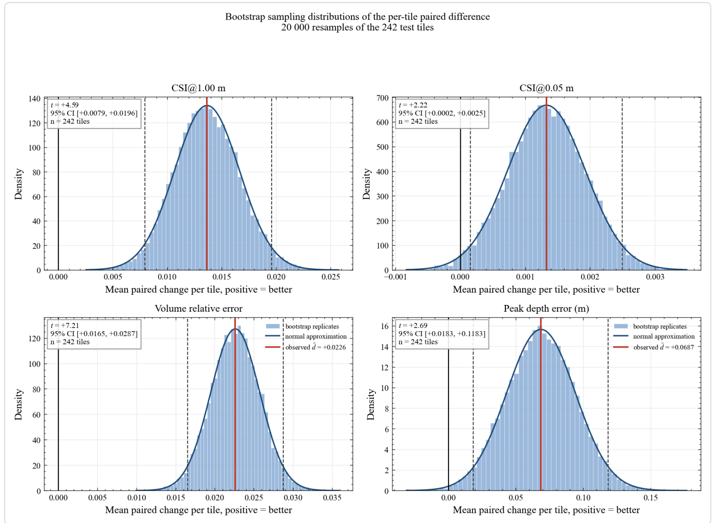
图 46 逐瓦片配对差值的自助法抽样分布。四个子图 (a) 至 (d) 分别对应深水判定指标、整体判定指标、体积相对误差与峰值深度误差。这里把配对单位换成了瓦片，也就是拿同一块地面在两个模型上的表现相比，两百四十二块测试瓦片因此给出两百四十二对数值。横轴是两个模型在这批瓦片上的平均差值，所有指标都已统一符号，正值表示微调更好，负值表示更差，这样四个子图的方向可以放在一起看。柱状图是对瓦片有放回地重新抽样两万次得到的均值分布，它刻画的是这个平均差值在换一批瓦片时会有多大波动。深色曲线是均值与标准差相同的正态分布，用来检查自助分布在有限样本下是否仍然接近正态，两者贴合说明用正态区间不会失真。黑色实线在零处，红色实线是实测均值，两条虚线夹出的范围是自助法给出的百分之九十五置信区间。各子图左上角的文本框给出统计量、置信区间与配对样本量。四个子图的小结分成两组。深水判定指标与体积相对误差的平均改善分别是正零点零一三七与零点零二二六，置信区间都不跨零，方向可靠。整体判定指标的平均改善只有零点零零一三，区间的宽度已经超过均值本身，改善存在但边缘。峰值深度误差的方向最不稳定。把四个指标放在一起，最稳的两个都落在深水与水量上，本报告的改动价值也正集中于此。
