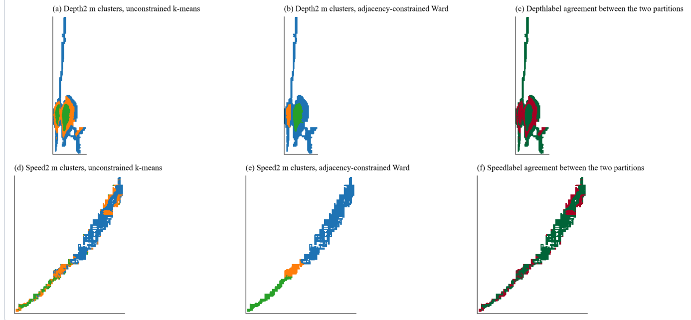
图 27 最大连通核上的区域划分对照。 上排三幅是水深，下排三幅是流速，每排的第一幅是无约束 K 均值划分，第二幅是加入上下左右邻接约束的 ward 层次聚类划分，第三幅用红绿两色标出两种划分标号是否相同，绿色表示相同。两幅划分图共用同一个簇编号色标，编号按单元的平均对数水深排序。核由湿区做一次三乘三闭运算后取最大连通分量得到，水深核有 23317 个单元，流速核有 5047 个。就本图而言，同一个二米水深场上两种划分的 V-measure 只有 0.468，说明无约束 K 均值给出的簇在空间上是碎的，加约束之后簇才连成片。
