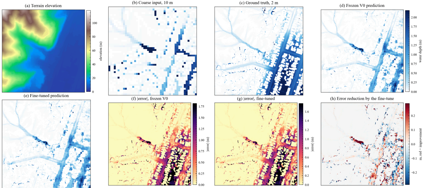
图 40 测试集中深水像元最多的瓦片，八面板逐格对比。该瓦片属于百年重现期情景，位于网格第四十二行第十列，真值峰值四点零七米，水深超过一米的像元有七千九百零八个。上排四个面板依次是地形高程、十米粗分辨率输入、两米真值以及冻结基线的预测。下排依次是微调后的预测、冻结基线的绝对误差、微调后的绝对误差，以及微调相对冻结基线的误差削减量。误差削减面板中红色表示微调在这一格把误差改小了，蓝色表示改大了，颜色标尺对称于零。读这张图有一个最要紧的前提。上排四个深度面板共用同一套色标与量程，量程上限取这一格真值的九十九点五百分位，也就是二点一八六米，它们之间可以直接横向比较。下排两张误差面板不是这样，每一张各按自身绝对误差的九十八百分位单独设定量程，冻结基线约一点八二米，微调约一点七八米，最右侧的削减面板则对称于零。因此误差面板的深浅只能同一张面板内部读，不能拿去和深度面板比多少，这是读本图最要紧的一条限制。还要交代这一格的抽样身份。它是两百四十二块测试瓦片里最深的一块，湿区平均绝对误差零点六七二米，约为全量瓦片该指标宏平均零点二零六米的三点三倍，属于最不利的一格，不能当作典型瓦片来读。误差的分布也很不均匀。这一格的最大绝对误差是四点零四米，而误差面板在九十八百分位处截断，超出这一值的像元在图上饱和成最深色，同时百分之七十四的有效像元绝对误差不到零点零五米。逐像元统计给这一格定下一句判断，百分之四十五点四的像元误差变小，百分之四十七点五变大，平均绝对误差从零点六七二米降到零点六六六米，深水判定指标从零点二零一降到零点一八九。净改善存在，但单格抽样的波动足以盖过真实效应，判断必须依靠全量配对统计。
