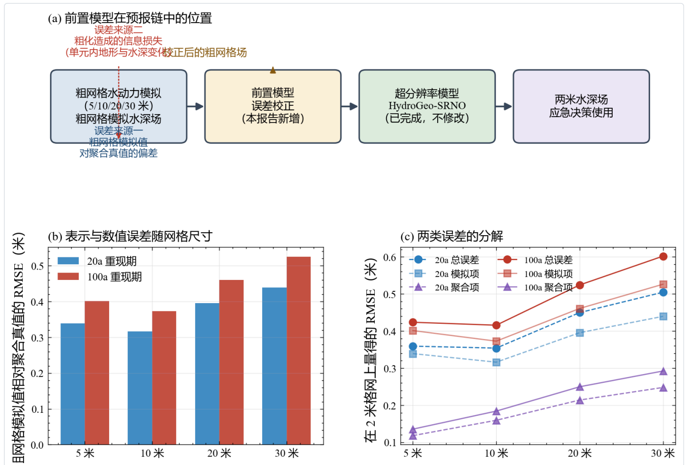
图5 前置模型在整个预报链中的位置与两类误差的量级。子图(a)是一条流程示意。第一个方框是粗网格水力模拟, 它给出边长五米到三十米的粗网格模拟水深场。第二个方框是本章新增的前置模型, 它读取粗网格水深场与同一档粗网格上的静态地理特征, 输出一个校正后的粗网格场。第三个方框是已经完成的超分辨率模型 HydroGeo-SRNO, 本章不对它做任何改动。第四个方框是最终交付的两米水深场。方框之间的箭头表示数据流向, 校正后的场同时向上反馈一条虚线, 标注的是两类误差的来源。虚线来自粗化本身的信息损失, 也就是单元内地形起伏与水深变化在取平均时被抹平的那一部分。子图(b)是柱状图, 横轴是四档网格边长, 纵轴是粗网格模拟值相对聚合真值的均方根误差, 单位是米, 两种颜色对应二十年一遇与一百年一遇两个情景。柱子越高表示粗网格离聚合真值越远。可以读出两个特征, 十米处的柱子最低, 二十米与三十米处的柱子明显抬升, 且一百年一遇情景整体高于二十年一遇。子图(c)把总误差拆成模拟项与聚合项, 横轴同样是网格边长, 纵轴是在两米格网上量得的均方根误差, 单位是米。圆点连线是总误差, 方点是模拟项, 三角点是聚合项, 实线对应一百年一遇, 虚线对应二十年一遇。可以读出模拟项始终高于聚合项, 且两者都随网格变大而上升, 但聚合项上升的速度更快, 说明网格越粗, 信息损失在总误差里的比重越大。
