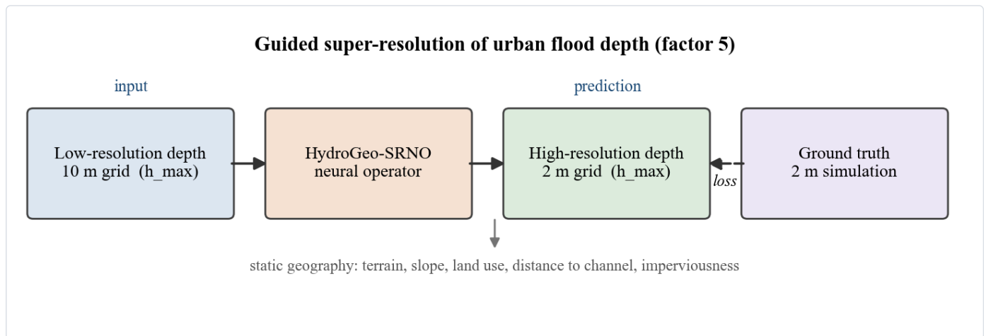
图1 引导式超分辨率任务的输入与输出。左侧方框是模型的输入，即十米网格上的最大淹没水深场。这里说的最大淹没水深，指的是一场降雨全过程中每个位置达到过的最大水深，它比某个瞬时水深更能代表风险，因为它记录的是最不利的时刻。中间是完成映射的神经网络。右侧是模型输出的两米网格水深，训练时与独立的高分辨率模拟结果逐像素比对。下方箭头表示静态地理信息同时输入模型，它不随降雨情景变化，但对判断水往哪里流至关重要。这类结构与图像超分辨率的差别在于，低分辨率输入是一次完整的水动力求解结果，与高分辨率真值之间没有降采样关系。两者之间也就不存在确定的解析关系，因此模型无法靠套用现成的插值公式得到答案，必须真正理解地形对水流的约束。
