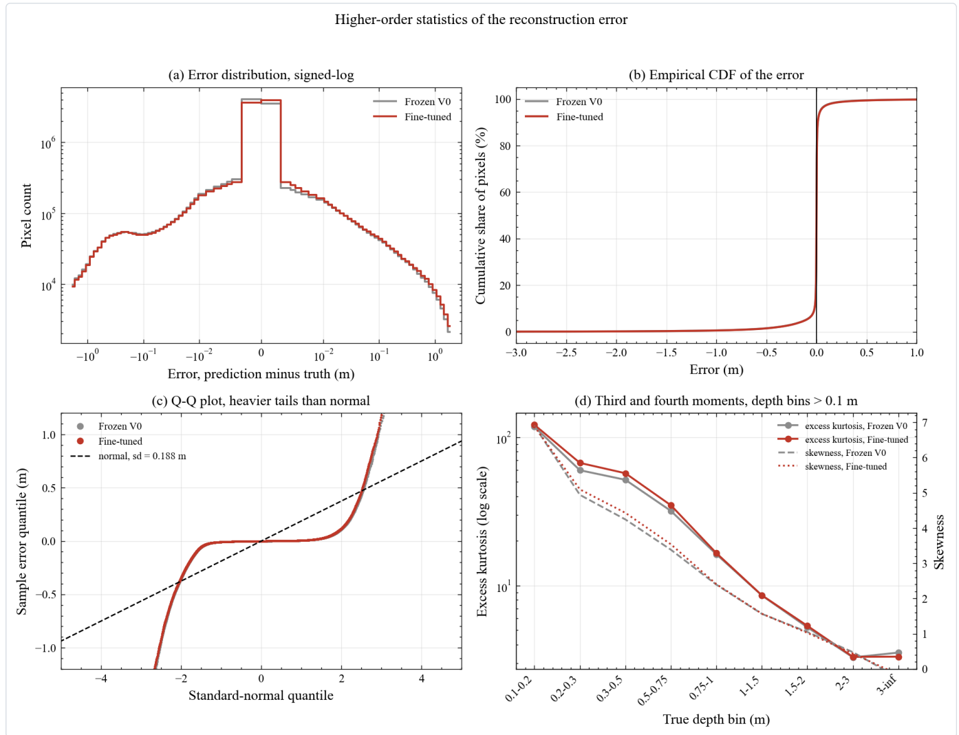
图 49 重构误差的分布与高阶矩。 这一组子图把误差当成一个分布来考察，关注的是它的形状而不只是平均值。(a) 是两个模型误差的频次分布，横轴采用对称对数标度以便同时展示零附近的密集区与两侧的长尾，纵轴为对数标度。(b) 是误差的经验累积分布，横轴是误差取值，纵轴表示误差不超过给定值的像元占比，曲线越陡说明误差越集中，曲线在某一侧拖长说明该侧出现大误差的机会更多。(c) 是分位数对分位数图。它的做法是把实测误差与一个标准差相同的正态分布按同样的累积概率逐点配对，如果误差服从正态分布，所有点就会落在黑色虚线上，散点偏离该线越远说明尾部越重。(d) 是分水深区间的偏度与超额峰度，峰度用对数纵轴，偏度用右侧纵轴，最浅的两个区间因为真值接近零、分布退化，未纳入该子图。读的顺序是先看 (a) 判断整体形状，再看 (b) 定位大误差出现在哪一侧，然后用 (c) 检验尾部是否偏离正态，最后用 (d) 看不同水深上的形状差异。四幅子图给出的阶段性结论是误差分布接近拉普拉斯形状，左尾很厚。两个模型的分布曲线几乎完全重合，说明微调没有改变误差的总体形状，只挪动了少量质量。用正态假设去推断深水误差的置信区间会严重低估风险。
