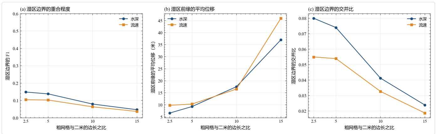
图 22 湿区前缘的重合程度。掩膜一律由水深场给出,阈值取五厘米,水深用事件最大值,流速取峰值水量那一小时的瞬时水深。边界由形态学腐蚀得到,原掩膜减去腐蚀结果就是一圈边界像元。(a)是两圈边界的 F1,(b)是两条前缘线之间的修正豪斯多夫距离,取两个方向里较大的一个,(c)是边界交并比。水深上前缘 F1 从五米的 0.148 降到三十米的 0.046,修正豪斯多夫距离从 6.58 米升到 36.98 米。流速上前缘 F1 更低,五米是 0.104,三十米是 0.036。就本图而言,区域内部的标号一致性远高于前缘线的一致性,四对前缘 F1 最高只有 0.148。五米与十米这一对在区域内部有 0.714 的 V-measure 与 0.891 的平均交并比,边界比较里没有出现同量级的取值,分辨率的损失主要落在湿区轮廓上。
