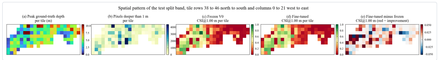
图 39 测试集的空间格局与逐瓦片性能。 这张图回答的是误差长在哪里。五个子图共用同一套网格，横向二十二列自西向东，纵向九行自北向南，每一格是一个四百八十米见方的瓦片。测试集只覆盖完整网格南部的那一条，图中因此只画这一条，完整网格的其余部分不进入本图，那里也没有可评估的淹没像元。(a) 每格的最大真值水深，采用百分位截断以避免个别极值压低对比度。(b) 每格中水深超过一米的像元个数，它是判断该格是否属于深水区的依据。(c) 与 (d) 分别是冻结基线与微调模型在每格上的深水判定指标，取值范围为零到一，数值越高表示该格的深水范围越准确。(e) 是两者的差值，红色表示微调更好，蓝色表示更差。读法是先看 (a) 与 (b) 确定深水在哪里，再把 (c) 与 (d) 对照着看哪里的判定质量差，最后用 (e) 检查改善是否集中在问题最严重的位置。三个层次对应三个问题，也就是水在哪里、哪里判得差、改好了没有。逐瓦片统计给出的结论是改善方向明确而幅度不大。改善超过零点零一个指标单位的瓦片有九十七个，变差超过同样幅度的只有三十个，其余一百一十五个落在两者之间。
