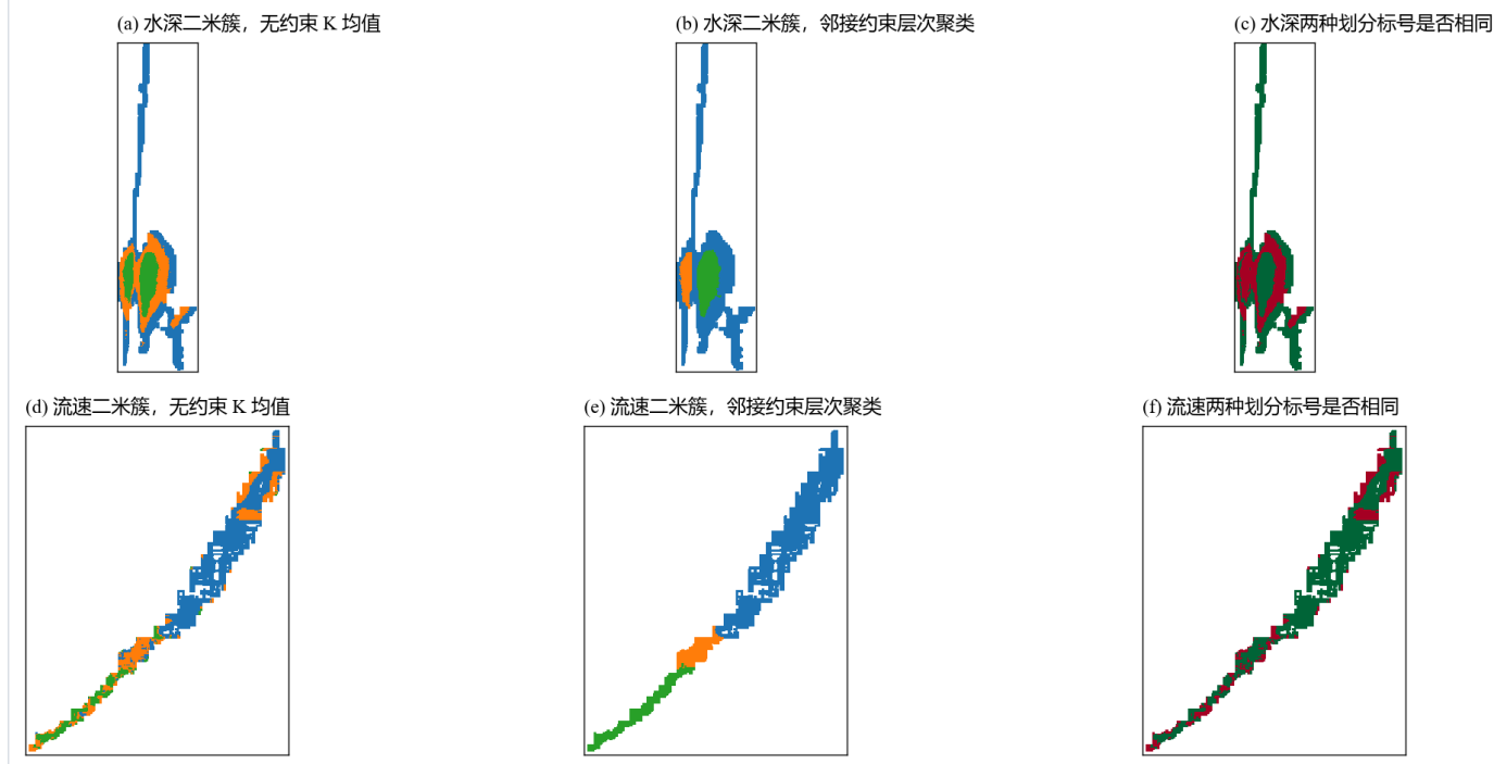
图 27 最大连通核上的区域划分对照。上排三幅是水深，下排三幅是流速，每排的第一幅是无约束 K 均值划分，第二幅是加入上下左右邻接约束的 ward 层次聚类划分，第三幅用红绿两色标出两种划分标号是否相同，绿色表示相同。两幅划分图共用一个簇编号色标，编号按单元的平均对数水深排序。核由湿区做一次三乘三闭运算后取最大连通分量得到，水深核有 23317 个单元，流速核有 5047 个。就本图而言，同一个二米水深场上两种划分的 V-measure 只有 0.468，说明无约束 K 均值给出的簇在空间上是碎的，加约束之后簇才连成片。
