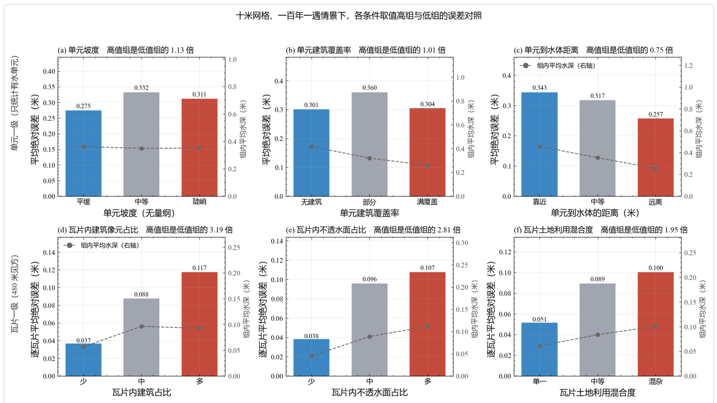
图 12 各条件取值三档之间的误差对照，十米网格。六个子图的横轴都是条件变量的三个取值档，由低到高依次为蓝色、灰色与红色三组柱子，纵轴是平均绝对误差，单位是米，柱顶数字是具体取值。每个子图还配一条灰色虚线，用右侧纵轴读数，表示该组内部的平均水深，单位是米，用来提示各组之间的水深并不相同。上排三个子图是单元一级，只统计有水单元，横轴依次是单元坡度、单元建筑覆盖率与单元到水体的距离，距离的单位是米。下排三个子图是瓦片一级，横轴依次是瓦片内建筑占比、瓦片内不透水面占比与瓦片土地利用混合度。单元建筑覆盖率的三档由二米建筑掩膜按面积加权聚合得到，覆盖率等于零为无建筑，介于零与一之间为部分覆盖，等于一为满覆盖。上排三幅的形状并不一致。坡度一幅的中间档最高，到水体距离一幅随距离单调下降，从靠近水体的 0.343 米降到远离水体的 0.257 米。建筑覆盖率一幅呈中间高两头低，部分覆盖组是 0.360 米，高于无建筑组的 0.301 米与满覆盖组的 0.305 米。下排三幅都呈明显的上升，建筑占比一幅从 0.037 米升到 0.117 米，不透水面一幅从 0.038 米升到 0.108 米，土地利用混合度一幅从 0.051 米升到 0.100 米。再看灰色虚线，上排建筑覆盖率一幅的虚线随横轴下降，说明满覆盖组的平均水深反而浅，从无建筑组的 0.417 米降到满覆盖组的 0.259 米，部分覆盖组居中在 0.320 米。既然误差的主要外部条件集中在建成状况上，校正模型就应当把建筑与地类信息当作主要输入。
