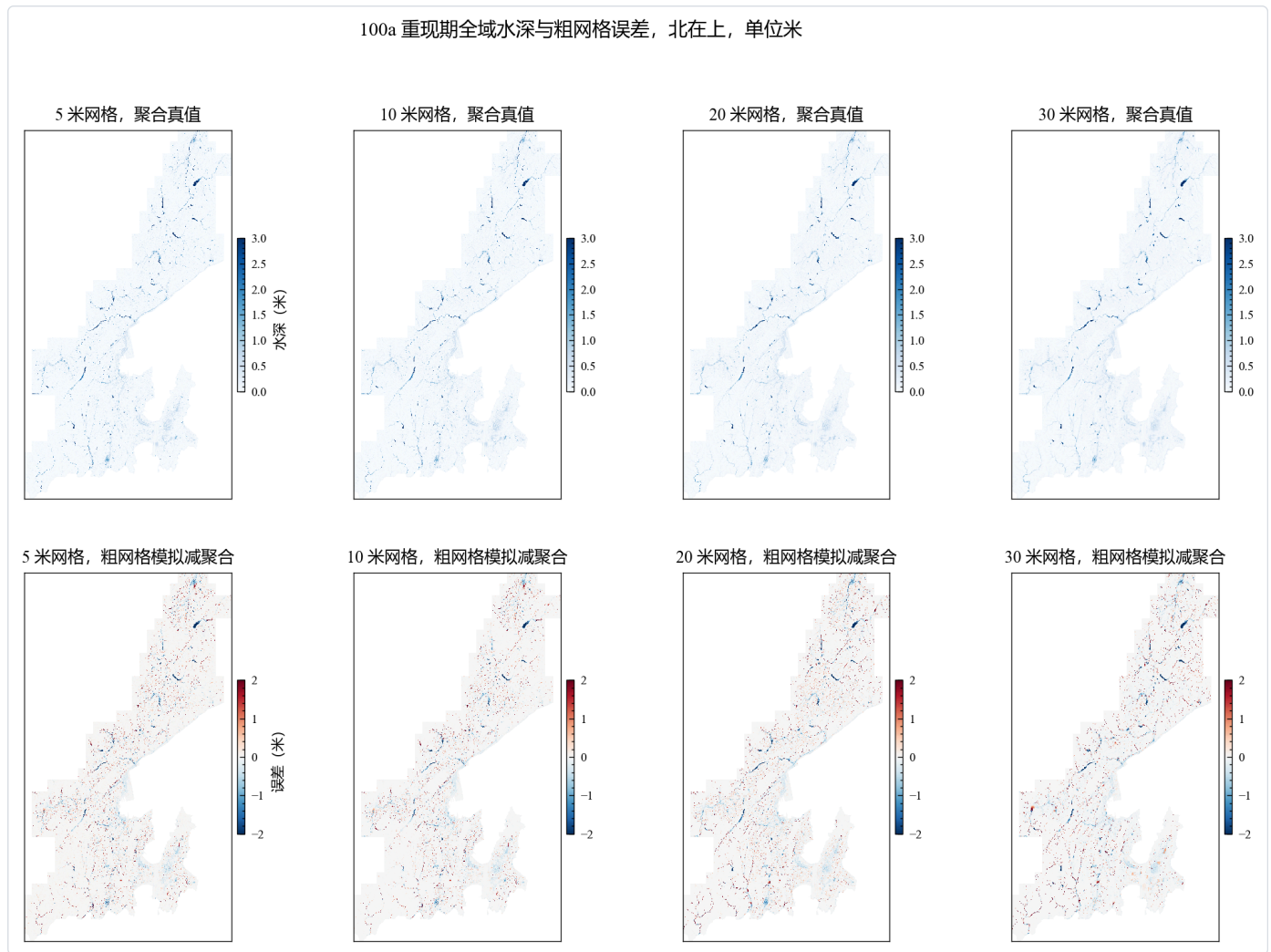
图 9 一百年一遇情景下全域水深与粗网格误差的空间分布。图分上下两排，每排四幅，自左向右依次是五米、十米、二十米与三十米网格。上排是聚合后的二米真值的水深场，颜色由浅蓝到深蓝表示水深由小到大，色标范围固定在零到三米，超出三米的部分按最深色显示，每一幅配一条独立色标，单位是米。纵横坐标是格网行列号，北在上方，为了便于印刷未标注刻度数值。可以读出淹水集中在中部与南部的河谷与低洼街区，随网格变粗，同一片水域的颜色变得更均匀，细密的支流消失。下排是图 4 所说第三笔账的误差场，也就是粗网格模拟值减聚合真值，颜色用发散色标，红表示粗网格算深了，蓝表示算浅了，色标范围对称固定在负二米到正二米，单位是米。可以读出误差不是逐点随机的，它沿河道与地形陡变带成片出现。五米网格上的红色斑块最碎，随网格变粗逐渐连成大片，三十米网格上的蓝色条带几乎完整覆盖主要河道。把上下两排对照，可以确认蓝色条带的位置与上排的深蓝色河道位置重合，说明欠估发生在水最深的地方。
