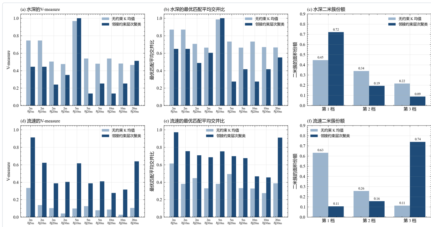
图 28 连通核上的无约束与邻接约束划分对比。上排是水深，下排是流速。左列是十个分辨率组合的 V-measure，中列是最优匹配平均交并比，两列的横轴都是分辨率组合，蓝色柱为无约束，深蓝色柱为邻接约束。右列是二米划分三个簇的面积份额，横轴是簇编号，两组柱并列。就本图而言，水深处上五米与十米的 V-measure 由 0.969 升到 1.000，十米与二十米由 0.538 降到 0.137。流速上五米与十米由 0.098 升到 0.617，约束把水深最大一簇的份额从 0.446 抬到 0.721。
