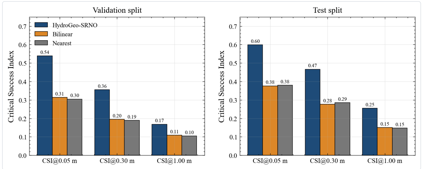
图 27 模型与两种传统插值方法的指标对比。左子图 (a) 是验证集，右子图 (b) 是测试集，两个子图的结构完全一致，可以左右对照着读。每组内三根柱子依次是模型、双线性插值与最近邻插值，柱子的颜色区分方法。纵轴是临界成功指数，取值在零到一之间，越高越好。横轴是三档判定阈值，从左到右依次升高，阈值越高表示判定积水的门槛越严。柱顶数字是具体取值。这张图的作用是给出一个背景基线，回答学习模型相比不做学习的插值方法到底好多少，好在哪个阈值上，以及这个优势是否在不同数据集合上稳定。
