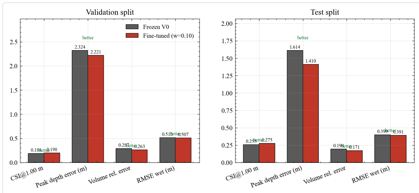
图 48 冻结基线与微调模型的逐项对比。这张图的用意是把改动前后放在一起，让读者一眼看清哪几项动了、哪几项没动。左子图 (a) 是验证集，右子图 (b) 是测试集，两个子图的结构完全一致，可以左右对照。每组内左柱是冻结基线，也就是微调之前的模型，右柱是微调之后的模型。四个指标依次是深水指标、峰值深度误差、体积相对误差与湿区均方根误差。读这张图要先分清方向，深水指标越大越好，后三项越小越好，因此后三项的柱高降低才代表改善。柱间的文字标出该项是变好还是变差，不确定方向时可以依赖这个标注。两个子图都给出是为了确认改善能在独立区域上复现，这一点在第 5.9 节有专门讨论。四组柱子读下来的结论只有一句，改善集中在与深水直接相关的三项上。深水指标从 0.184 升到 0.198，峰值深度误差从 2.32 米降到 2.22 米，体积误差从 0.287 降到 0.263，测试集上的降幅比验证集更大，说明修正具有普遍性，不是对验证集地理特点的适配。
