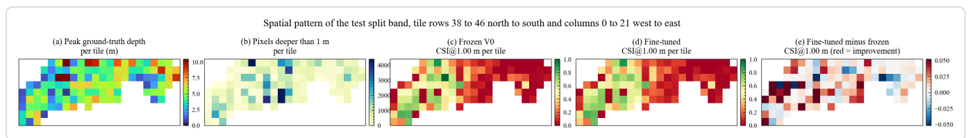
图 16 测试集的空间格局与逐瓦片性能。五个子图共用同一套网格，横向二十二列自西向东，纵向九行自北向南，每一格是一个四百八十米见方的瓦片，图中只画测试集实际覆盖的那一条。(a) 与 (b) 确定深水在哪里，(c) 与 (d) 是冻结基线与微调模型的深水判定指标，(e) 是两者的差值。改善超过 0.01 个指标单位的瓦片有 97 个，变差超过同样幅度的只有 30 个，其余 115 个落在两者之间。
