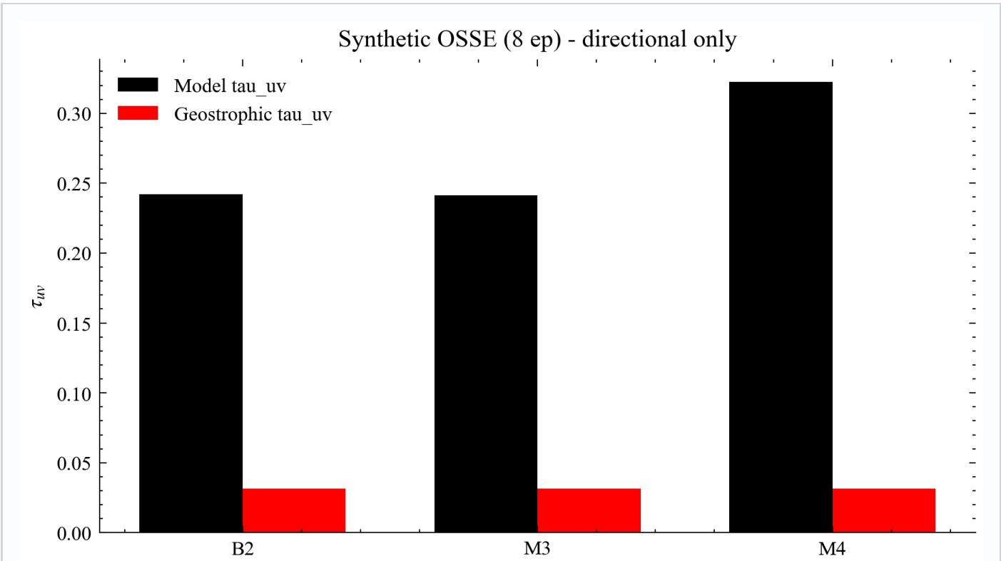
图1. 合成 OSSE 消融：表面流场解释方差 \tau_{uv}
