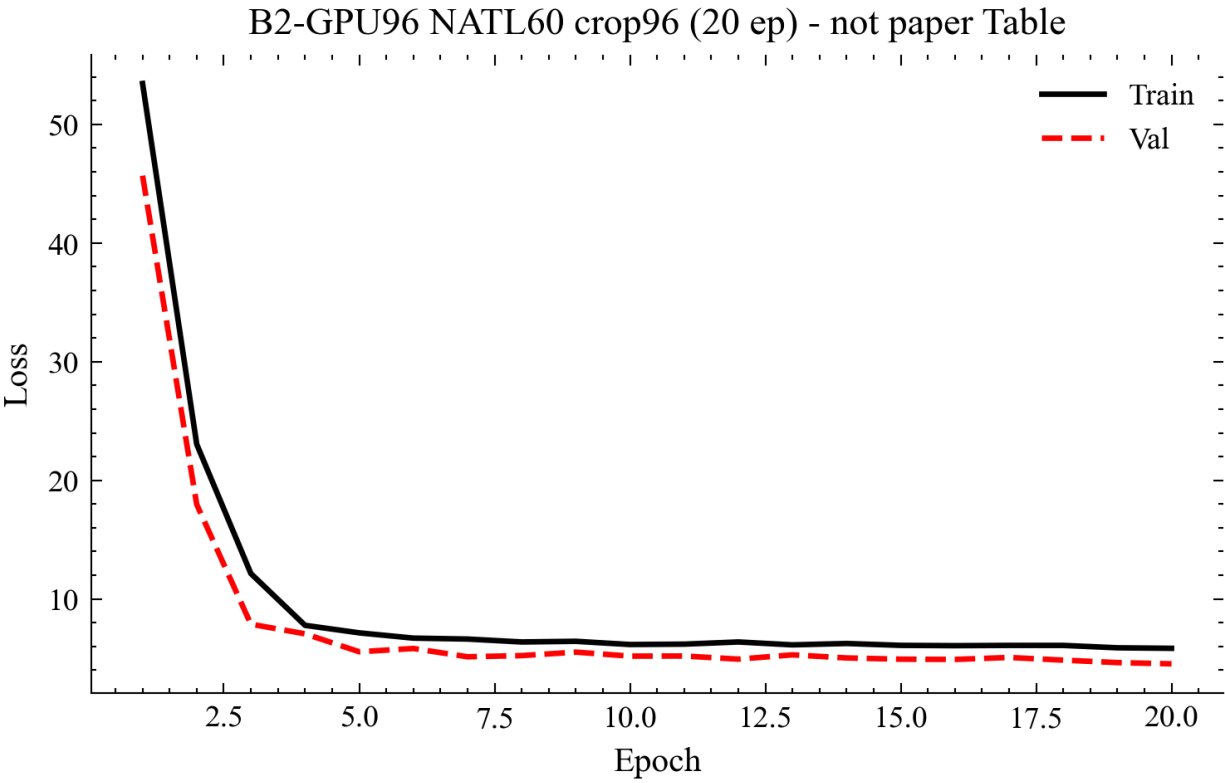
图5. B2-GPU96 训练/验证损失曲线
