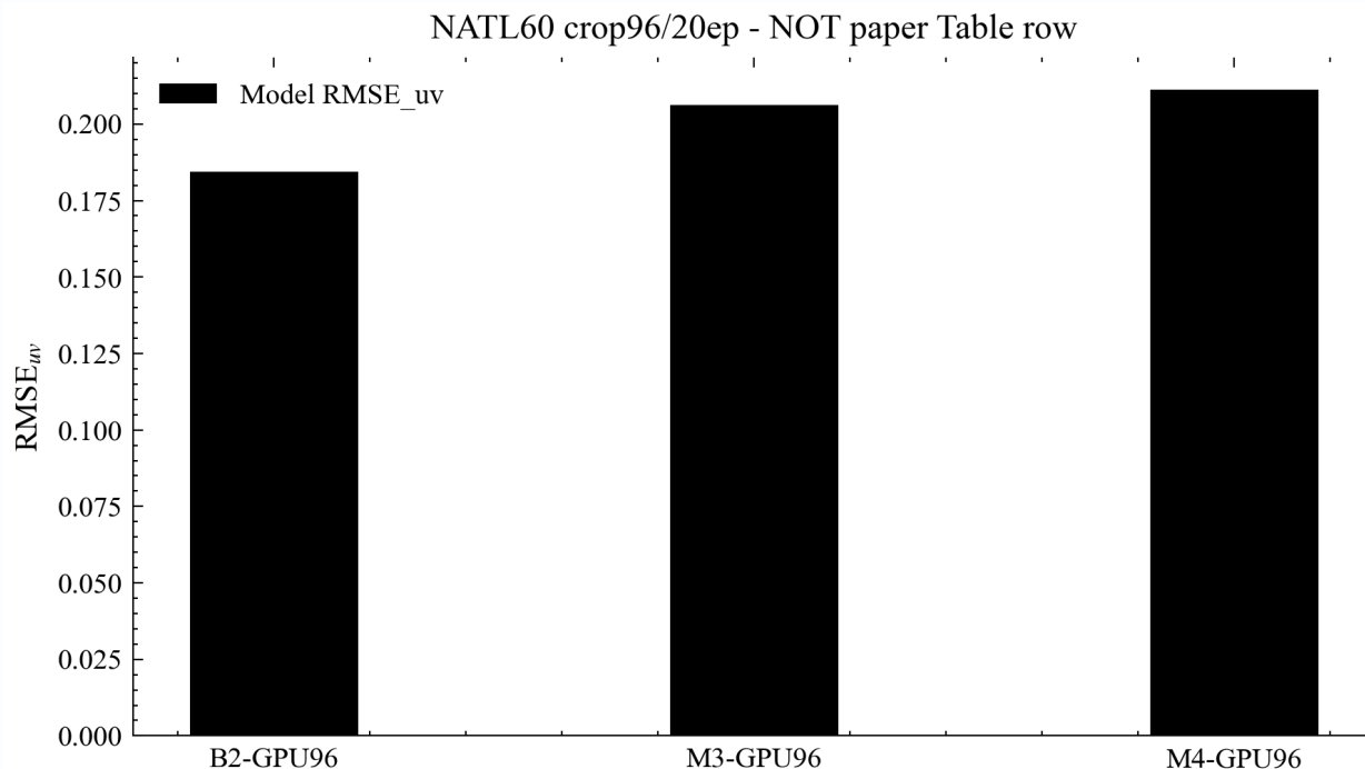
图4. NATL60 GPU96（crop96/20ep）RMSE uv
