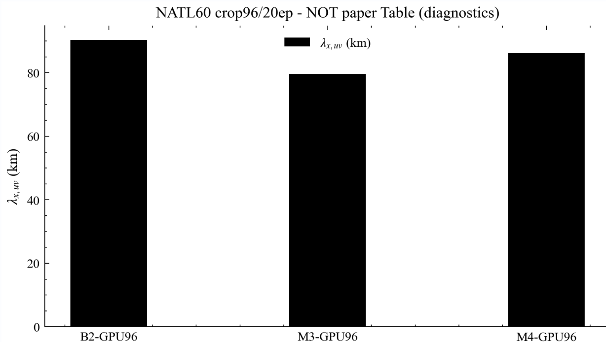
图9. NATL60 GPU96 (crop96/20ep) \lambda_{x,uv} 诊断
