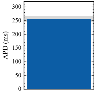
0D APD
