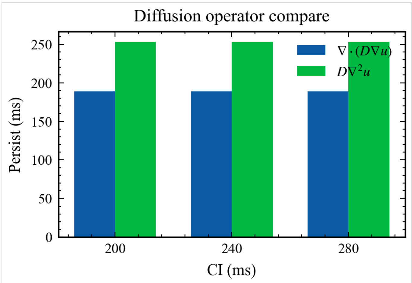
图4. 扩散算子对照： \nabla \cdot (D \nabla u) 与 D \nabla^2 u 的激活持续
