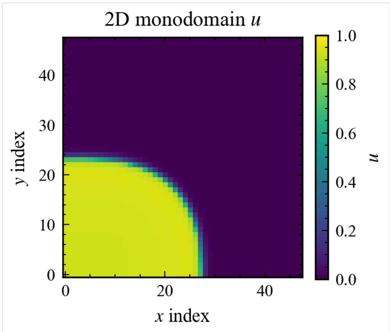
图注：修正 MS、无纤维化短时程仿真终态 u 场（烟雾测试，非折返证据）。
