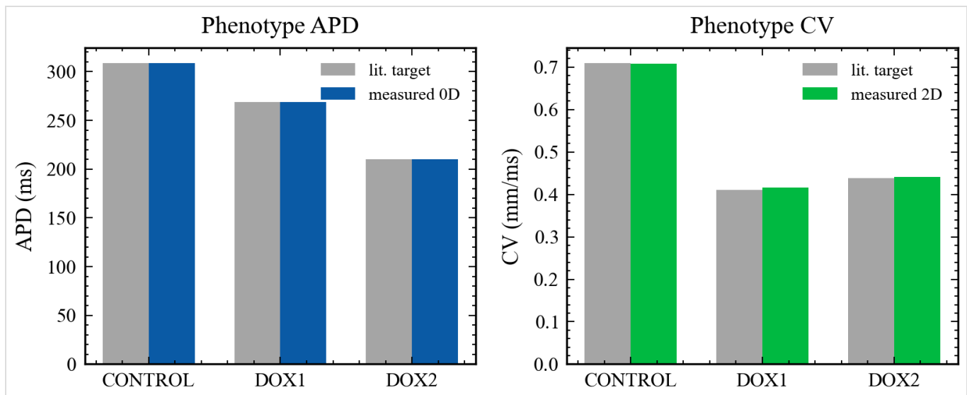
图4. CONTROL/DOX1/DOX2 表型标定：文献目标 vs 本机实测
