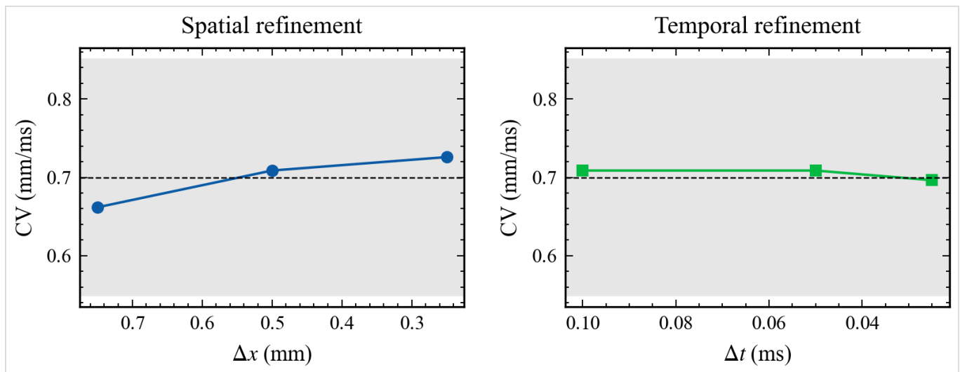
图3. 均匀组织 CV 的空间/时间收敛
