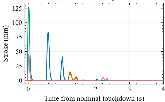
(d) Platform response
