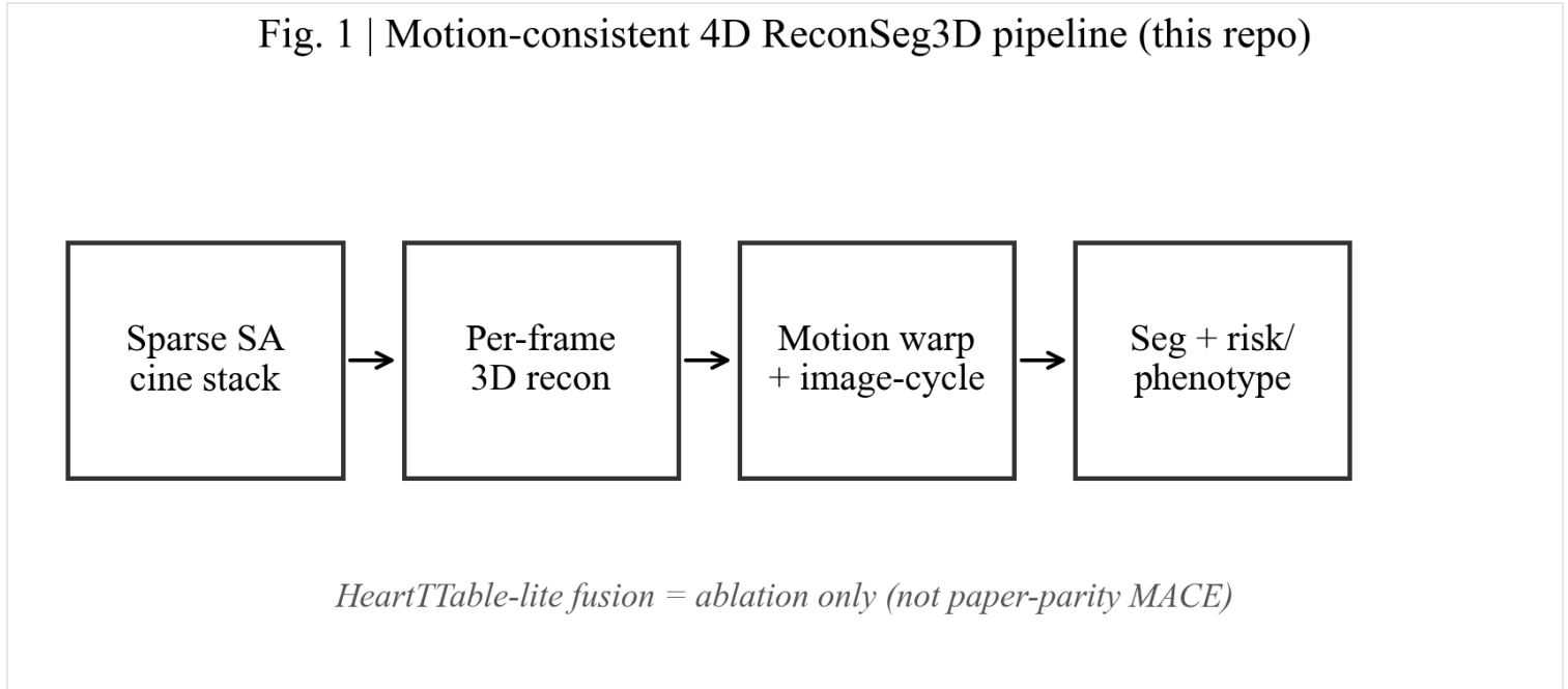
图1 运动一致四维重建-分割流水线示意
