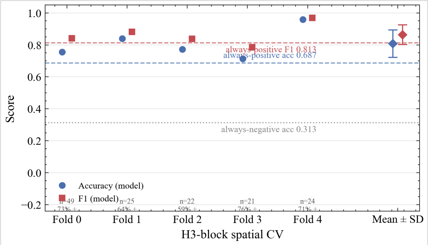
图 4 · Figure 4 — 空间 H3 块 CV 各折 Accuracy 与 F1（SciencePlots + Times New Roman）。 如何读：横轴为折号 + Mean±SD，纵轴为 0–1 分数；成对标记点表示同一折的 Accuracy/F1，末位为 Mean±SD 误差棒；虚线/点线标记恒判正/恒判负常量类基线。 意义：展示评价协议的折间稳定性，而非单一乐观分数。 结论：多数折 Accuracy≈0.71–0.84，Fold4（n=24）更高；与表 3 均值一致。样本仍是 Lower Manhattan smoke。
