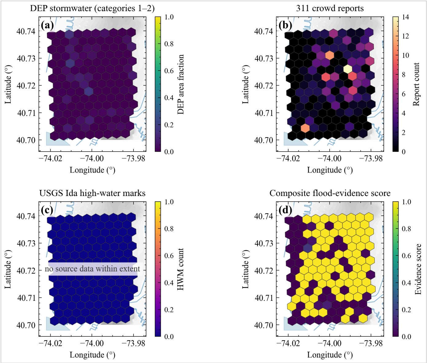
图 3 · Figure 3 — 源证据分解图：Lower Manhattan (n=141 R9) 四面板同支撑（SciencePlots + Times New Roman）。
