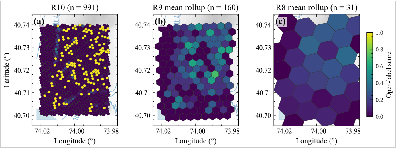
图 5 · Figure 5 — 多分辨率开放证据分空间并排图：(a) R10（n=991）；(b) R9 mean 上卷（n=160）；(c) R8 mean 上卷（n=31），共享 0–1 viridis 色标（SciencePlots + TNR）。 如何读：三面板同一地理足迹，从细到粗看局部热点如何在均值上卷后平滑；颜色只表达开放证据分（0–
