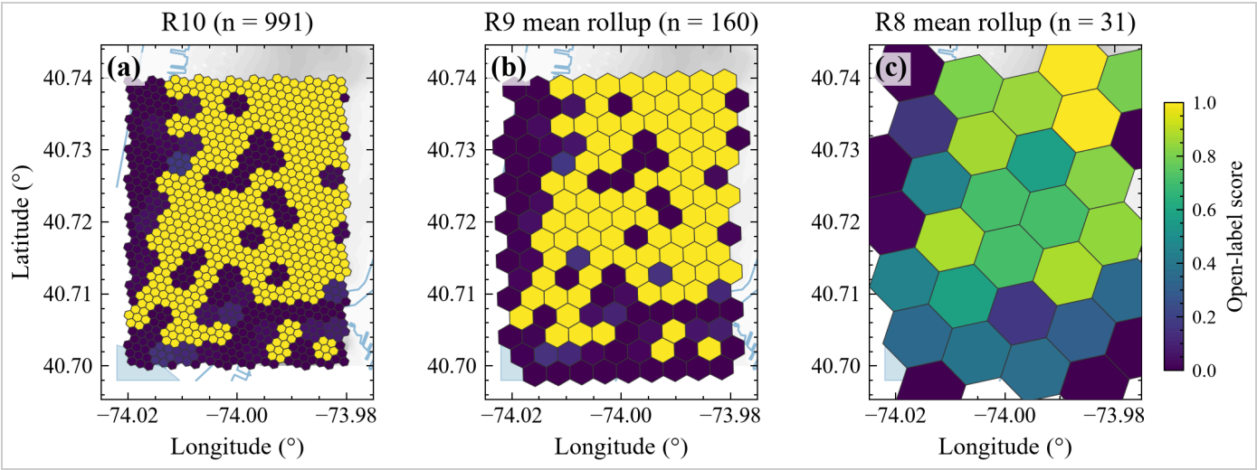
图 4 · Figure 4 — 多分辨率开放标签分空间并排图：(a) R10 (n=991)；(b) R9 mean 上卷 (n=160)；(c) R8 mean 上卷 (n=31)，共享 0–1 viridis 色标 (SciencePlots + TNR)。
