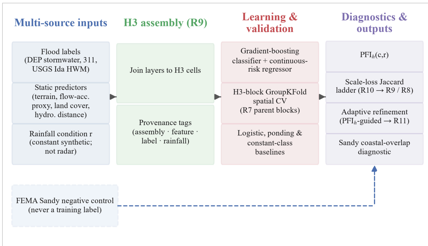
图 1 · Figure 1 — 开放标签 H3 雨洪学习协议的概念工作流（SciencePlots + Times New Roman）。
