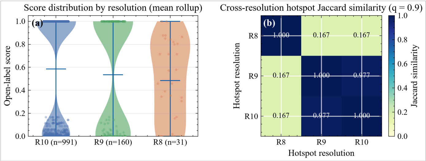
图 5 · Figure 5 — 分辨率效应：(a) 开放标签分在 R10/R9/R8 的分布压缩；(b) Jaccard 热点持久性矩阵（SciencePlots + TNR）。 如何读：(a) 三条小提琴由宽双峰压缩为窄带；(b) 非对角项远离对角线衰减：J(R10,R9)=0.977、J(R10,R8)=0.167、J(R9,R8)=0.167。 意义：把尺度损失从阶梯表扩展为「分布压缩 + 集合持久性」两种互补统计视图，对齐参考论文 Fig 5 类型。 结论：数值与表 3 完全一致；粗化同时压缩分布并瓦解热点持久性。
