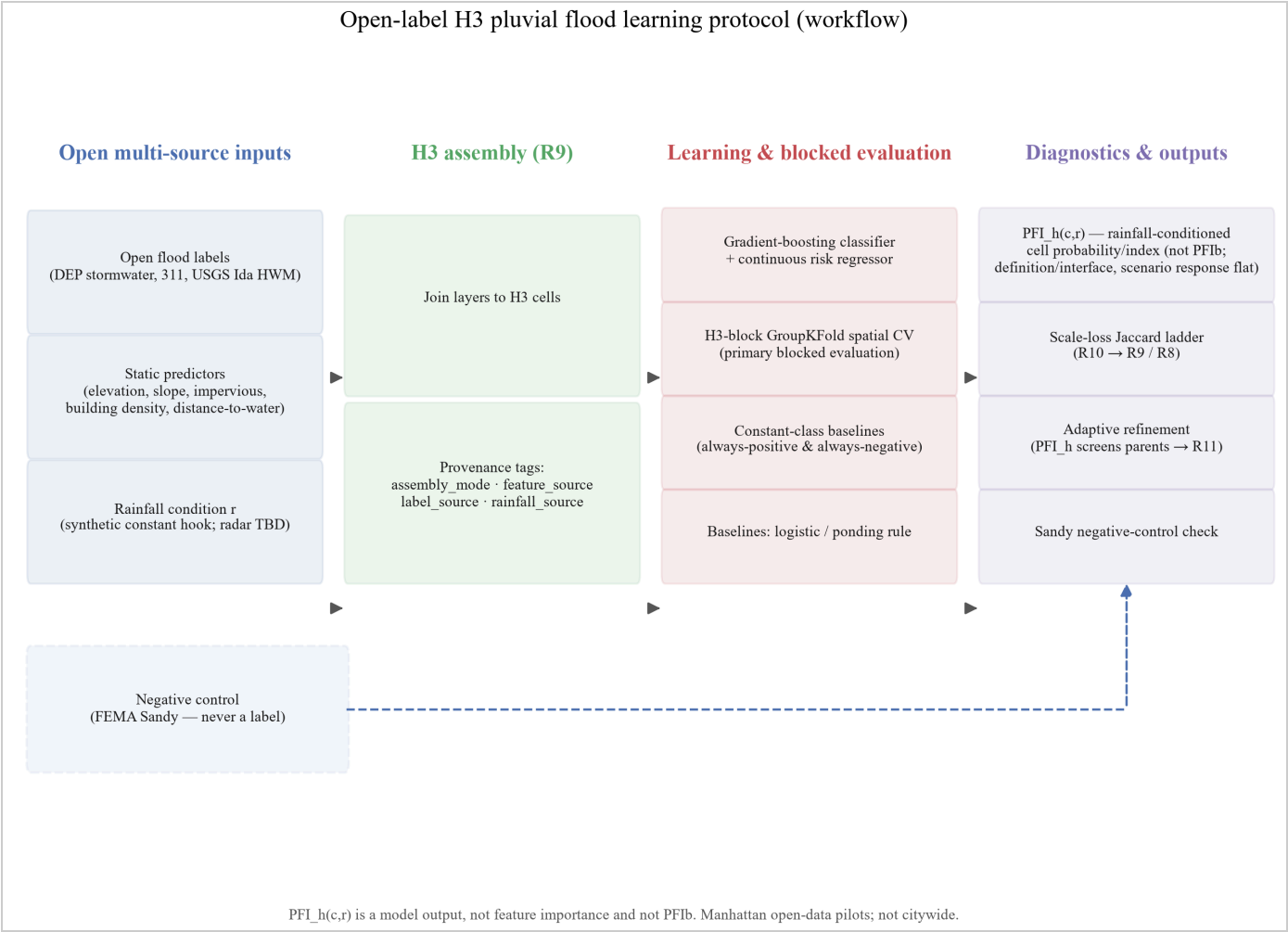
图 1 · Figure 1 — 开放标签 H3 雨洪学习协议的概念 workflow（SciencePlots + Times New Roman）。 如何读：从左到右四列——(1) 开放多源输入；(2) H3 组装（R9 + provenance 标签）；(3) 学习与分块评价（GBM + H3 块 GroupKFold 空间 CV + 常量类基线恒判正/恒判负）；(4) 诊断与输出（PFI h(c,r) 、Jaccard 阶梯、自适应加密、Sandy 负对照，其中 Sandy 为虚线旁路、绕过学习框）。 意义：一张图讲清整条协议与「证据—边界」纪律，对应手稿 Methods。 结论：PFI h(c,r) 是模型输出，不是特征重要性，也不是 PFIb；当前情景响应平坦；证据仅限 Manhattan 开放数据试点，非全市。
