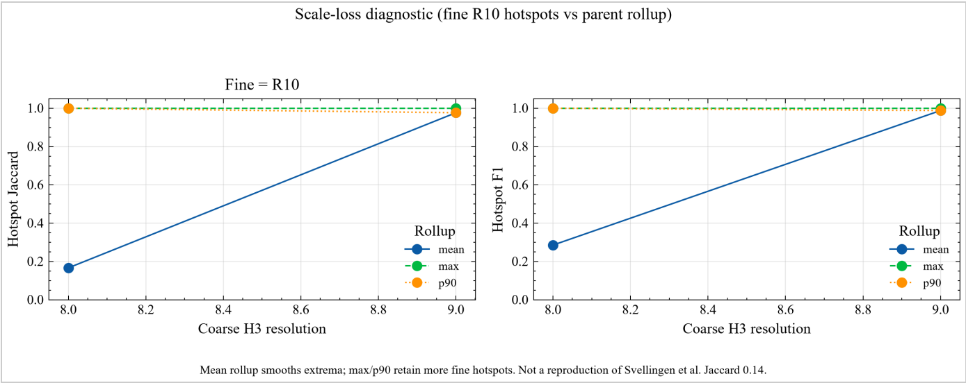
图 3 · Figure 3 — 开放标签热点 Jaccard/F1 随粗分辨率变化（SciencePlots + TNR）。
