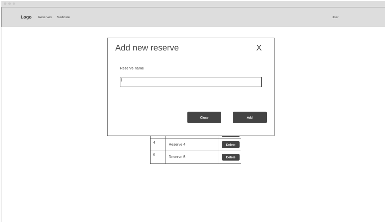
6 pav. Rezervo pridėjimo modalo wireframe
