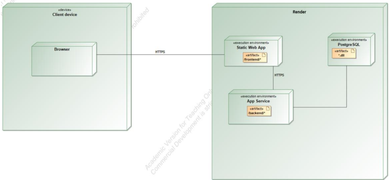
1 pav. Diegimo diagrama
