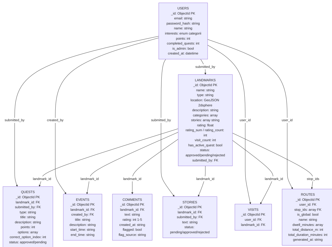
Figura 7: Modelul complet de date al aplicației CultureQuest: colecțiile MongoDB, câmpurile principale și relațiile dintre ele.
