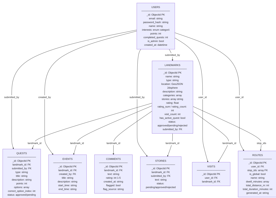
Figura 4: Modelul complet de date al aplicației CultureQuest: colecțiile MongoDB, câmpurile principale și relațiile dintre ele.
