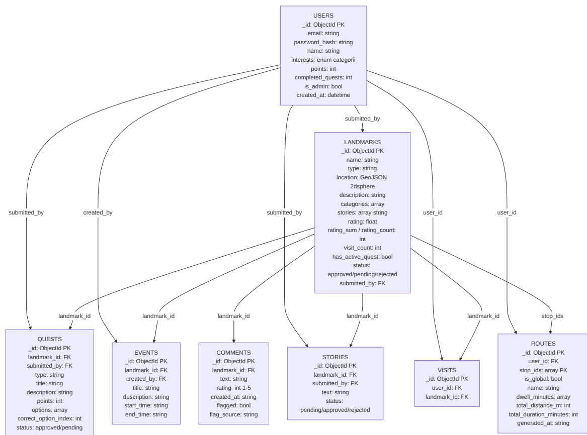
Figura 5: Modelul complet de date al aplicației CultureQuest: colecțiile MongoDB, câmpurile principale și relațiile dintre ele.
