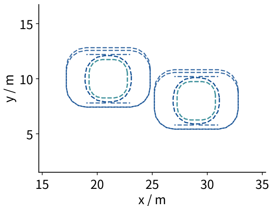
(a) B: 两台风机的水平作业意图
