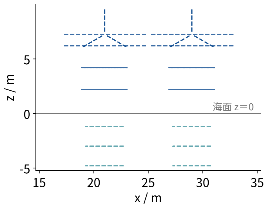
(b) B: 水上高度与基础深度
