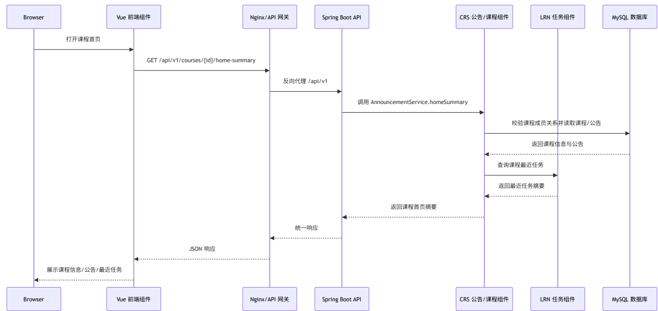
图 2-14 课程首页摘要组件顺序图
