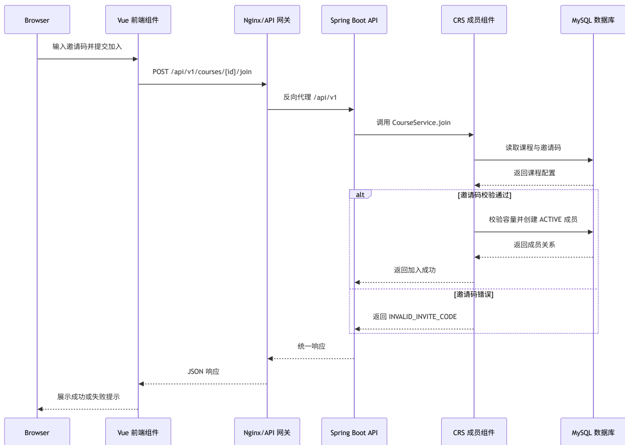
图 2-10 邀请码加入课程组件顺序图
