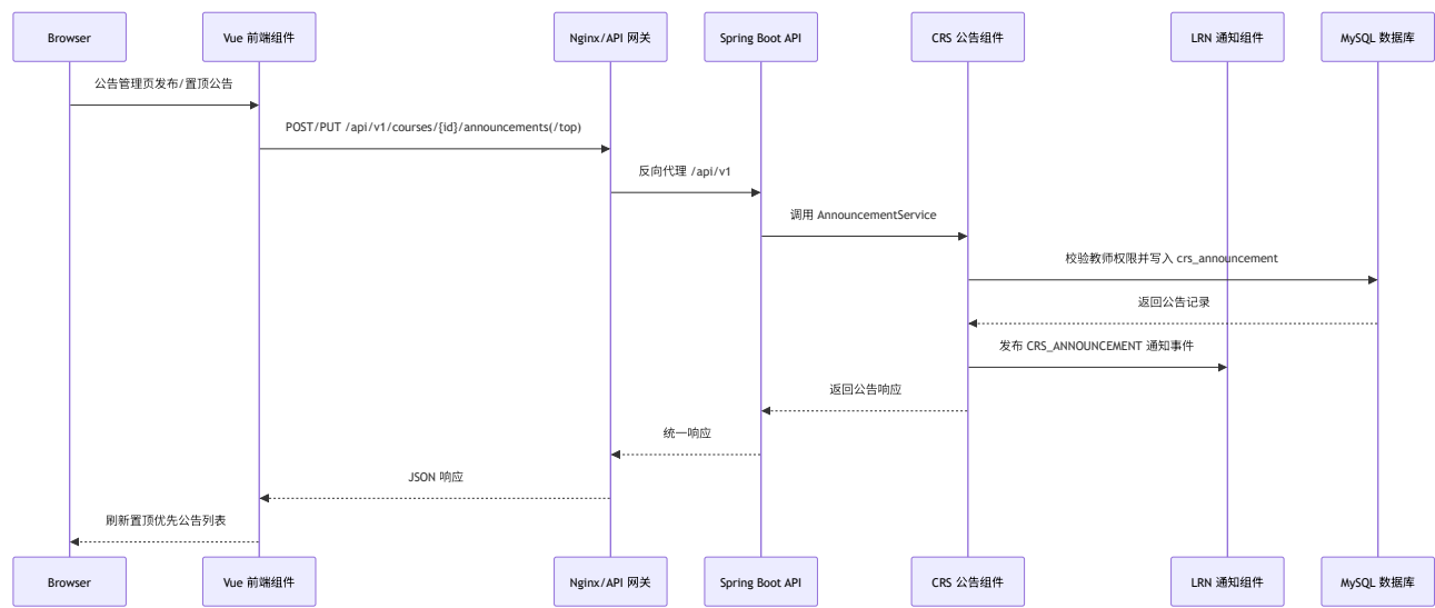
图 2-13 公告发布与置顶组件顺序图
