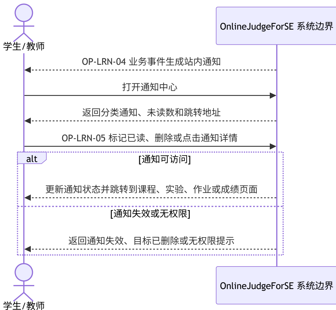
图 4-16 通知反馈系统顺序图
