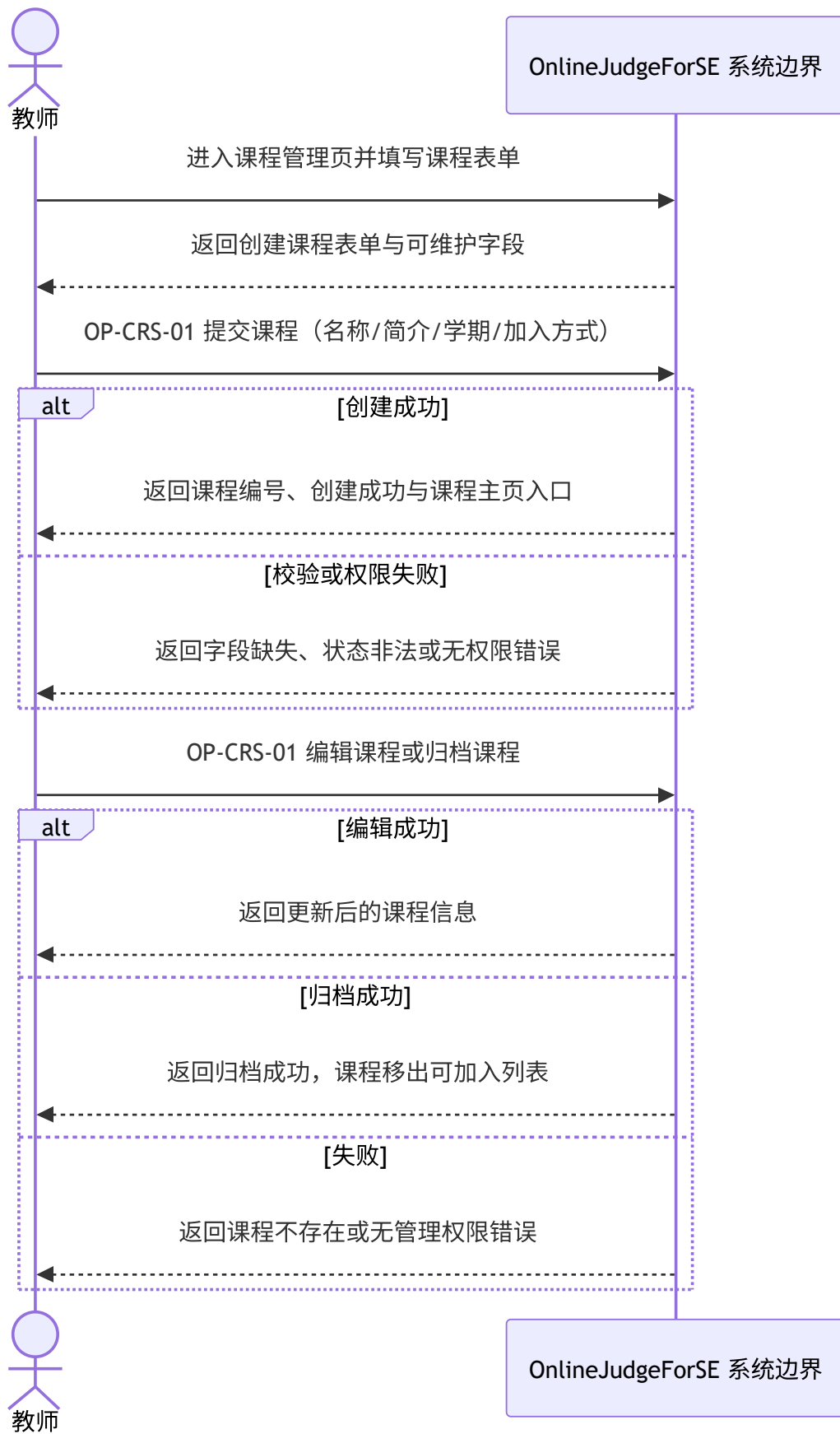
图 4-38 课程创建与维护系统顺序图
