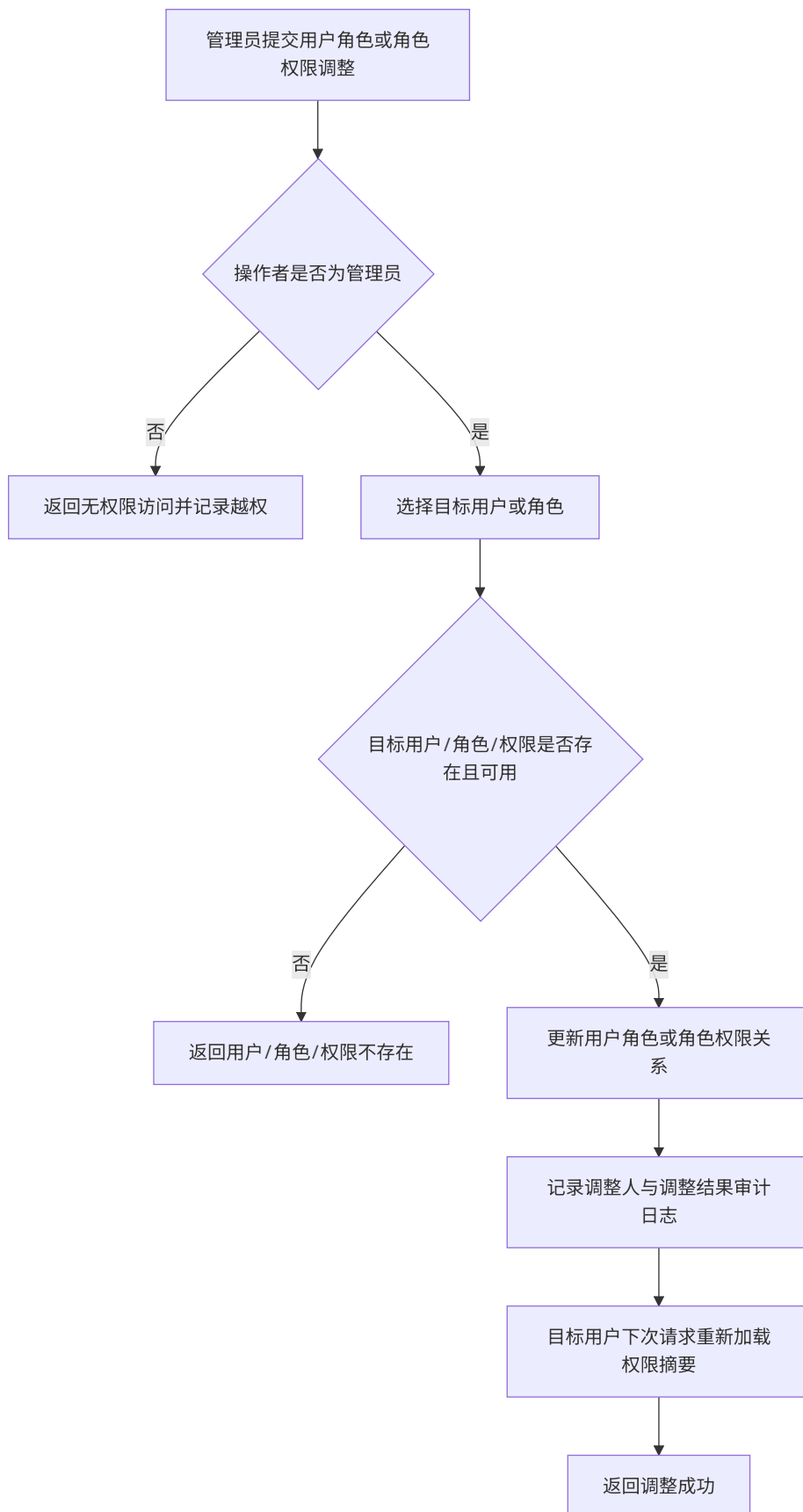
图 4-34 角色权限调整活动图
