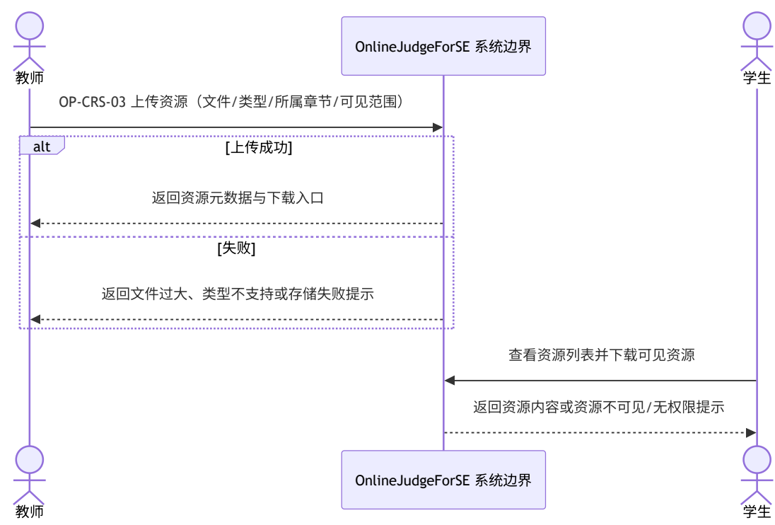
图 4-42 资源上传与下载系统顺序图
