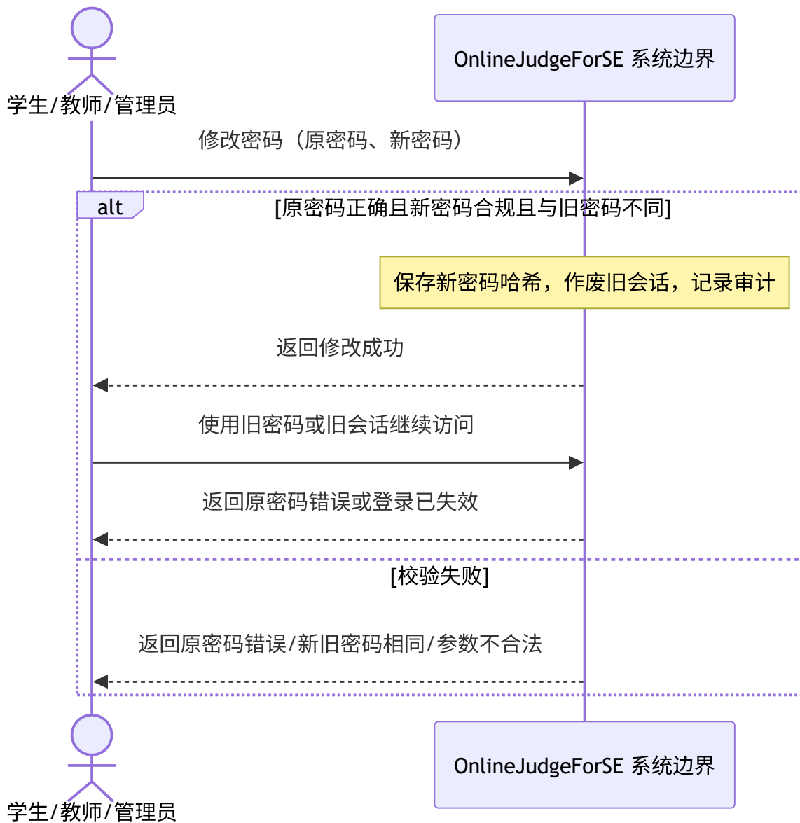
图 4-25 修改密码系统顺序图
