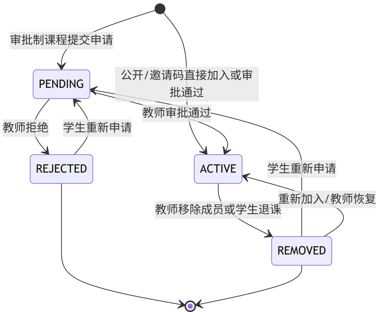
图 4-45 课程成员状态机（公开加入视角）
