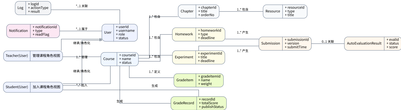
图 5-2 核心对象结构图
