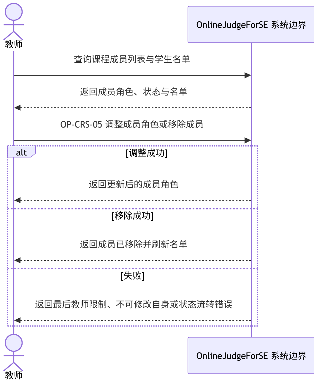
图 4-50 成员管理系统顺序图
