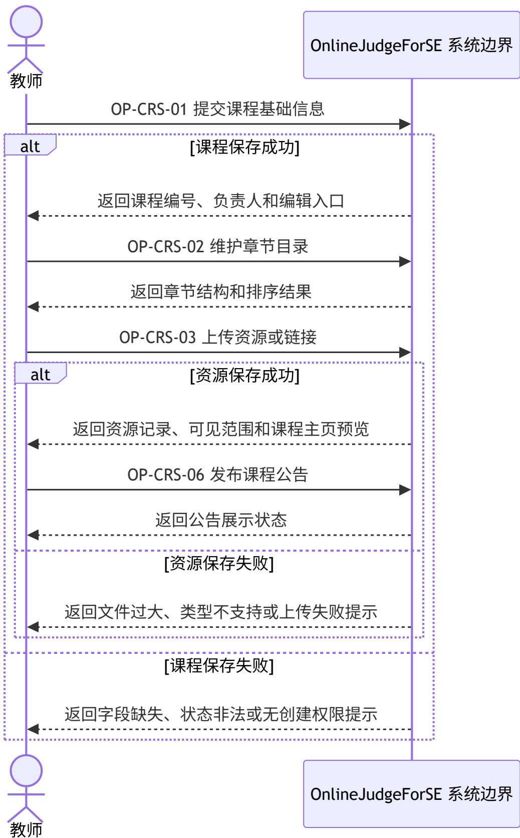
图 4-17 课程创建与资源维护系统顺序图
