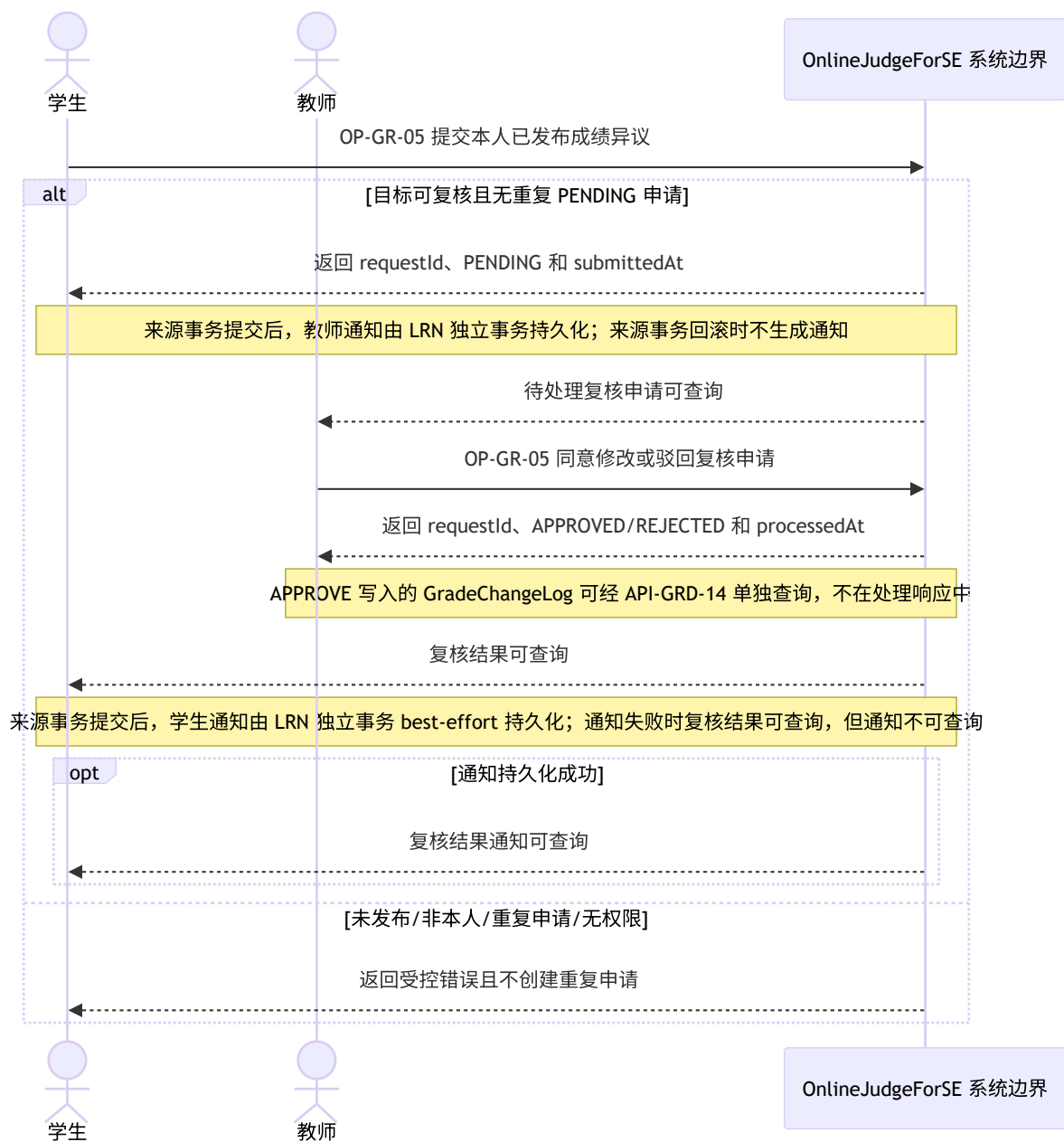
图 4-58 成绩异议复核系统顺序图
