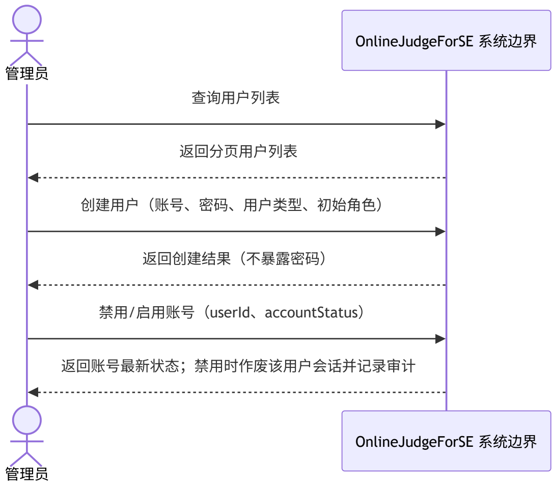
图 4-26 管理员用户与账号状态管理系统顺序图
