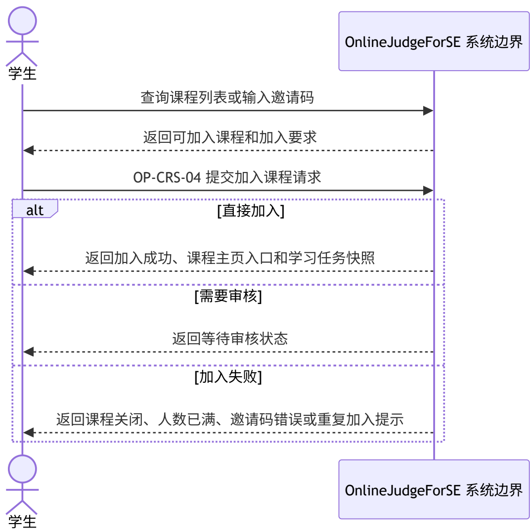
图 4-12 课程加入系统顺序图
