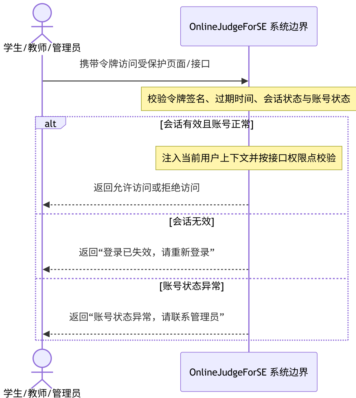
图 4-23 持续鉴权与当前用户上下文系统顺序图
