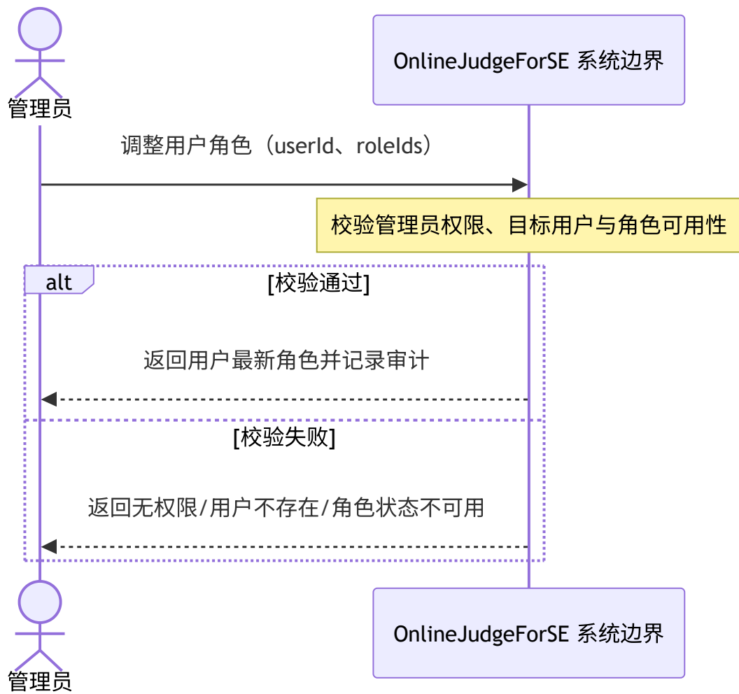
图 4-27 用户角色分配系统顺序图
