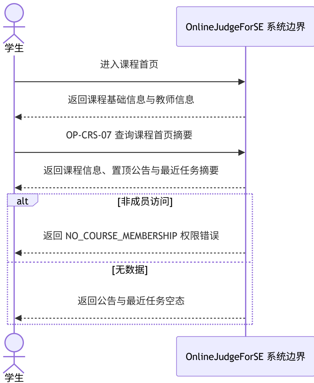
图 4-54 课程首页摘要系统顺序图
