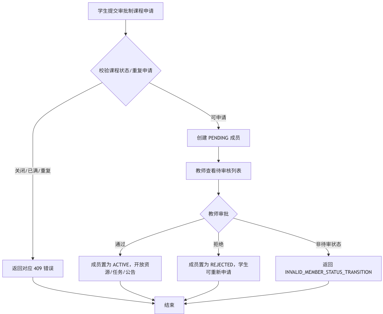
图 4-49 审批加入课程活动图
