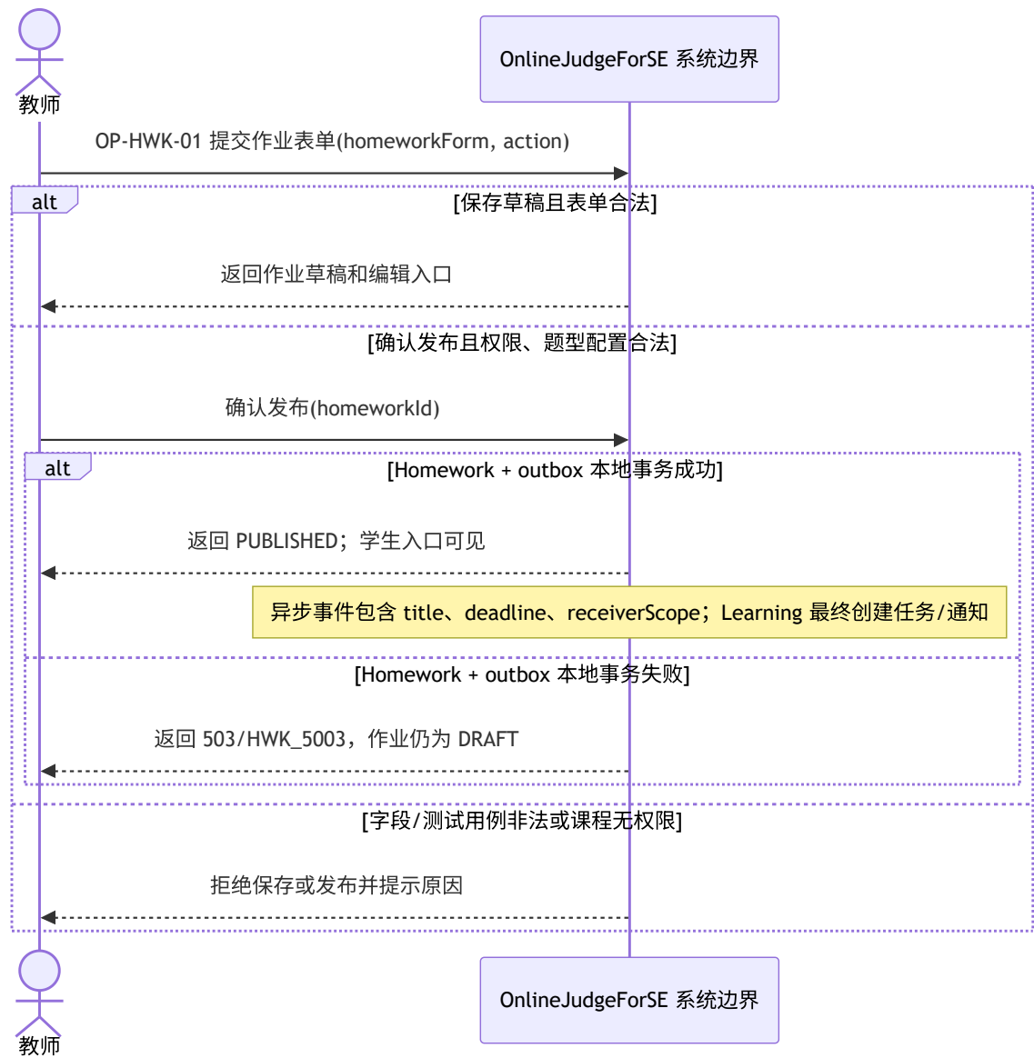
图 4-14B 教师创建并发布作业系统顺序图
