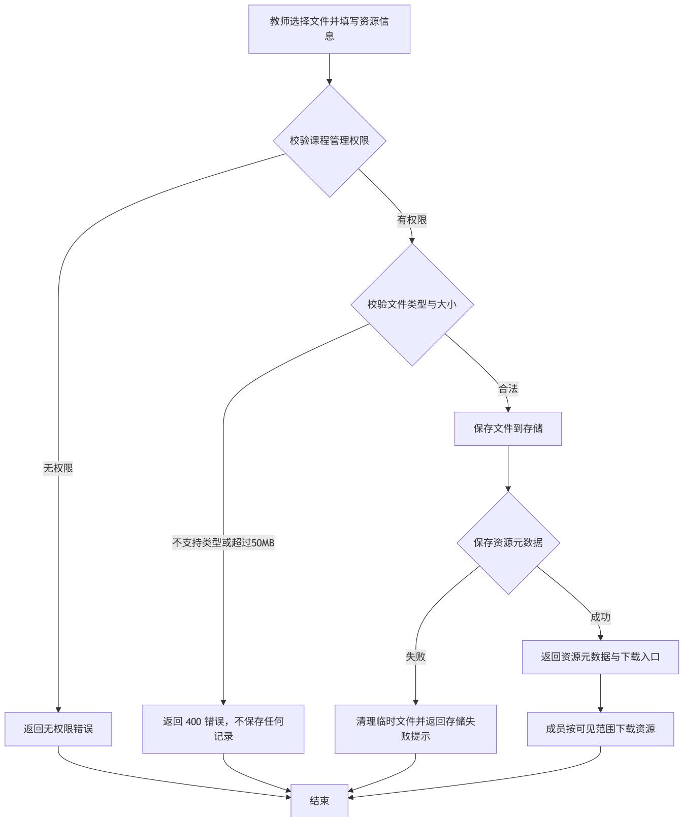
图 4-43 资源上传活动图（含失败回滚分支）
