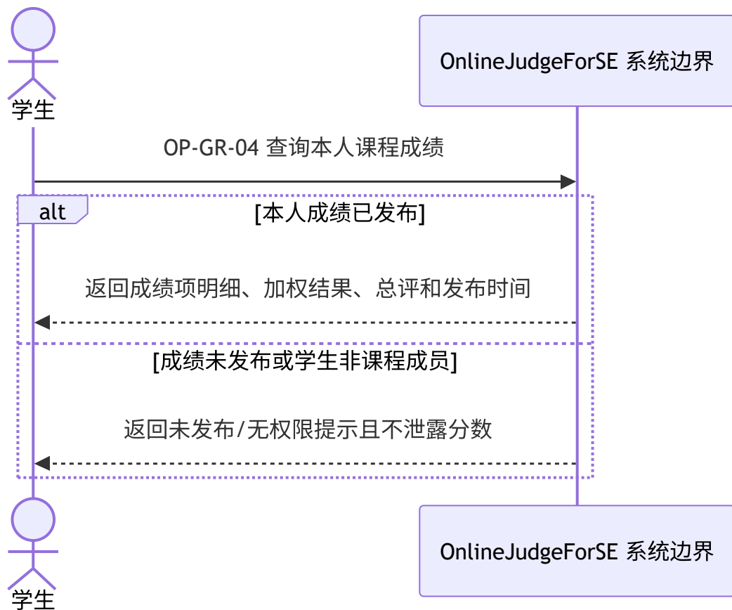
图 4-57 学生成绩查询系统顺序图
