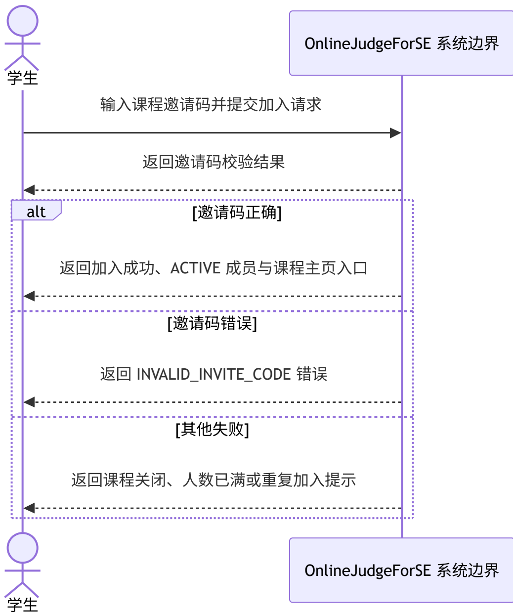
图 4-46 邀请码加入课程系统顺序图
