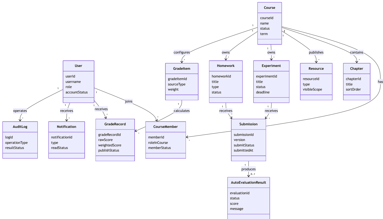
图 5-3 核心概念类图
