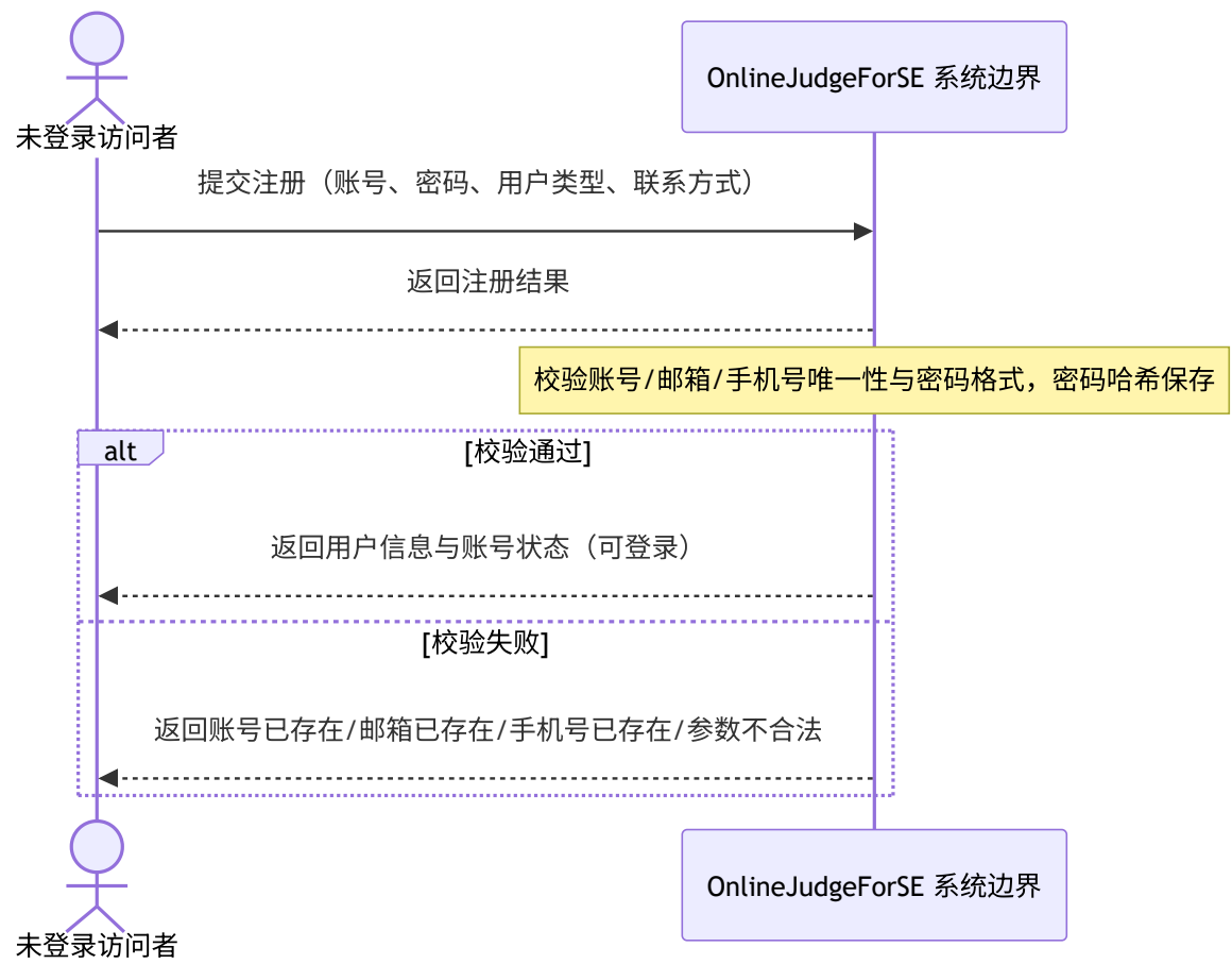
图 4-20 学生自助注册系统顺序图
