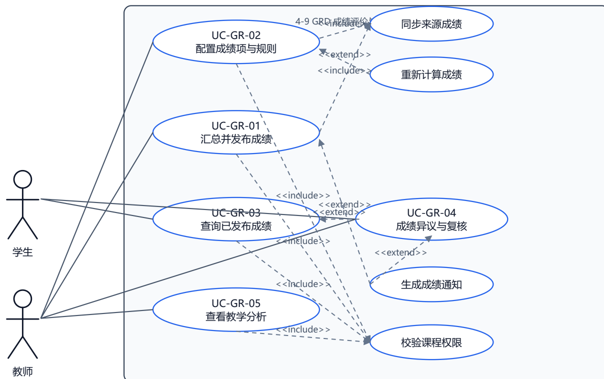
图 4-9 GRD 成绩评价与教学分析用例图
