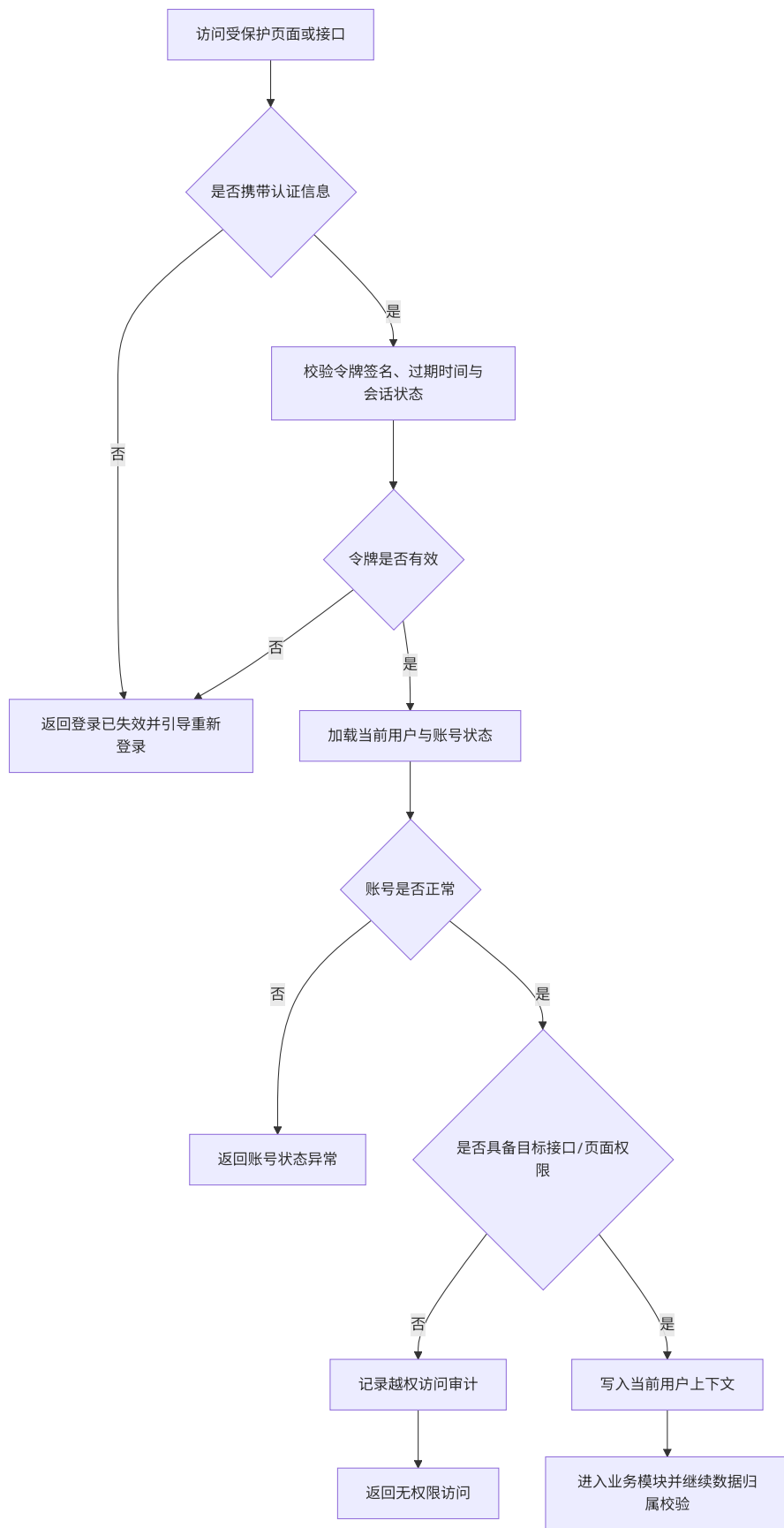
图 4-35 鉴权与越权拦截活动图
