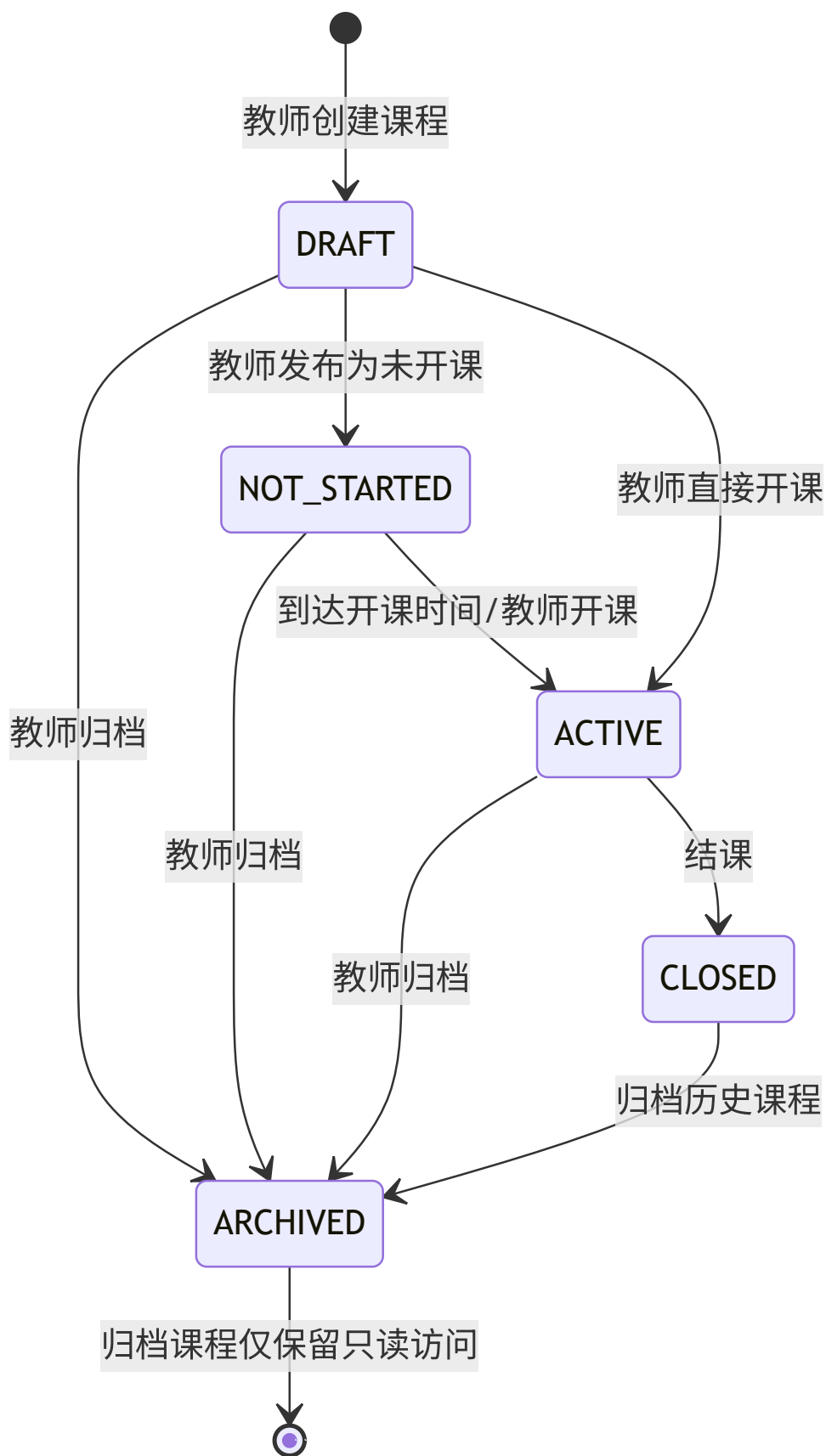
图 4-39 课程状态图 (草稿/未开课/进行中/结课/归档)
