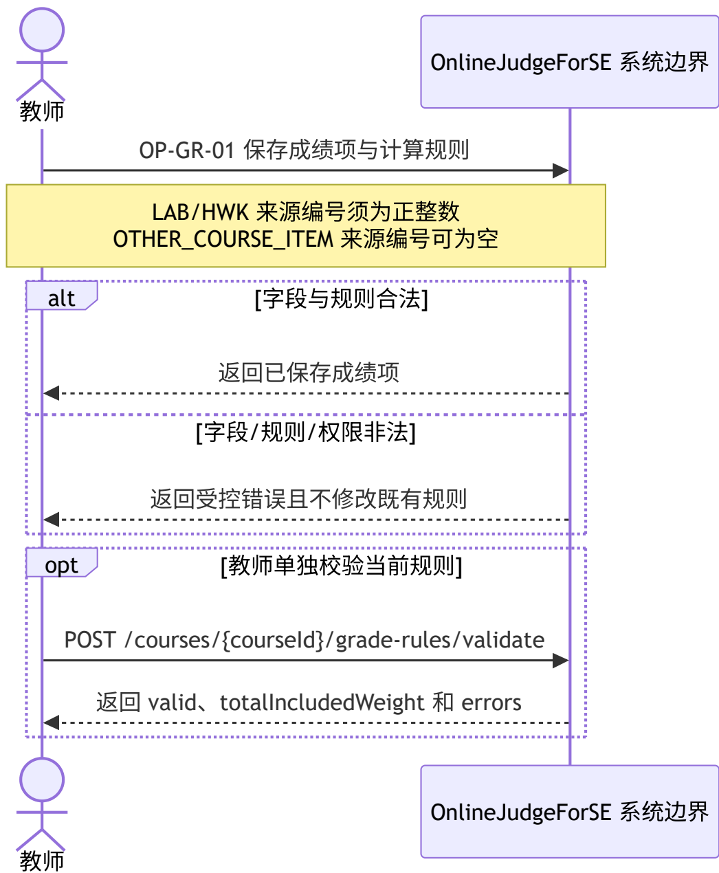
图 4-56 成绩项配置系统顺序图
