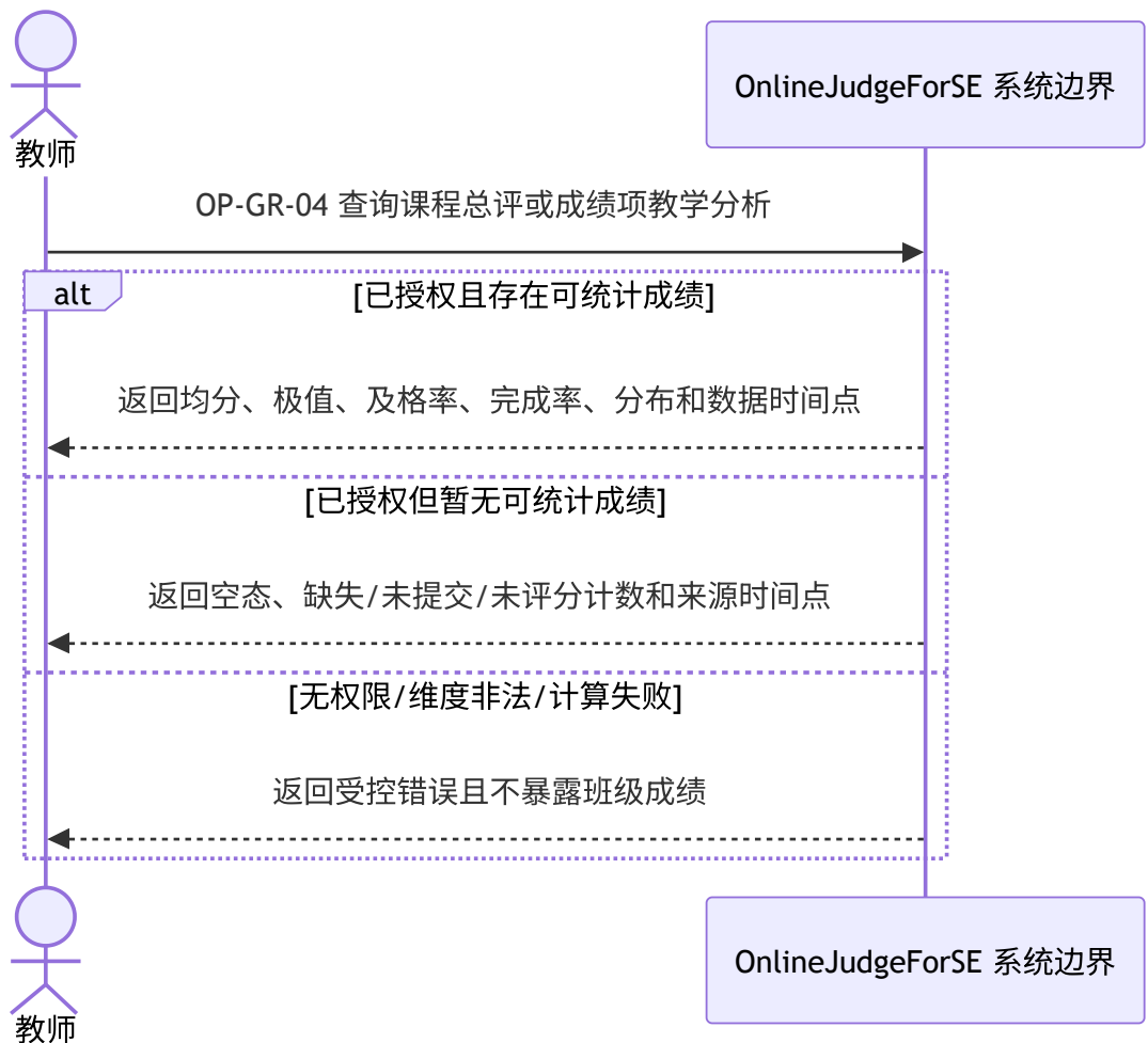
图 4-59 教学分析系统顺序图
