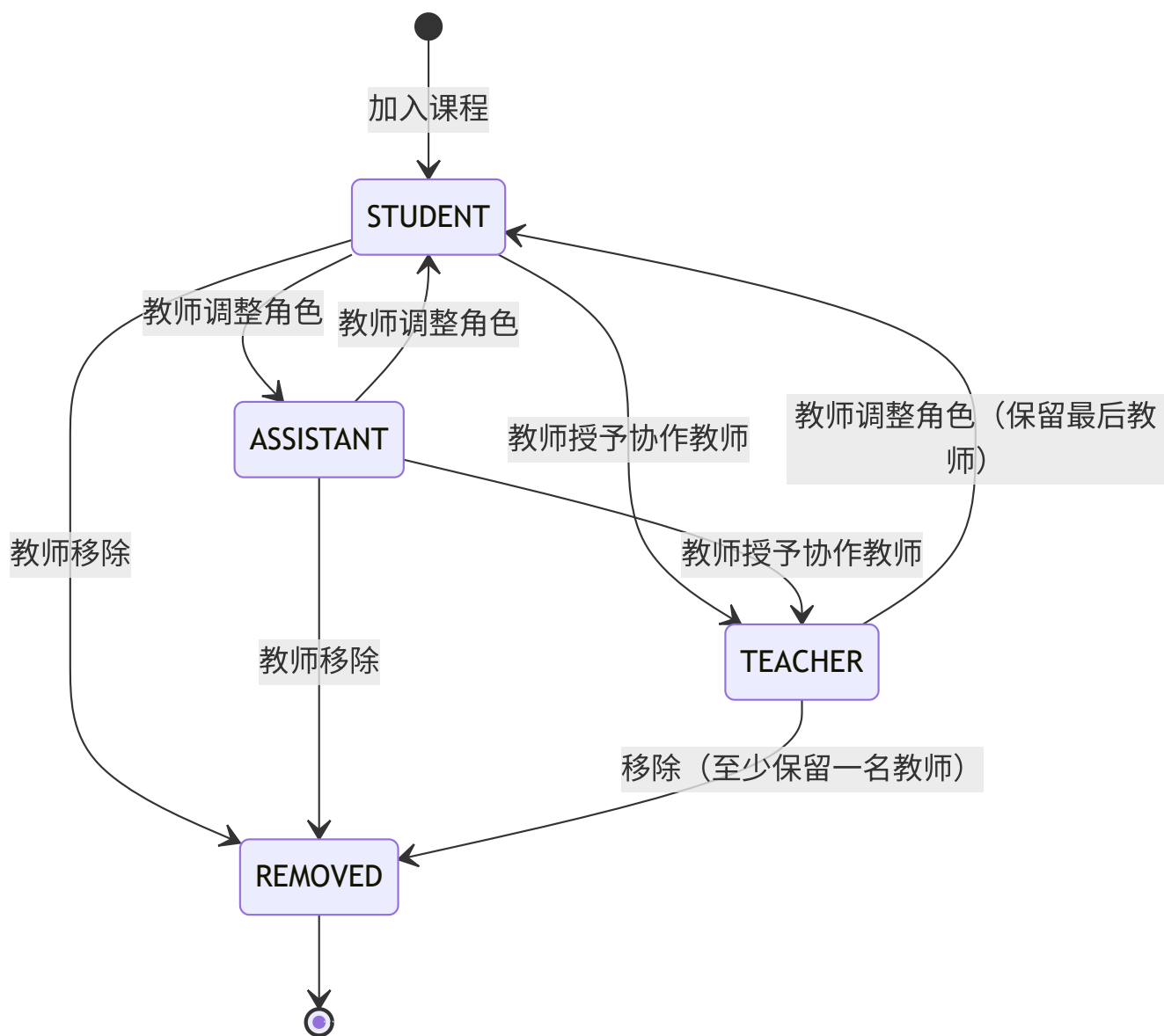
图 4-51 课程成员角色状态图
