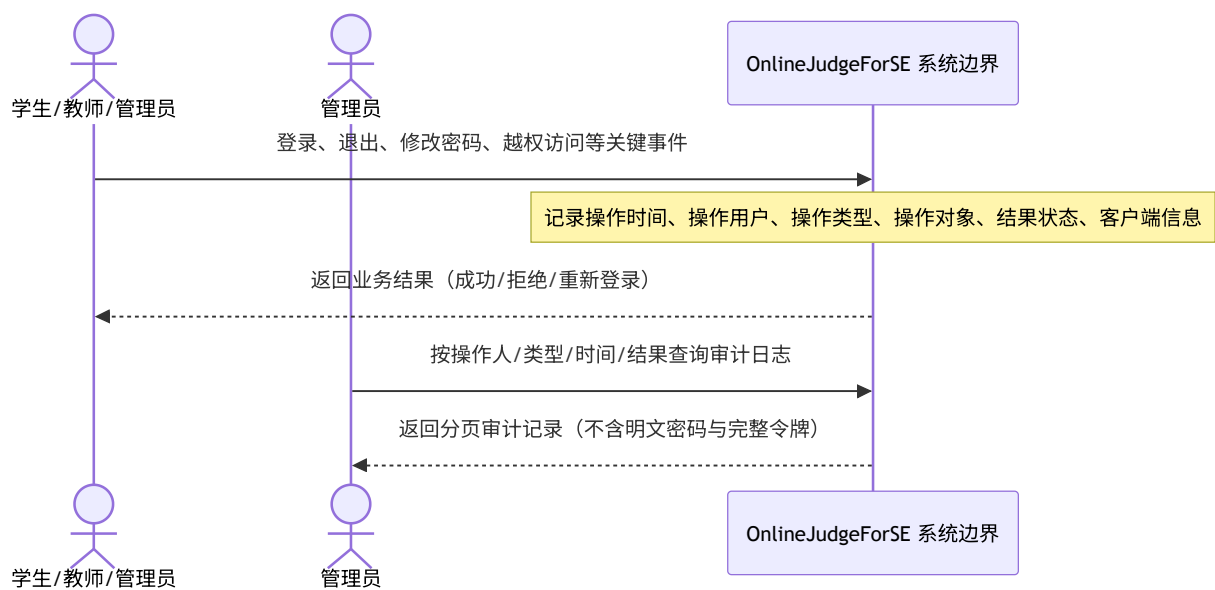
图 4-30 关键操作审计写入与查询系统顺序图
