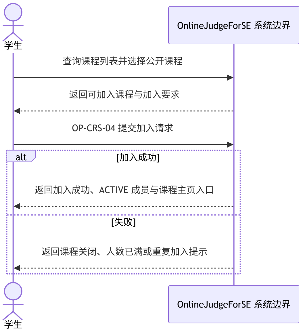
图 4-44 公开加入课程系统顺序图
