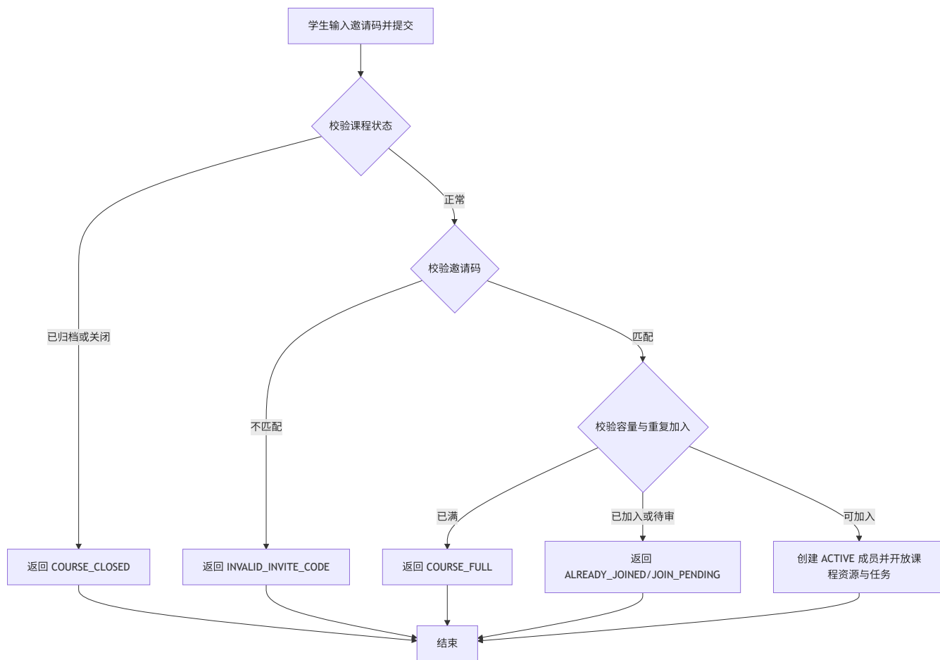
图 4-47 邀请码加入课程活动图
