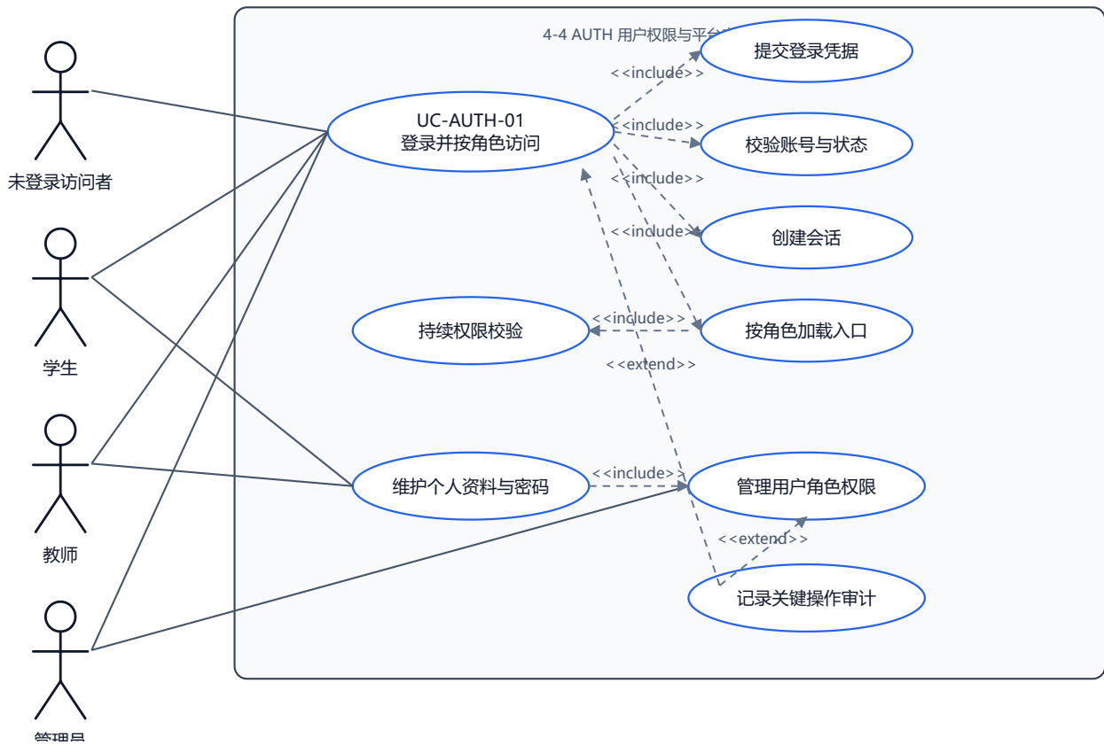
图 4-4 AUTH 用户权限与平台安全用例图
