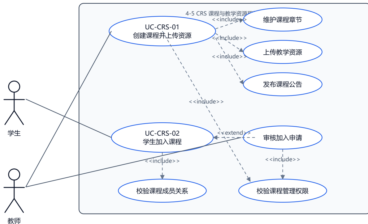
图 4-5 CRS 课程与教学资源用例图
