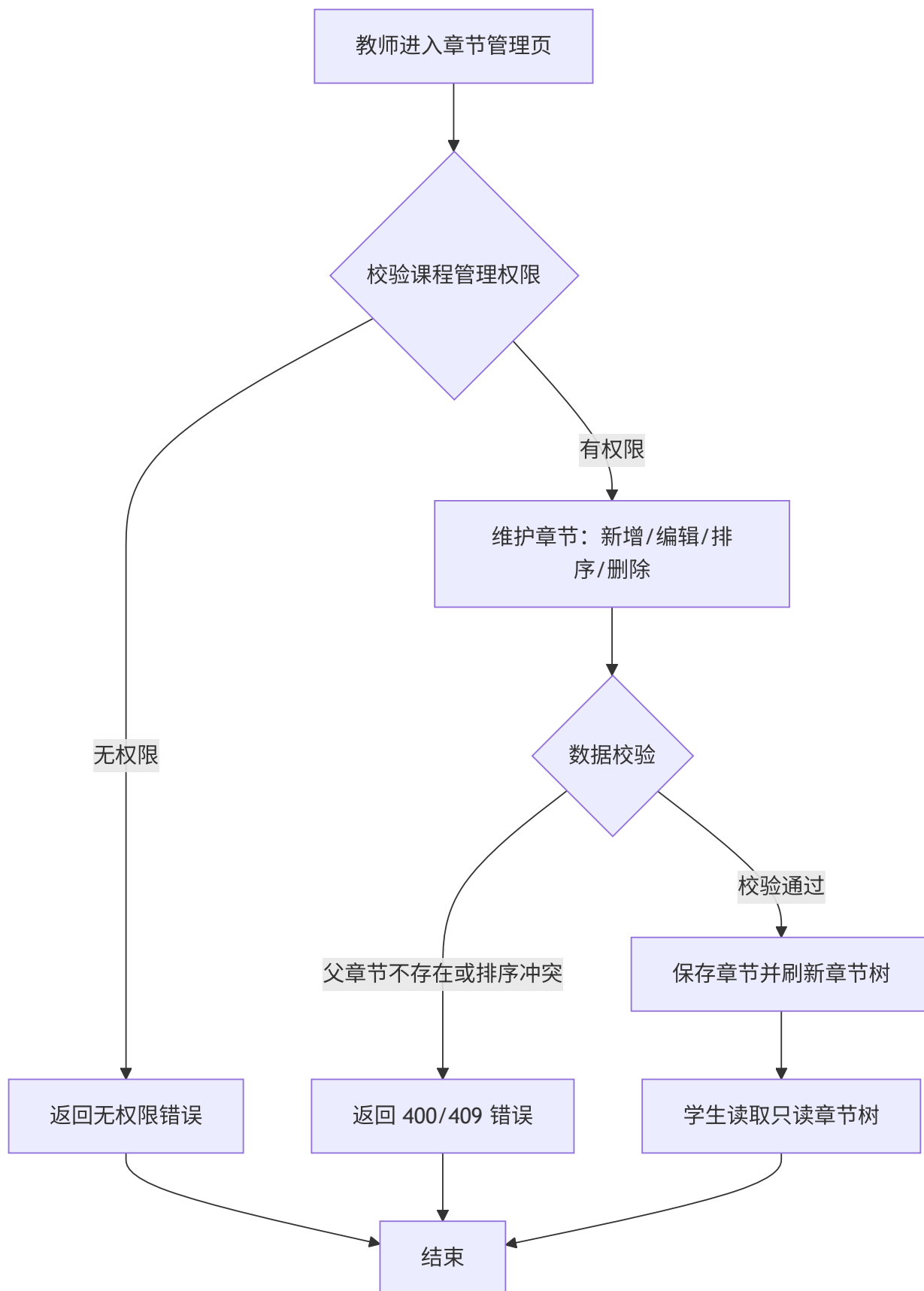
图 4-41 章节目录管理活动图
