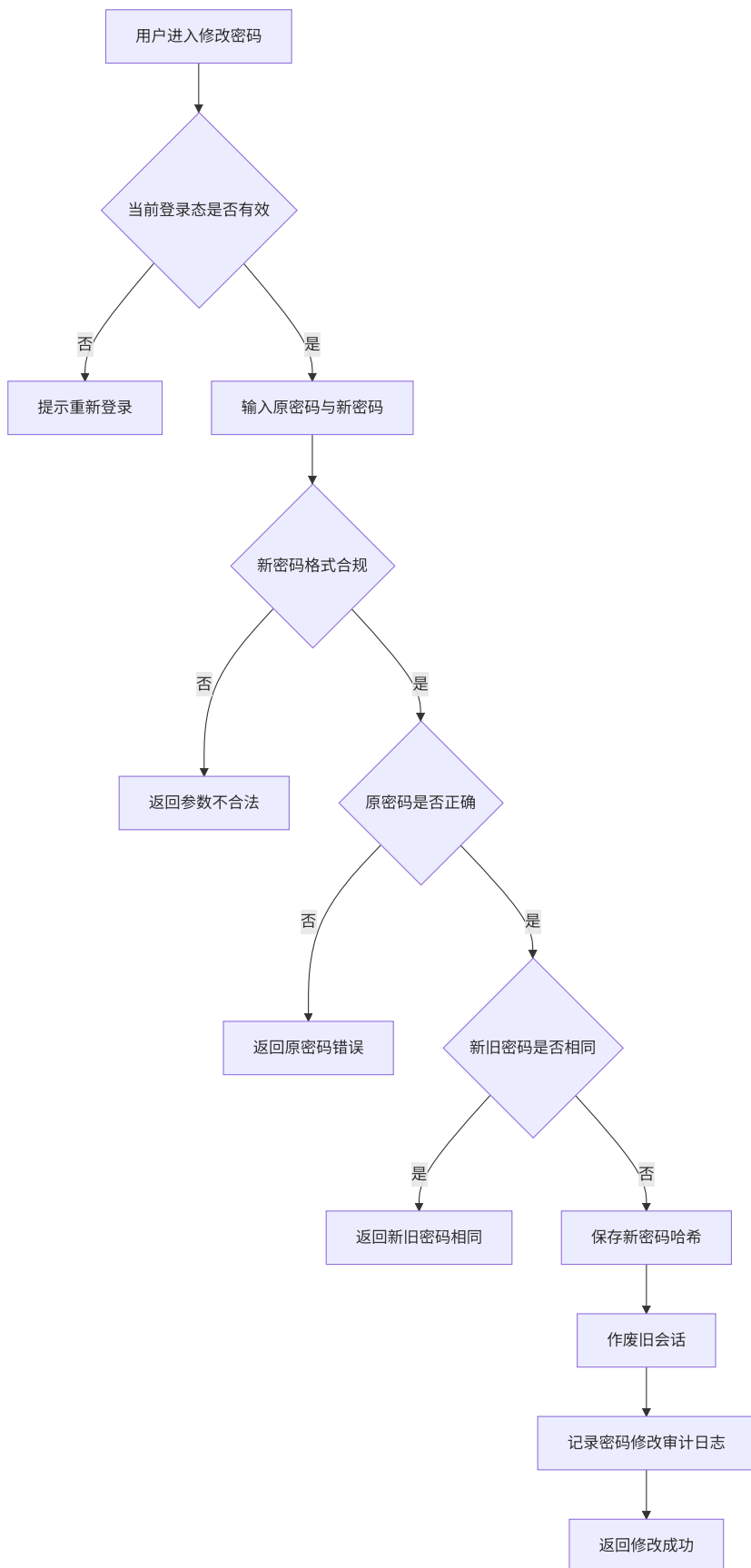
图 4-33 修改密码活动图
