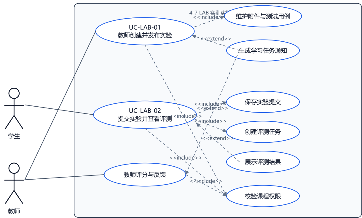
图 4-7 LAB 实训实验用例图
