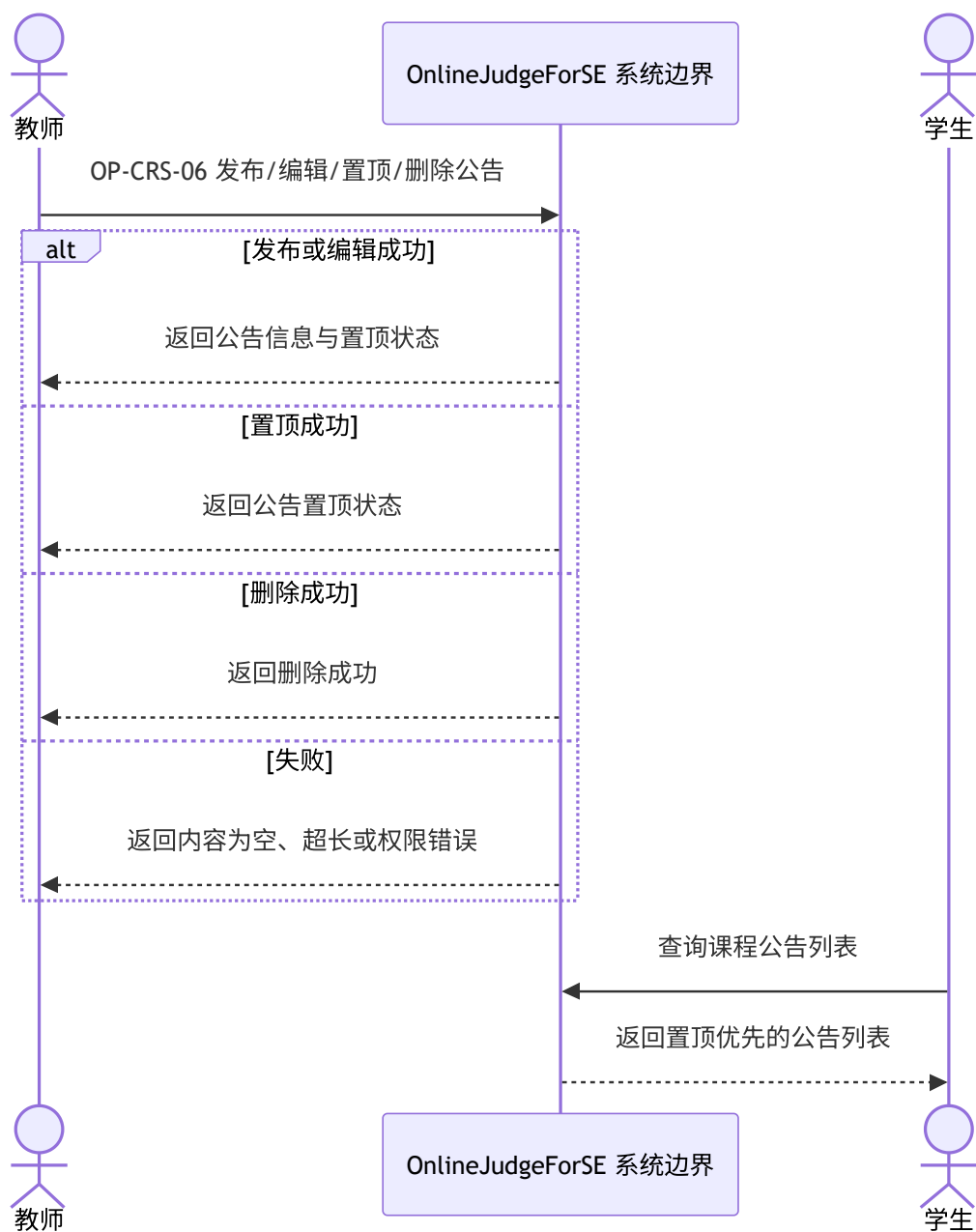
图 4-52 公告发布与置顶系统顺序图
