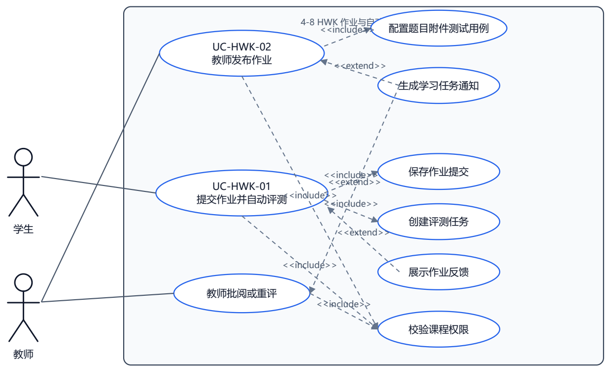
图 4-8 HWK 作业与自动评测用例图
