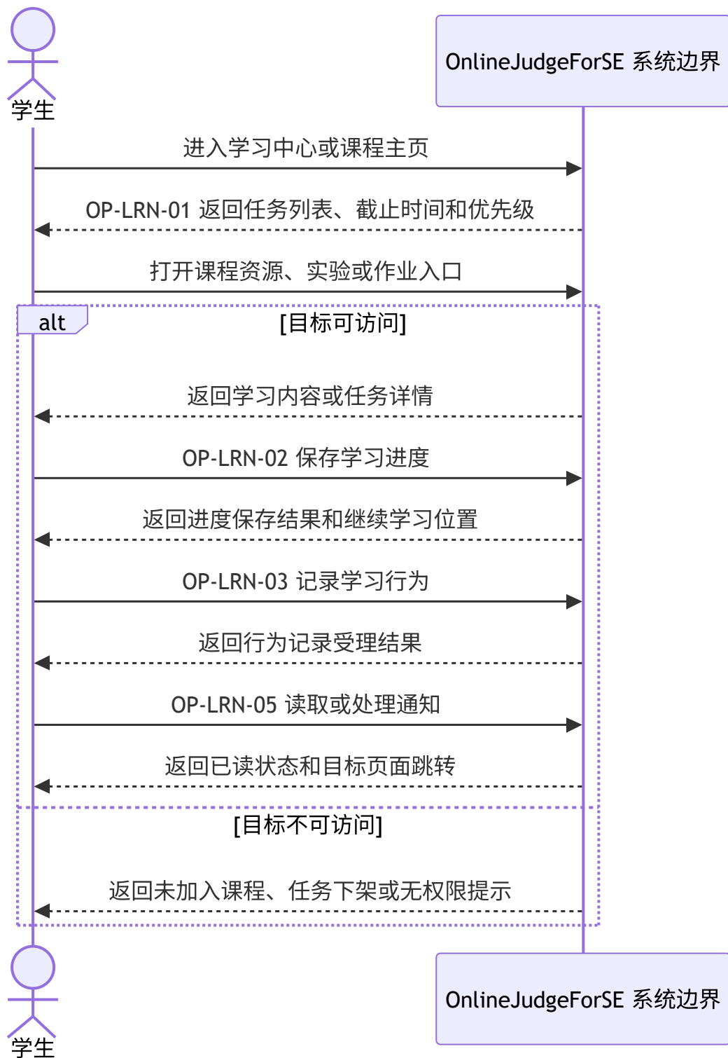
图 4-19 学习任务与进度系统顺序图
