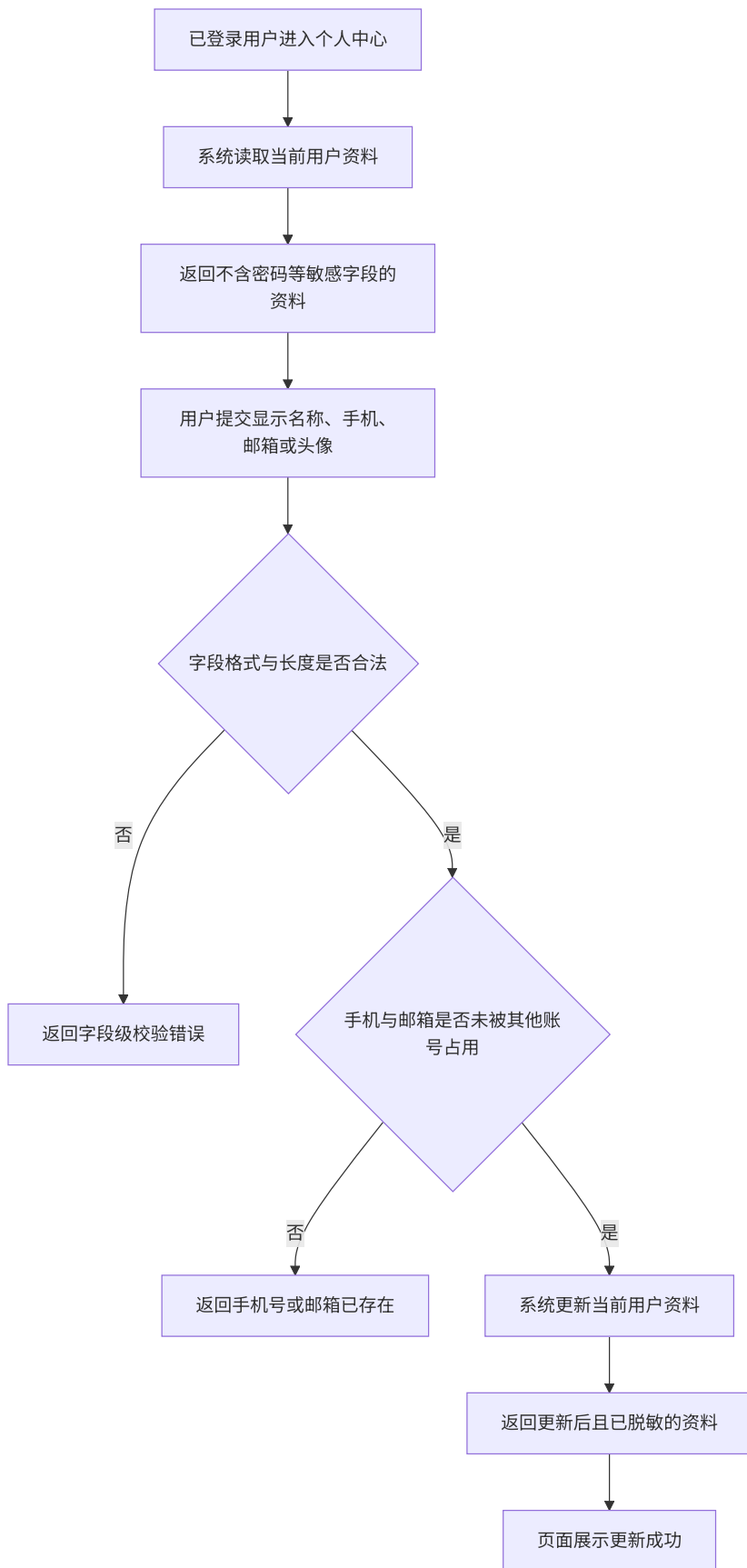
图 4-36 SC-AUTH-05 个人资料查看与修改活动图
