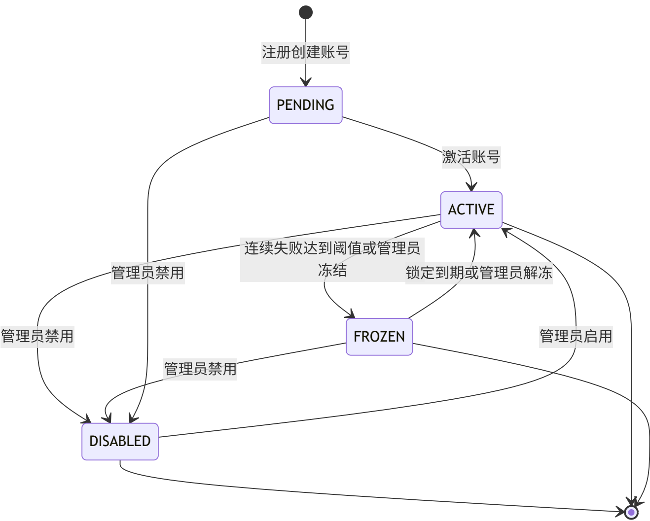
图 4-31 账号状态机
