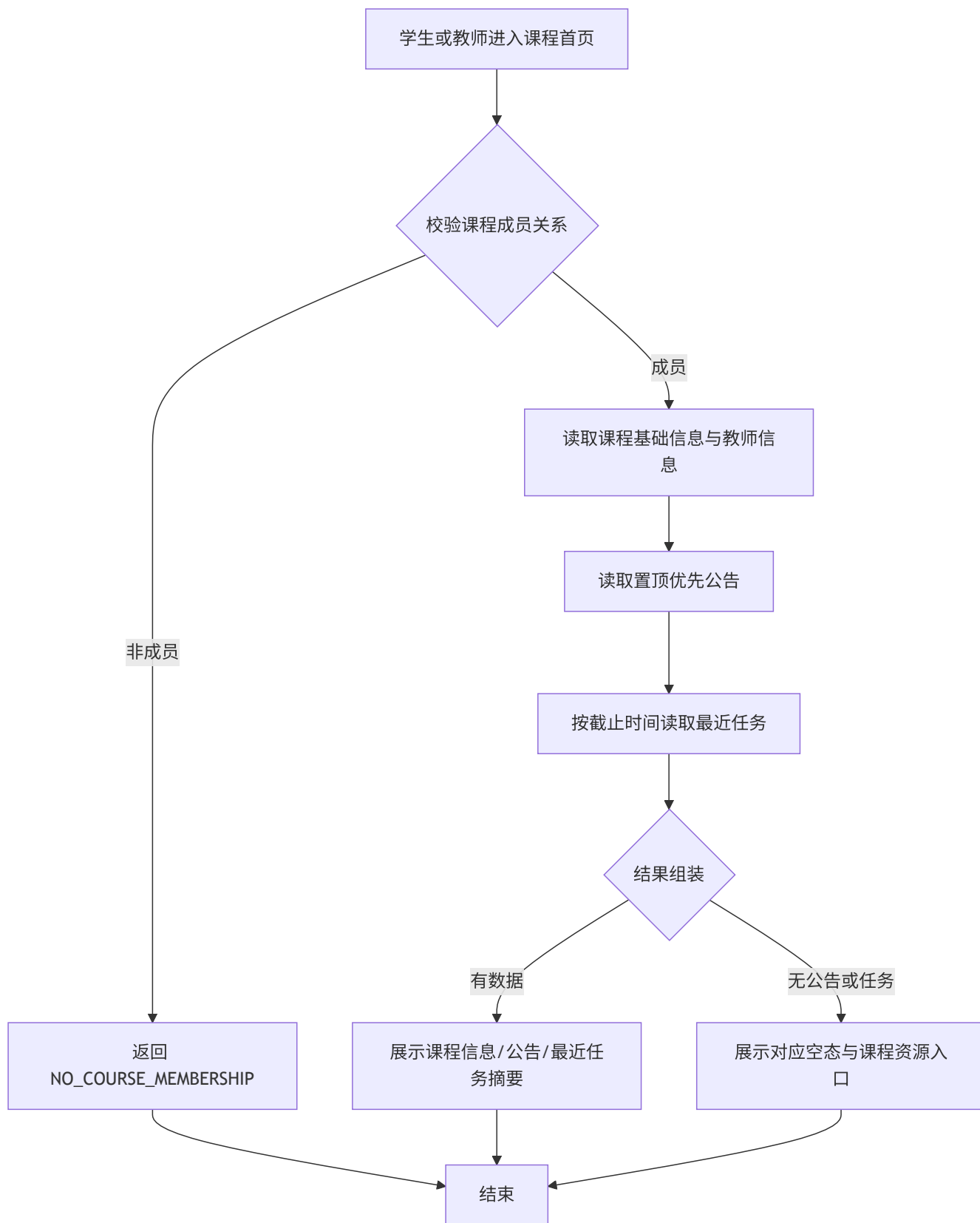
图 4-55 课程首页摘要活动图
