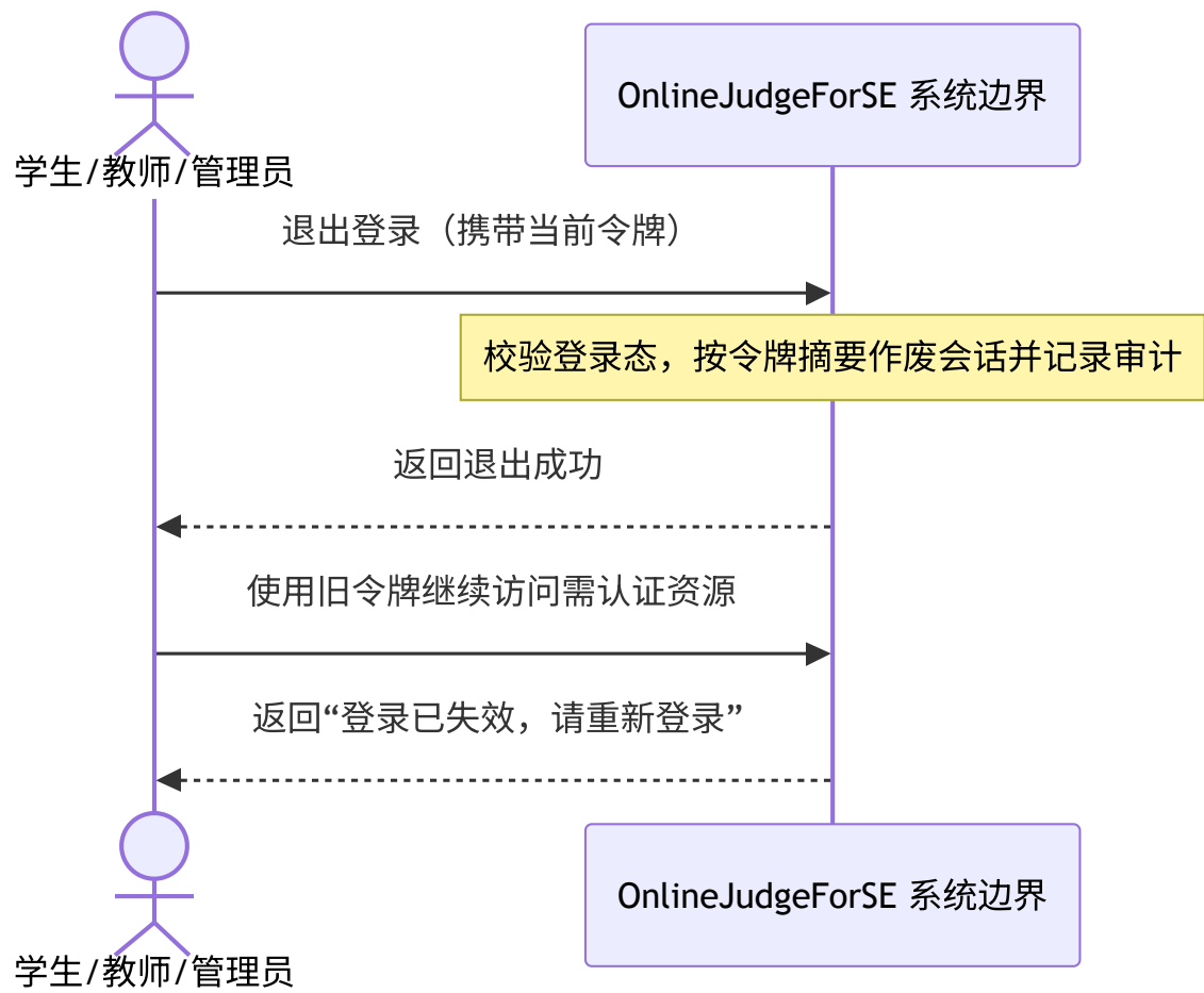
图 4-22 退出登录系统顺序图
