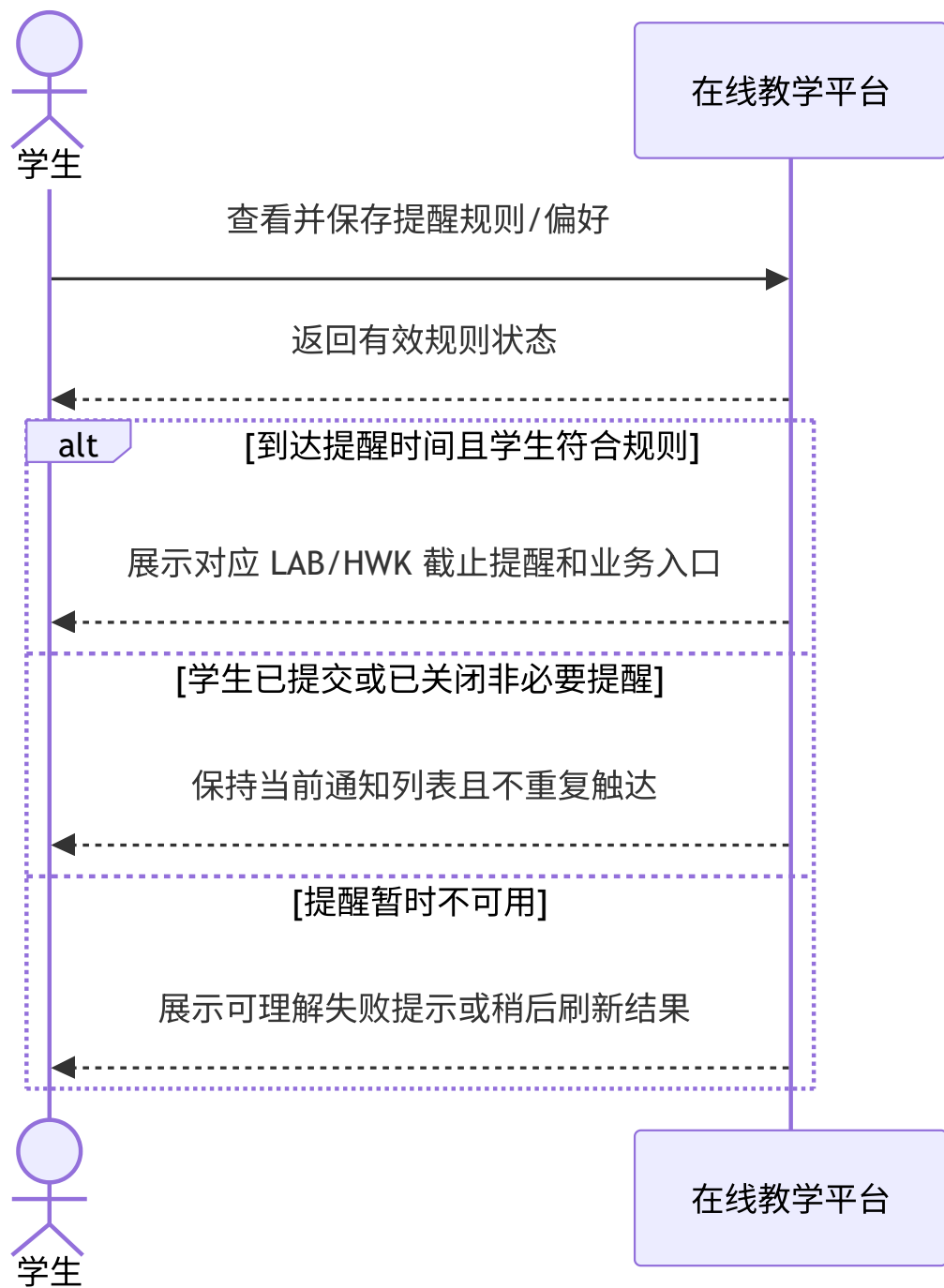
3.3.4.2 学习任务与进度系统顺序图
