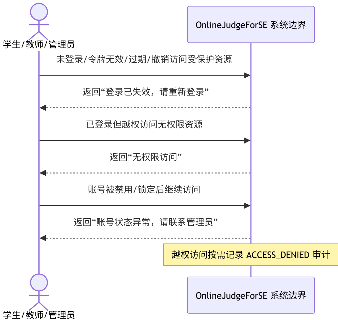
图 4-29 安全异常拦截系统顺序图
