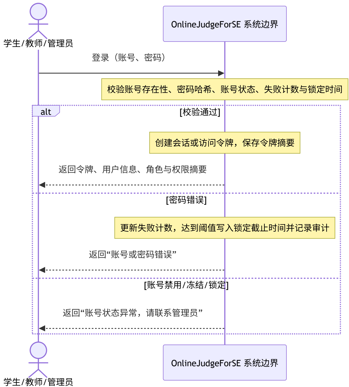
图 4-21 账号密码登录系统顺序图
