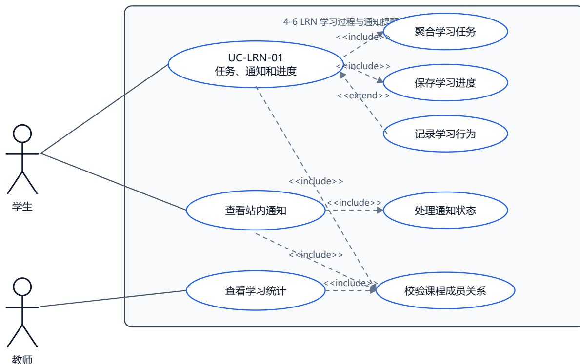
图 4-6 LRN 学习过程与通知提醒用例图
