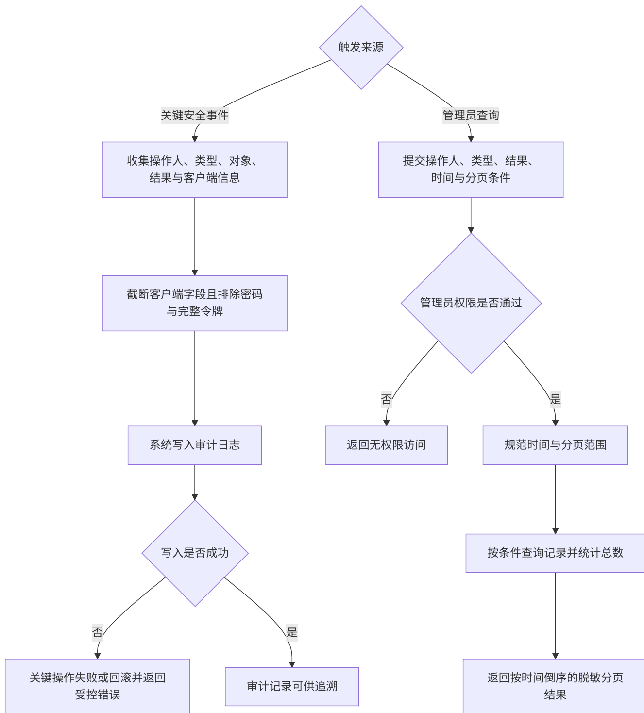
图 4-37 SC-AUTH-11 审计写入与查询活动图
