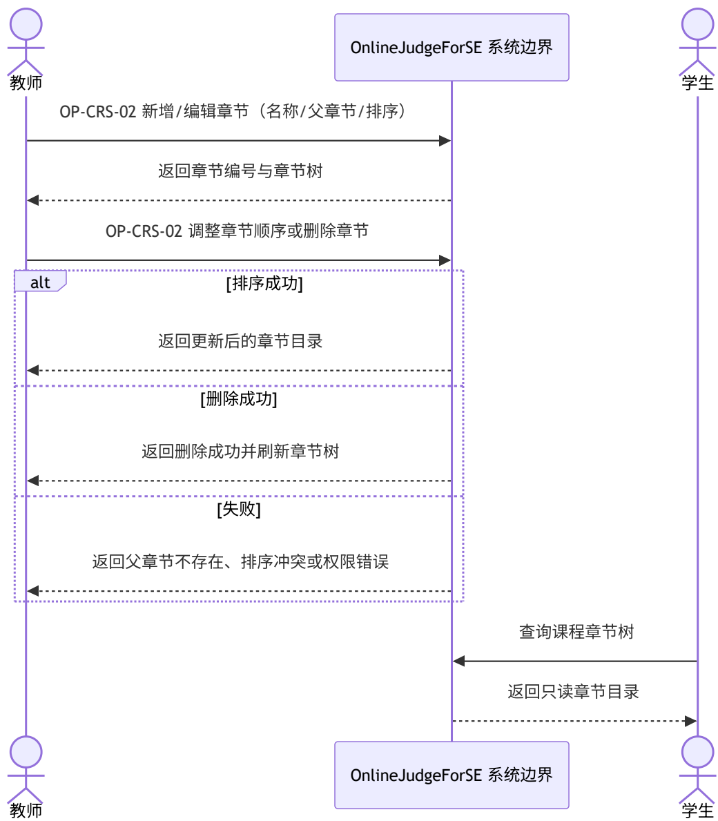
图 4-40 章节目录管理系统顺序图
