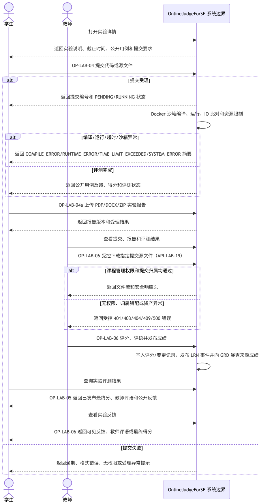
图 4-13 实验提交评测系统顺序图
