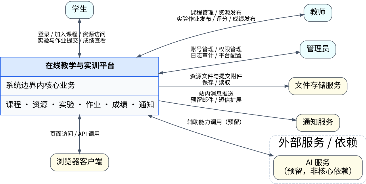
图 2-1 系统上下文图
