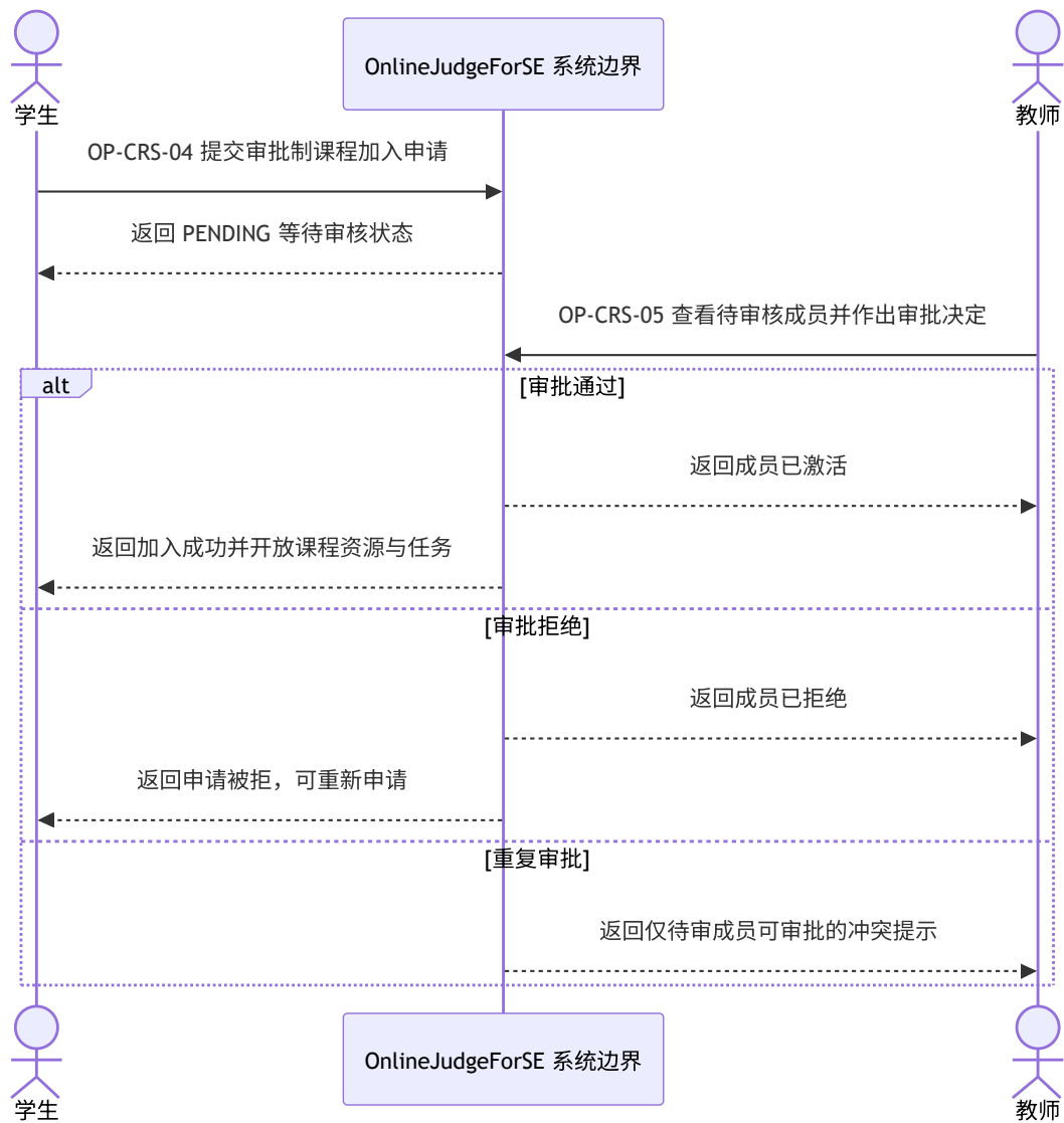
图 4-48 审批加入课程系统顺序图
