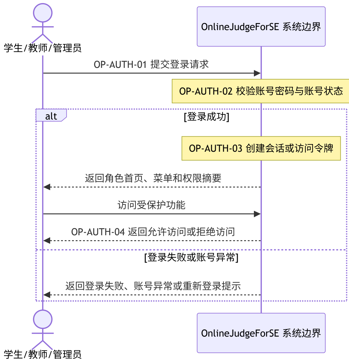
图 4-11 登录系统顺序图
