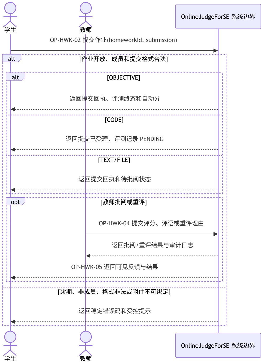
图 4-14A 学生提交作业并触发自动评测系统顺序图
