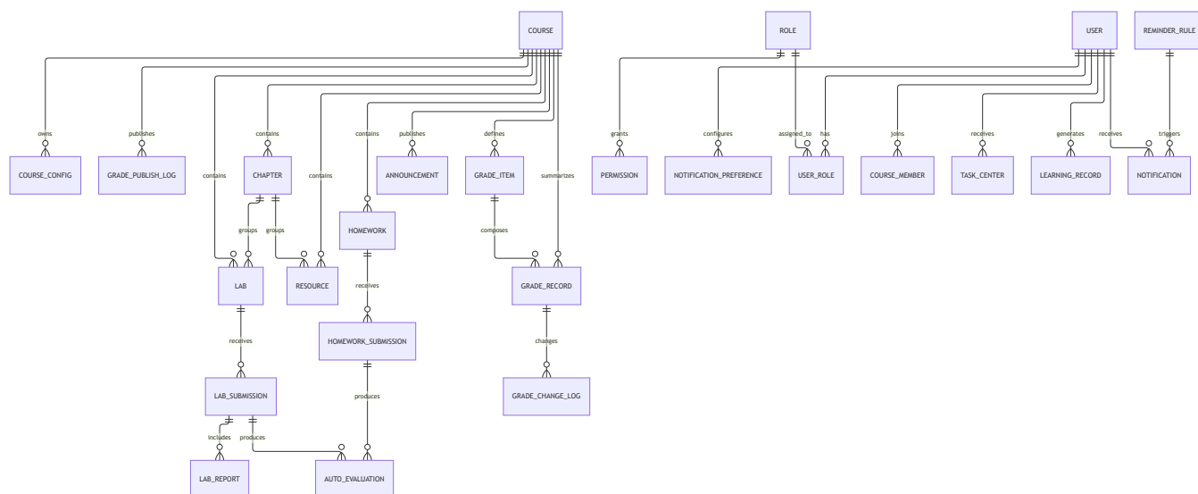
图 7-1 核心数据 ER 图（逻辑实体层）
