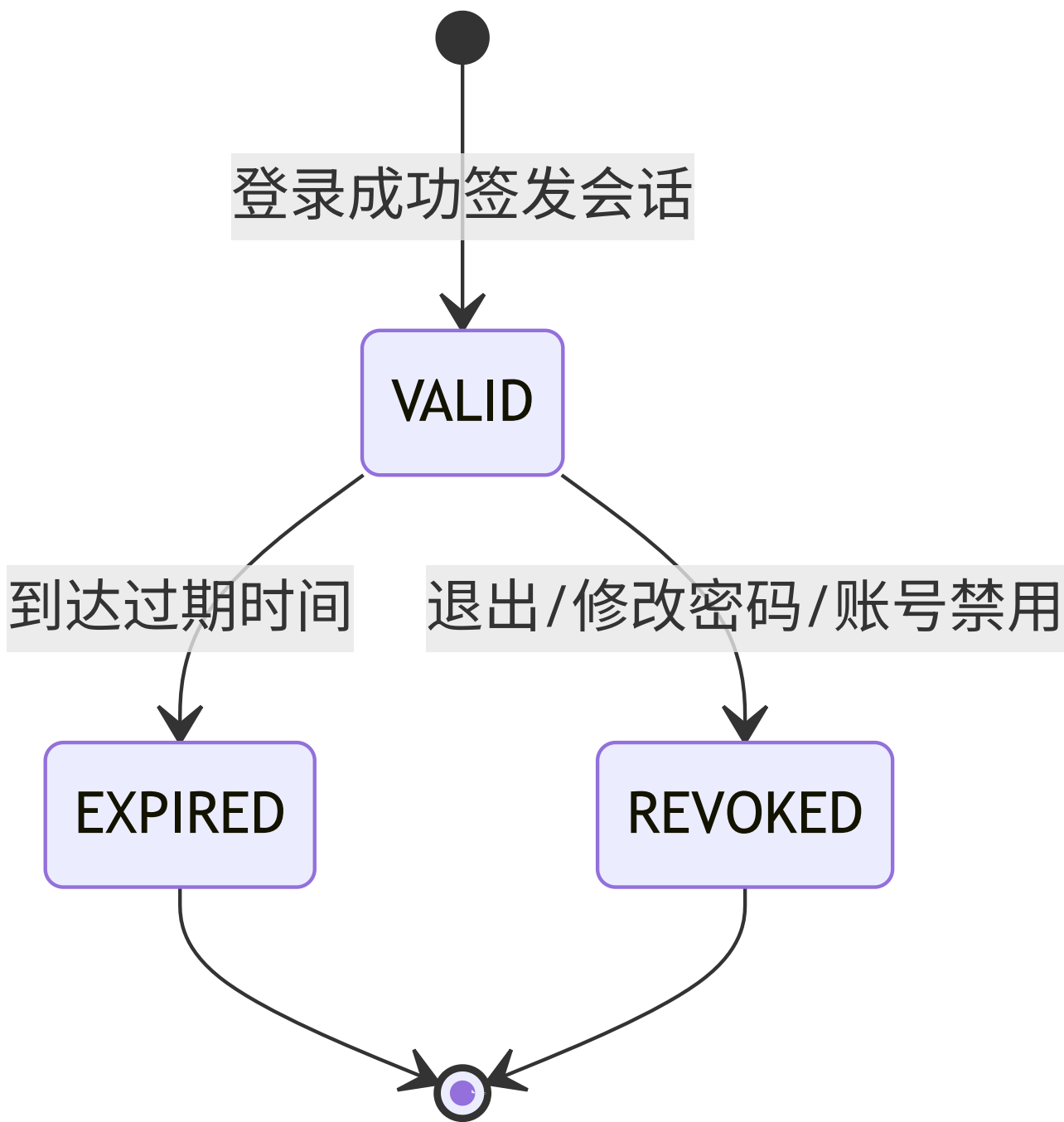
图 4-32 会话状态机
