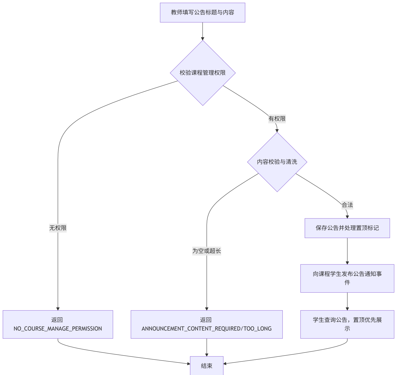
图 4-53 公告发布与置顶活动图
