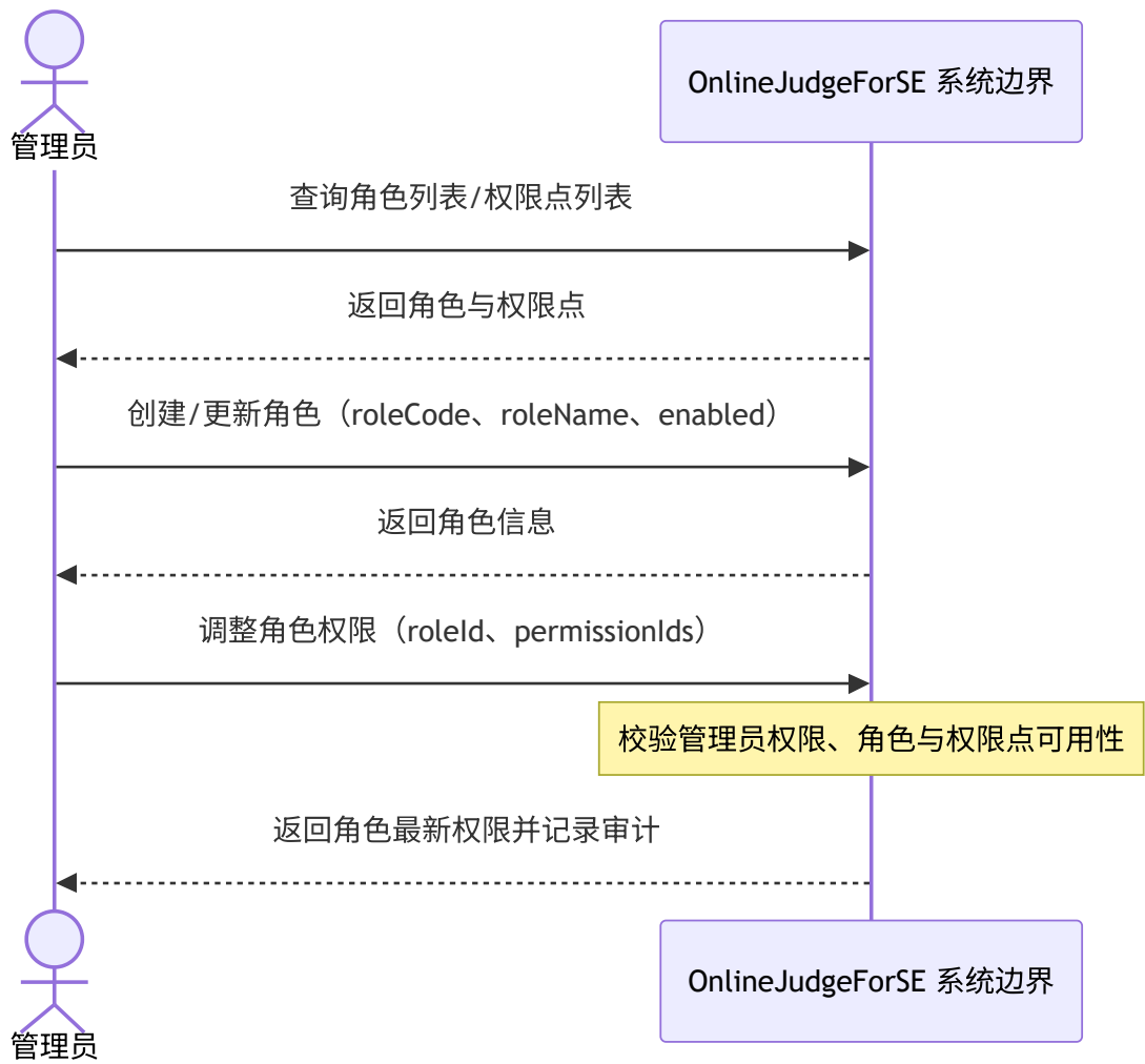
图 4-28 角色与角色权限维护系统顺序图
