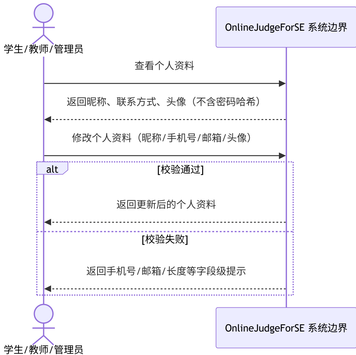
图 4-24 个人资料查看与修改系统顺序图
