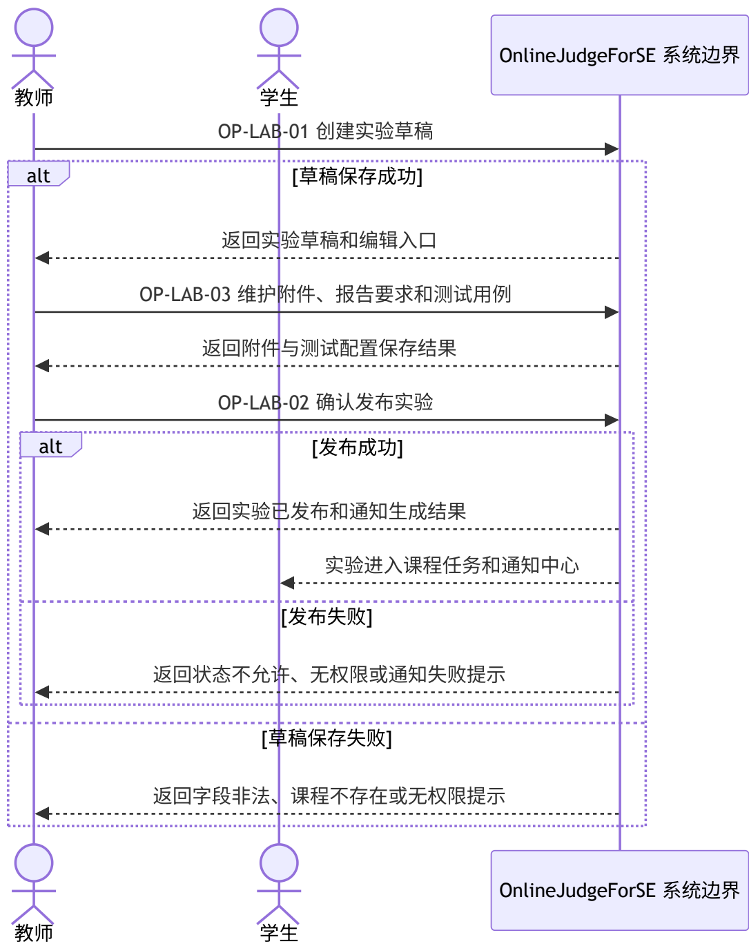
图 4-18 实验创建与发布系统顺序图
