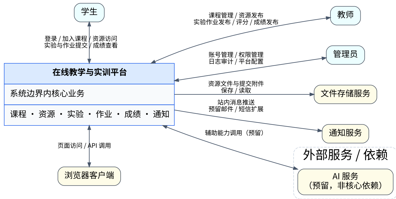
图 2-1 系统上下文图
