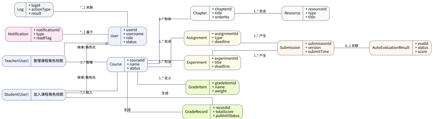
图 5-2 核心对象结构图
