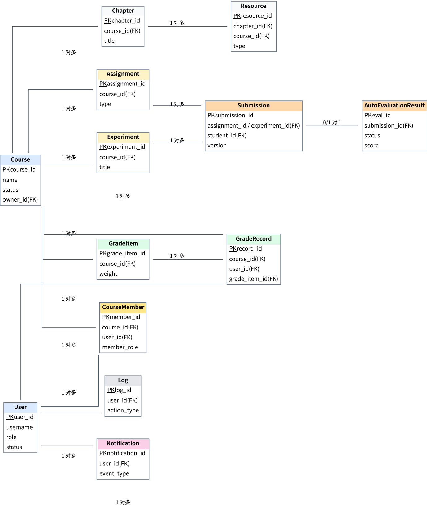
图 7-1 核心数据 ER 图
