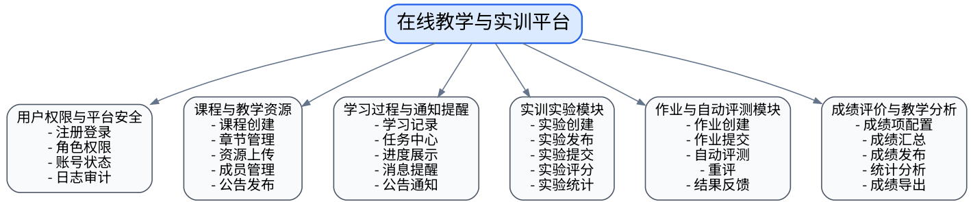
图 5-1 系统总体功能结构图
