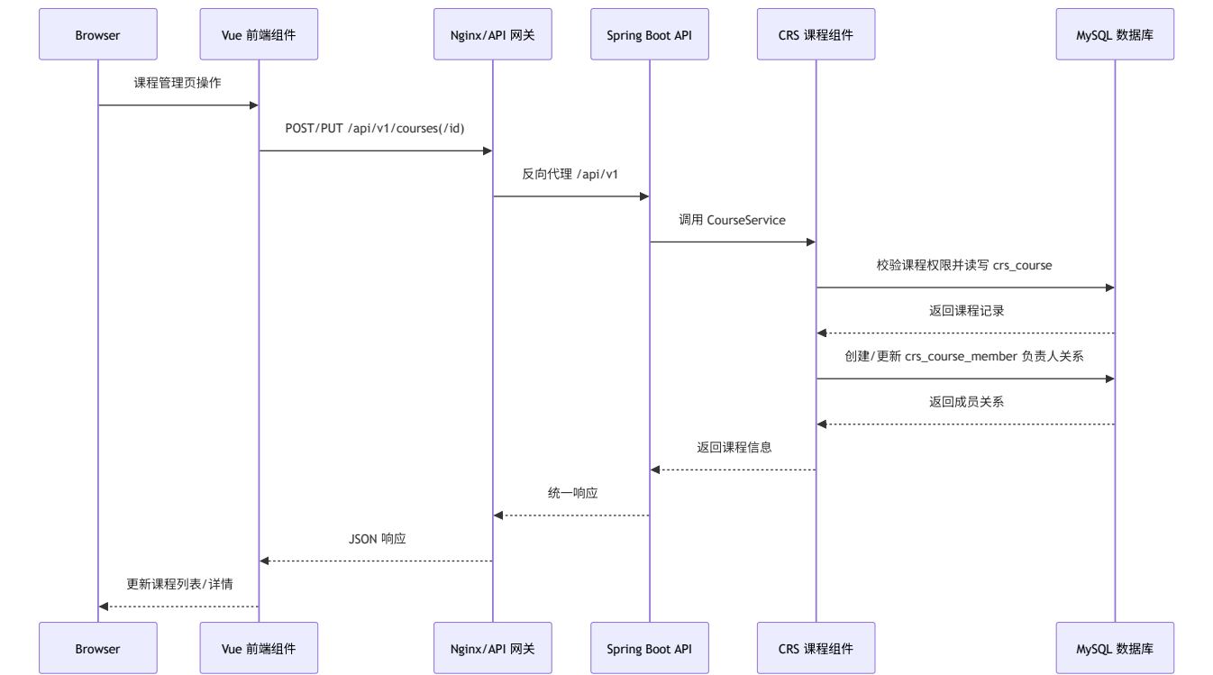
图 2-6 课程创建与维护组件顺序图
