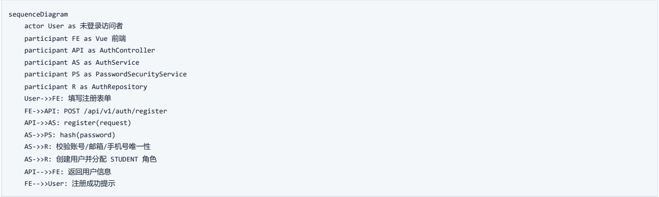
图 5-2 SC-AUTH-01 学生自助注册组件级顺序图
