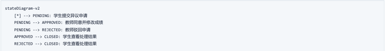
图 3-9 成绩异议申请状态机
