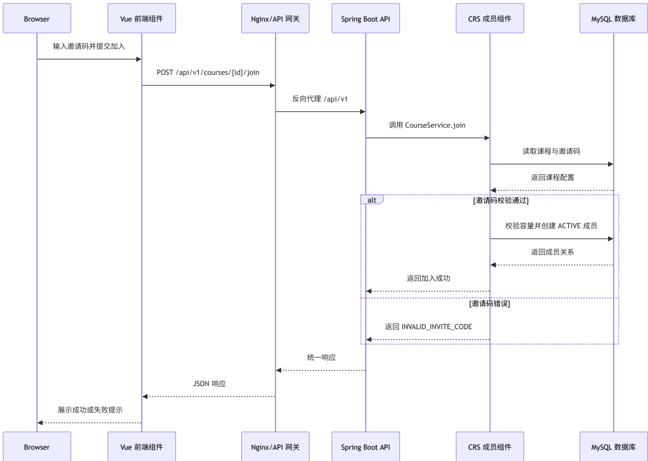
图 2-10 邀请码加入课程组件顺序图
