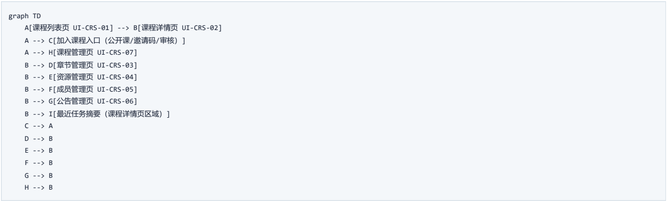
图 3-2 CRS 页面流转图
