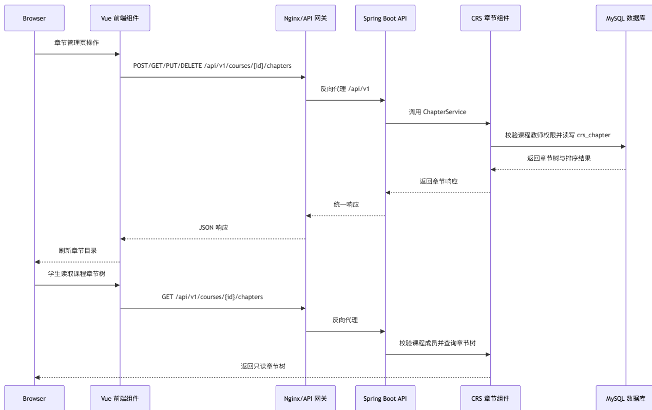
图 2-7 章节目录管理组件顺序图
