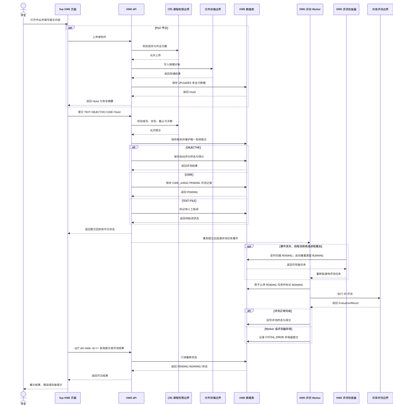
图 5-2-HWK-01 学生提交作业并触发自动评测组件顺序图。Mermaid 图源：docs/diagrams/arch/fig_5_2_hwk_01_submission_component.mmd。
