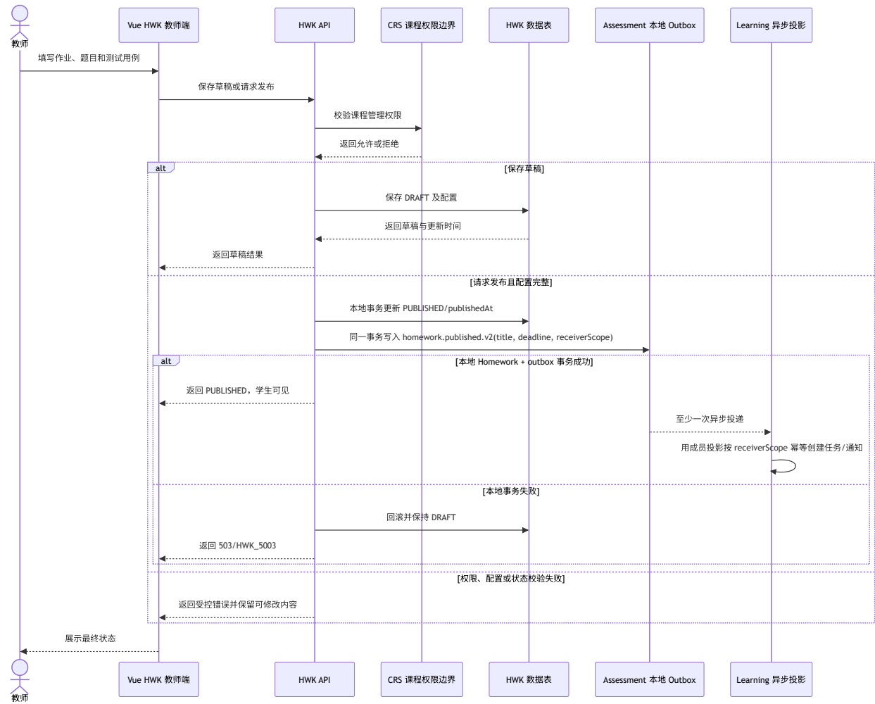
图 5-2-HWK-02 教师创建并发布作业组件顺序图。Mermaid 图源：docs/diagrams/arch/fig_5_2_hwk_02_publish_component.mmd。
