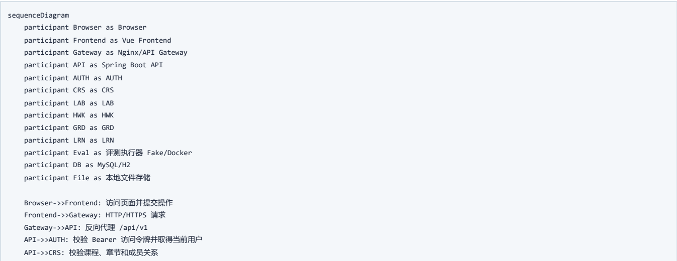
图 2-3 组件交互顺序图
