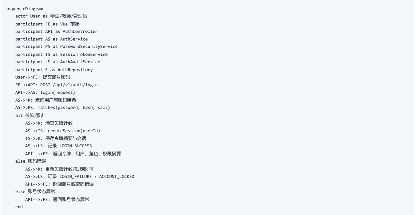
图 5-3 SC-AUTH-02 账号密码登录组件级顺序图
