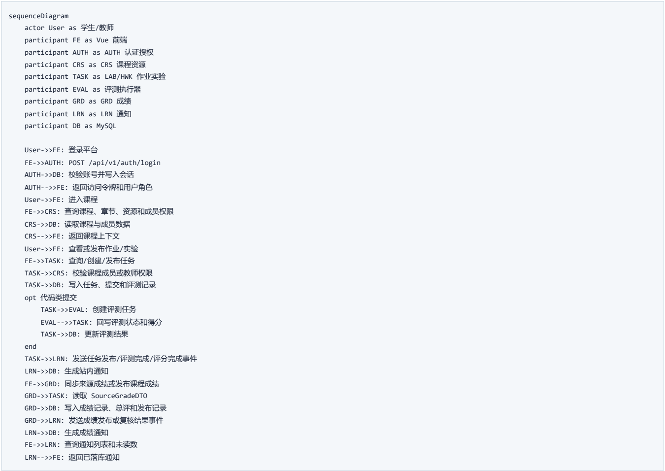
图 5-1 端到端主流程运行顺序图
