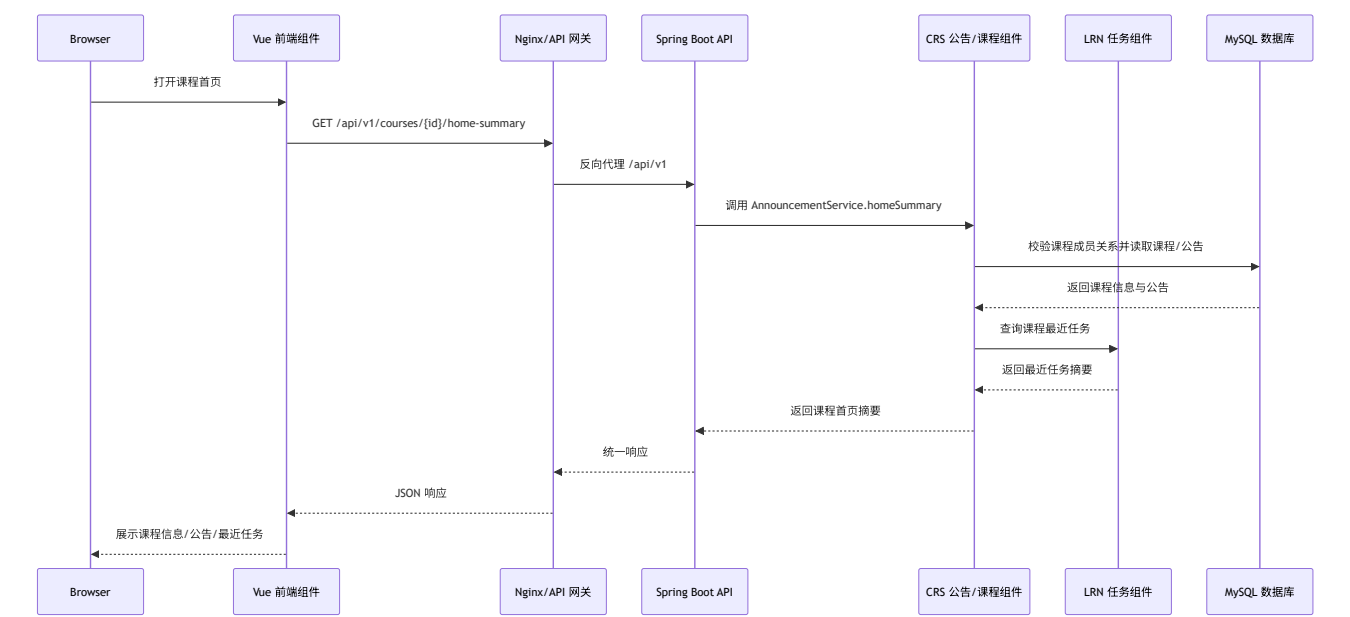
图 2-14 课程首页摘要组件顺序图
