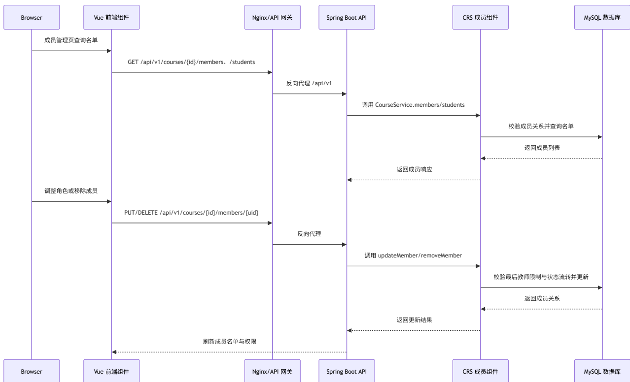
图 2-12 成员管理组件顺序图
