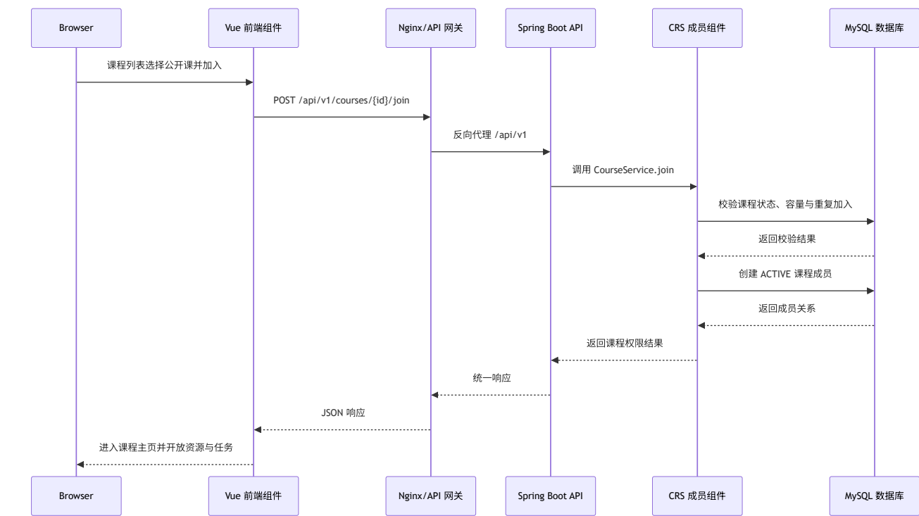
图 2-9 公开加入课程组件顺序图
