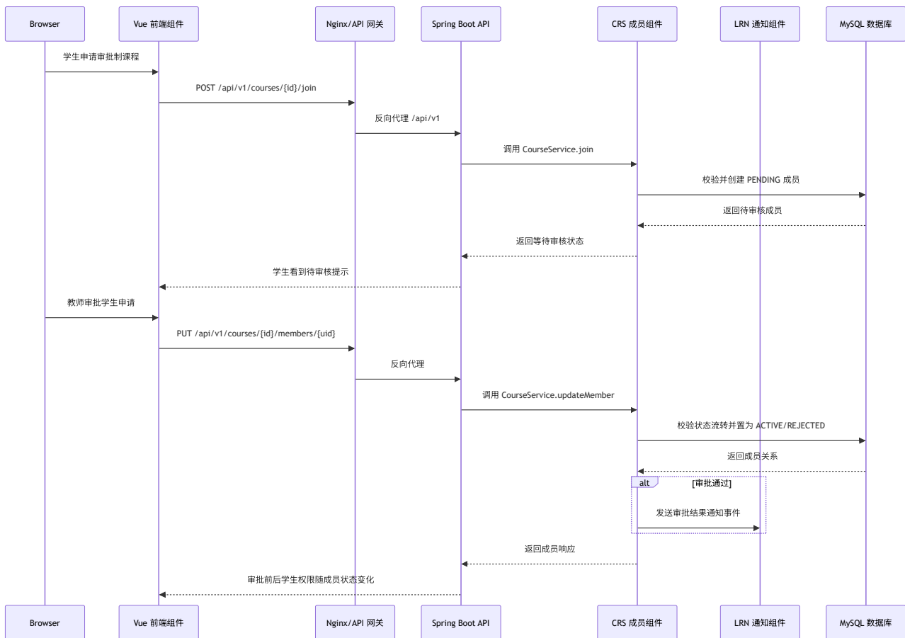
图 2-11 审批加入课程组件顺序图
