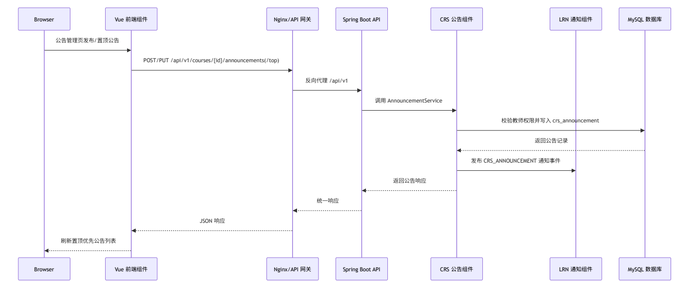
图 2-13 公告发布与置顶组件顺序图
