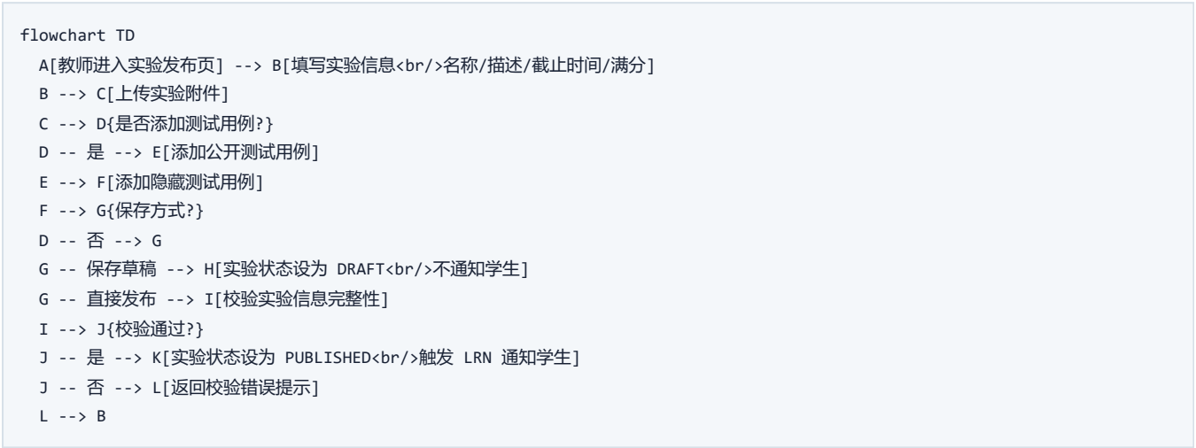
图 3-4-2 教师发布实验流程图
