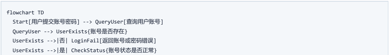
图 3-3 AUTH 用户登录流程图
