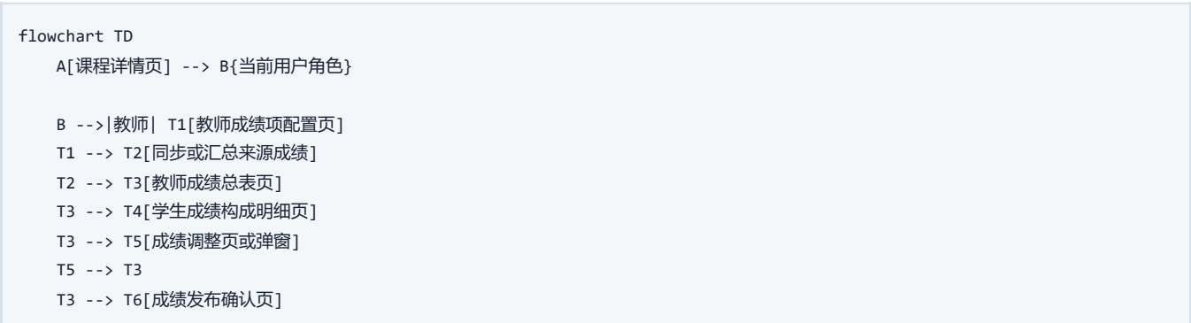
图 3-6-1 GRD 页面流转图
