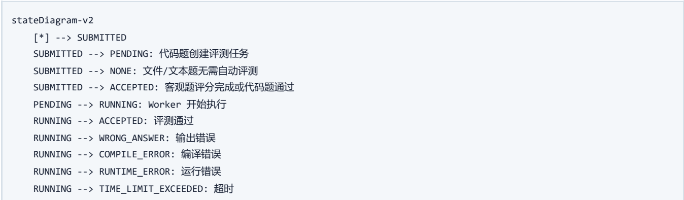
图 3-5-8 HWK 提交与评测状态机
