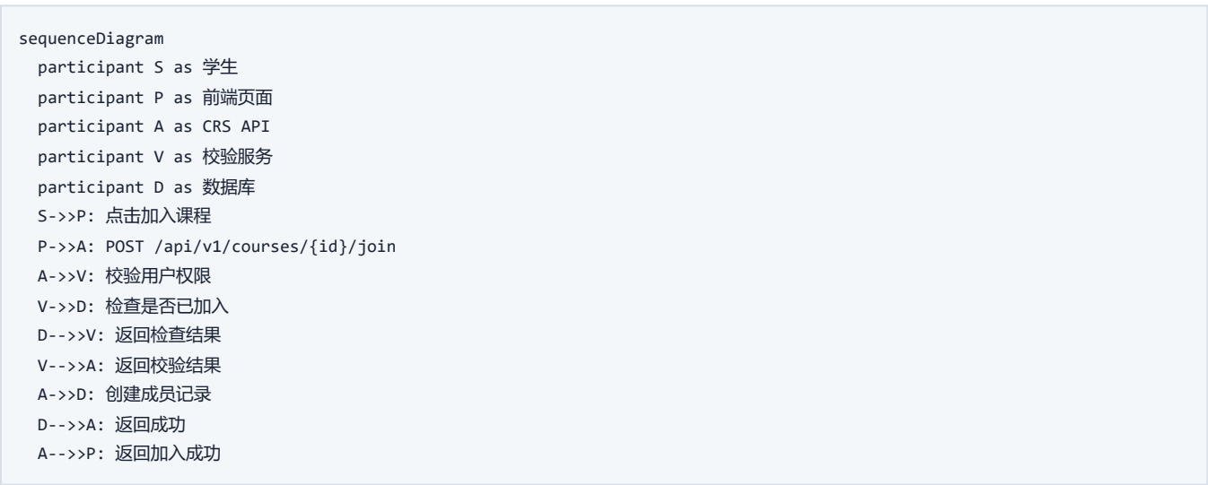
图 3-2-8 加入课程流程图
