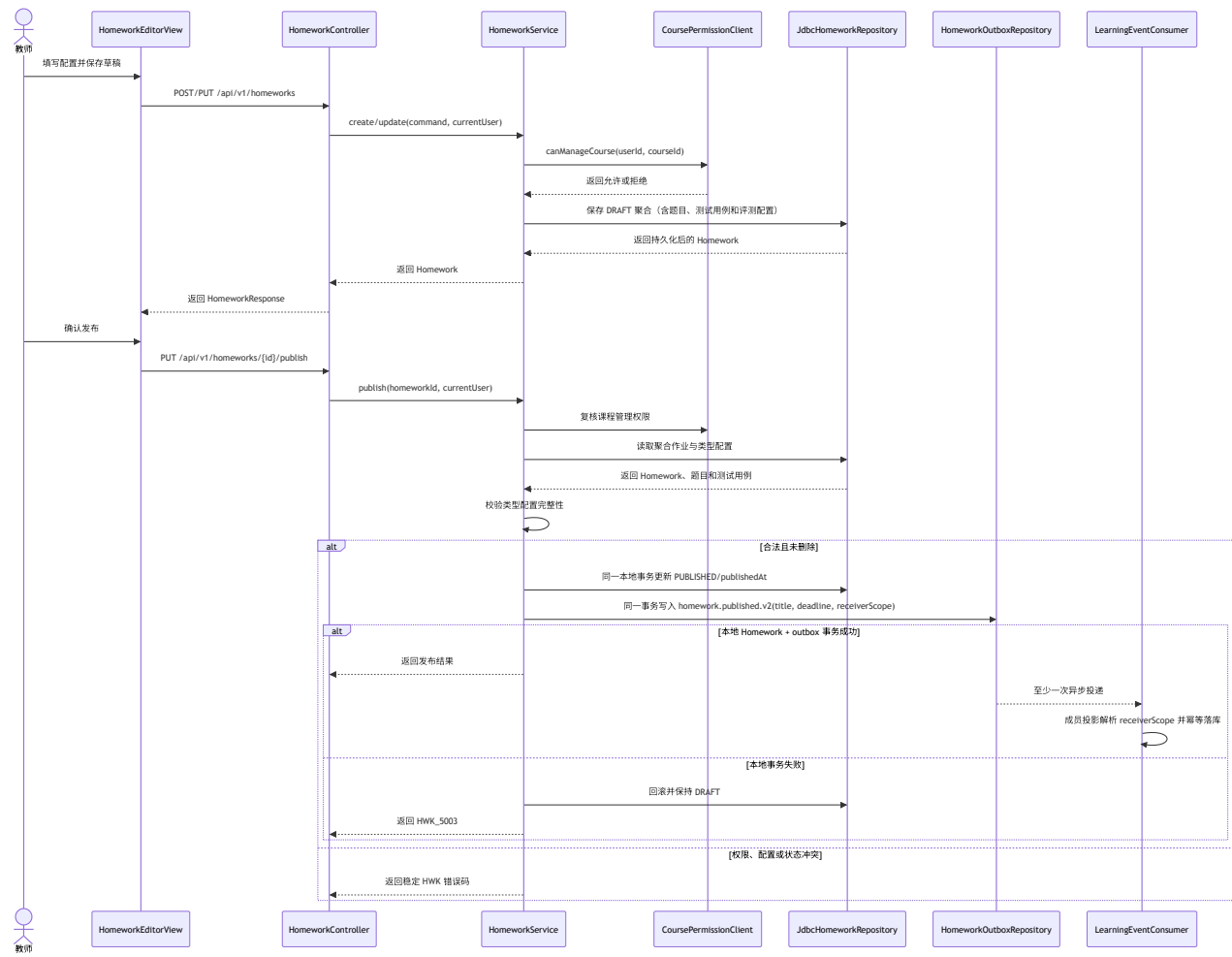
图 3-5-3A UC-HWK-02 教师创建并发布作业对象顺序图
