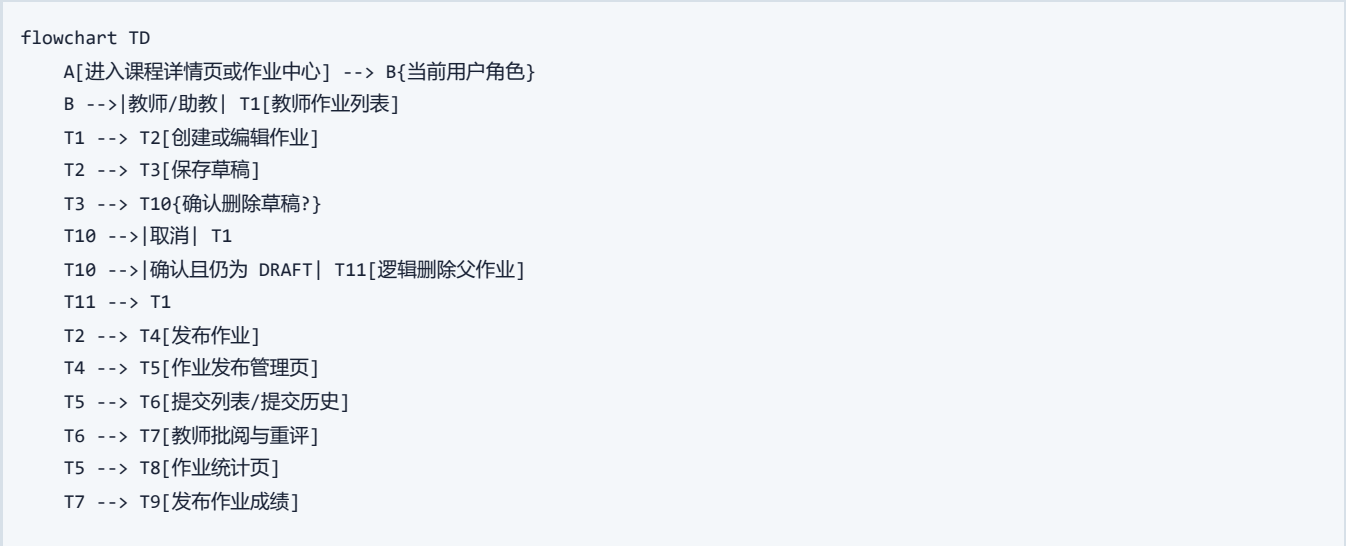
图 3-5-1 HWK 页面流转图
