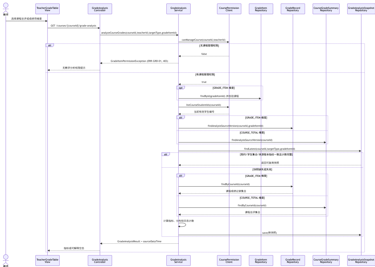
图 3-6-13 GRD 教学分析对象级顺序图
