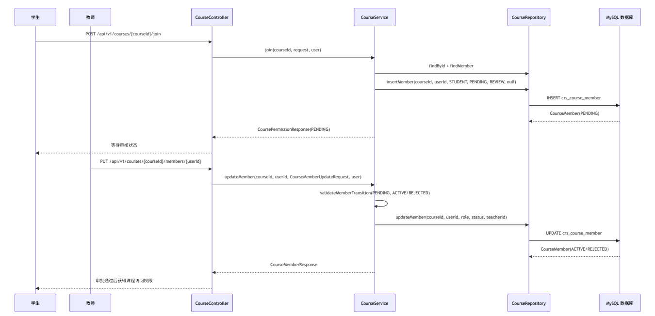
图 3-2-16 CRS-SC-07 成员管理对象顺序图
