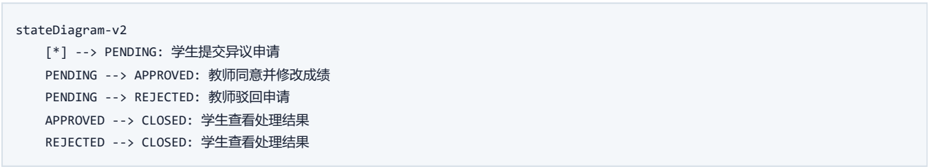
图 3-6-10 GRD 成绩异议申请状态机
