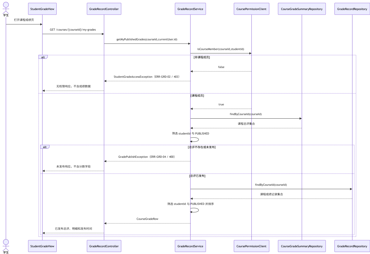
图 3-6-11 GRD 学生成绩查询对象级顺序图
