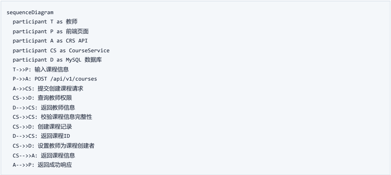
图 3-2-2 CRS 创建课程顺序图
