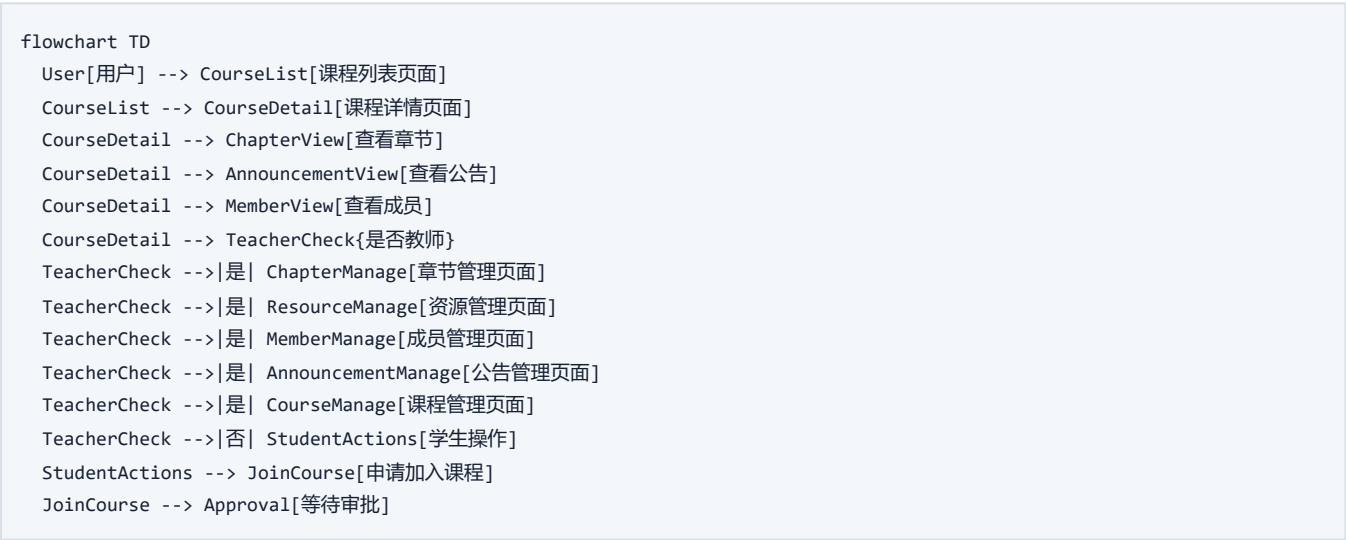
图 3-2-1 CRS 页面流转图
