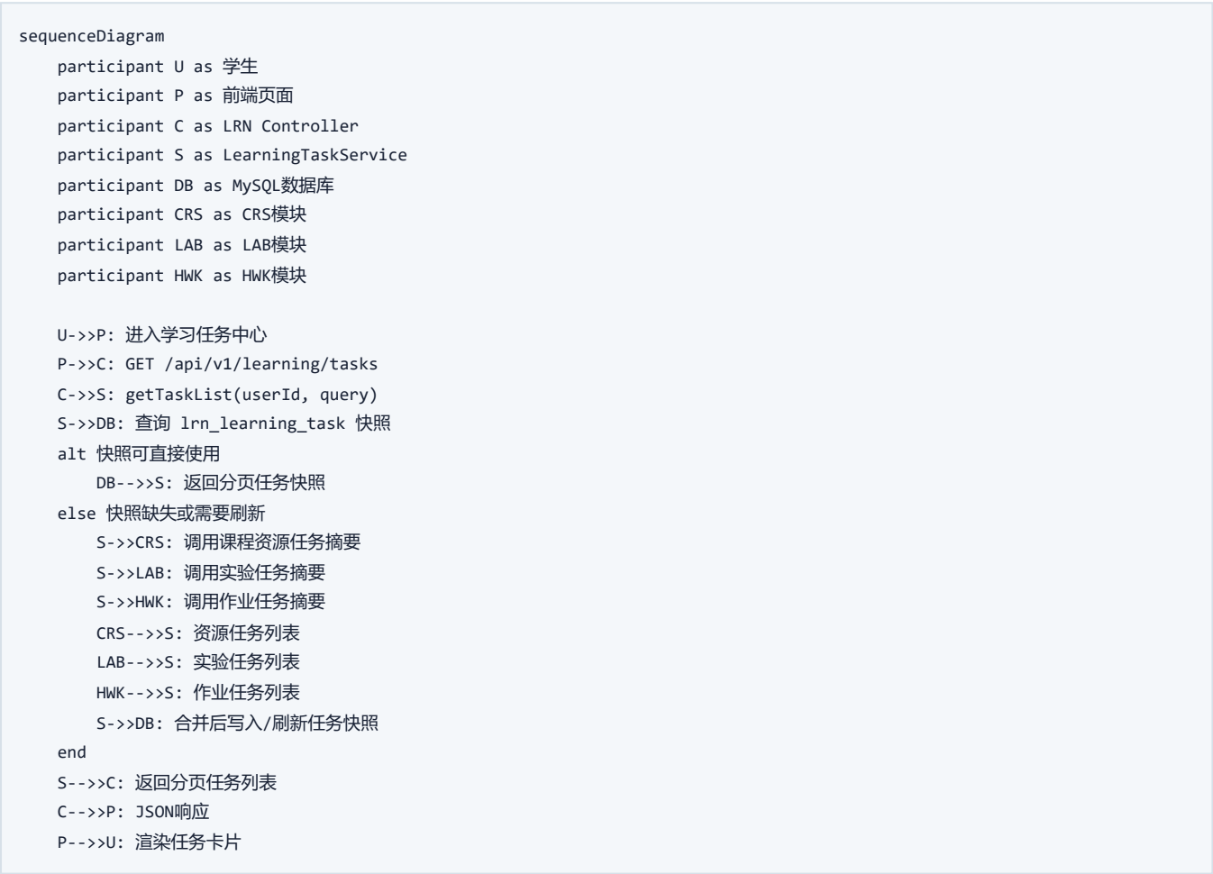
图 3-3-2 LRN 学习任务加载顺序图
