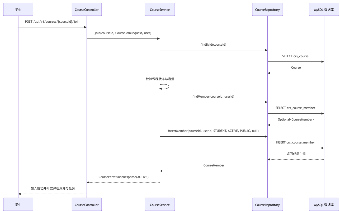
图 3-2-14 CRS-SC-05 邀请码加入课程对象顺序图
