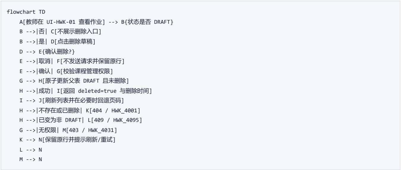
图 3-5-3A HWK 教师删除草稿流程图
