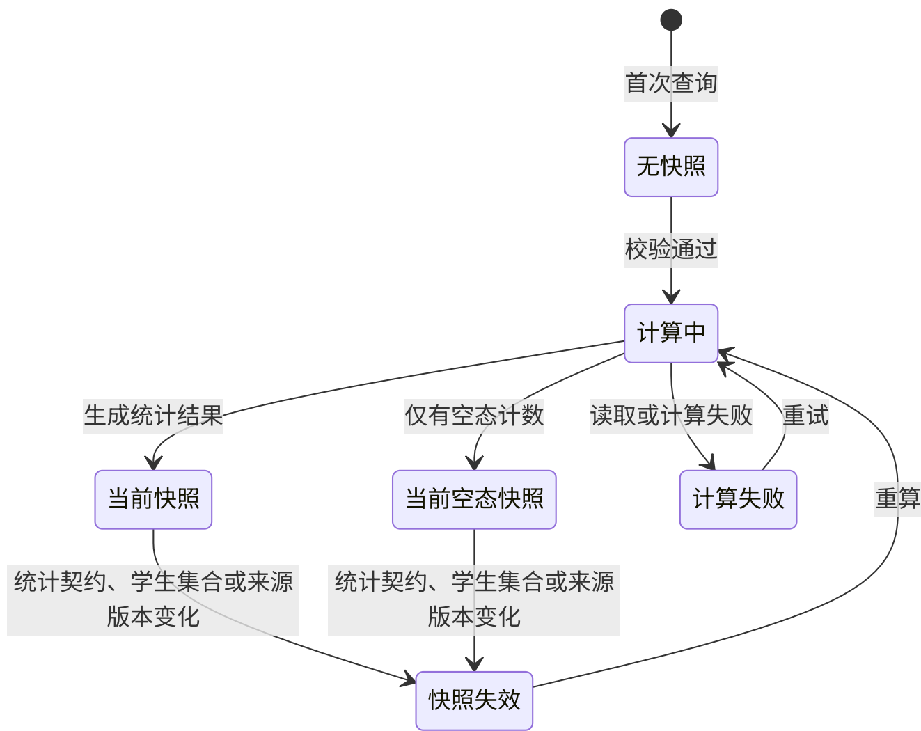
图 3-6-15 GRD 教学分析派生状态图
