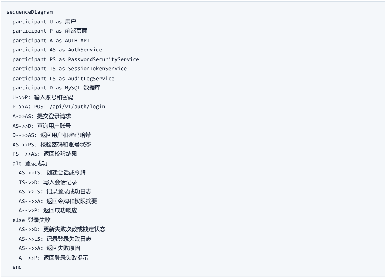
图 3-2 AUTH 登录顺序图
