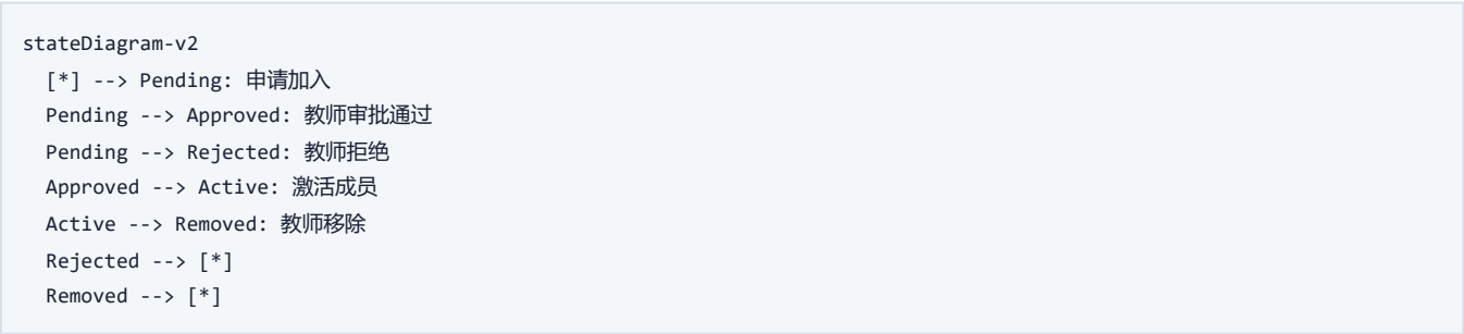
图 3-2-9 课程成员状态机
