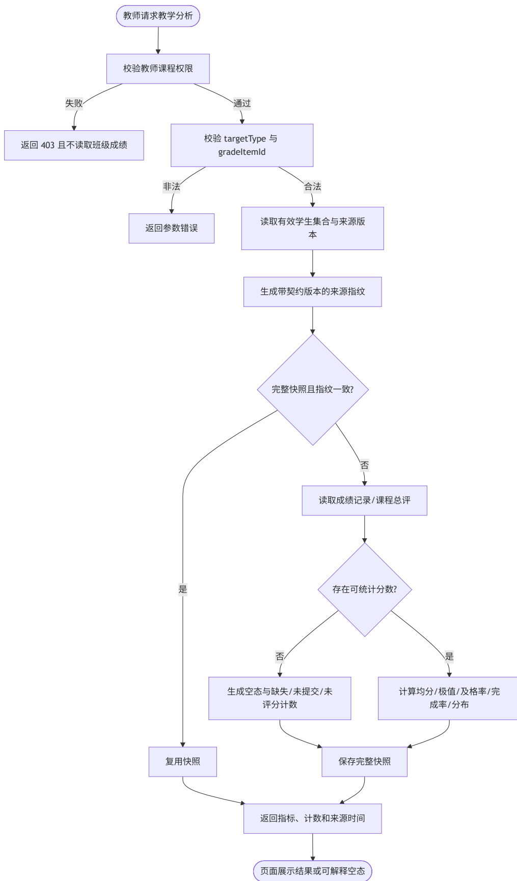
图 3-6-14 GRD 教学分析活动图
