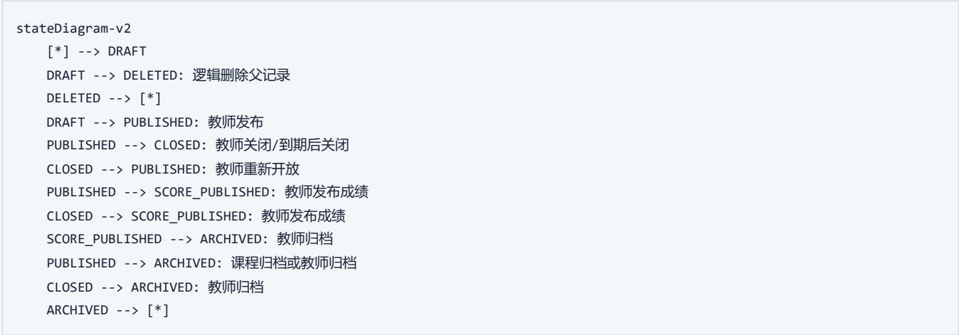
图 3-5-7 HWK 作业状态机
