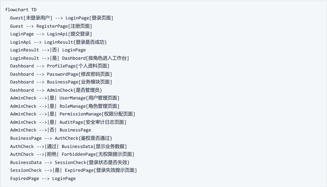
图 3-1 AUTH 页面流转图
