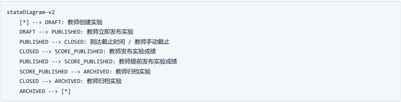
图 3-4-8 实验状态机
