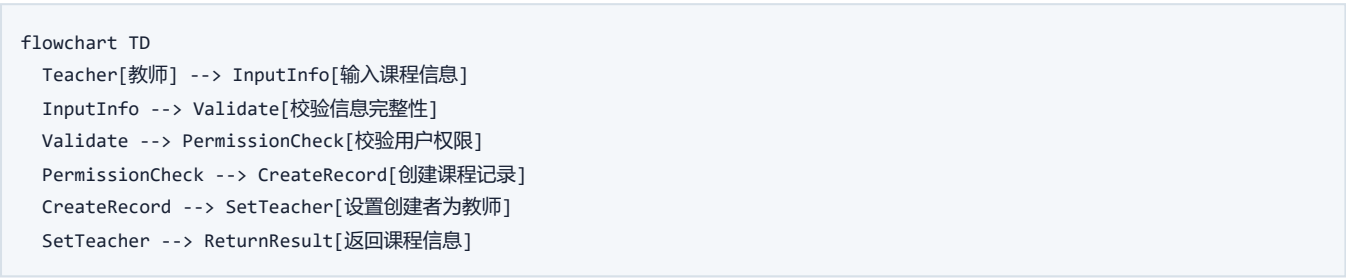
图 3-2-7 创建课程流程图
