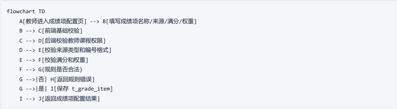
图 3-6-4 GRD 成绩项配置与规则校验流程图
