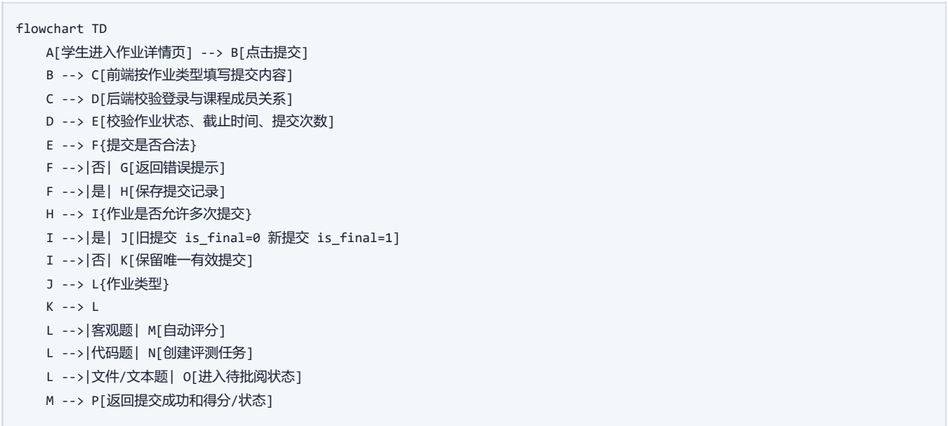
图 3-5-4 HWK 学生提交作业流程图
