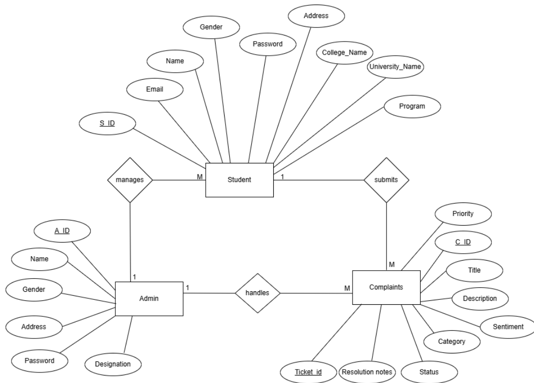
Figure 5. 5: ER Diagram
