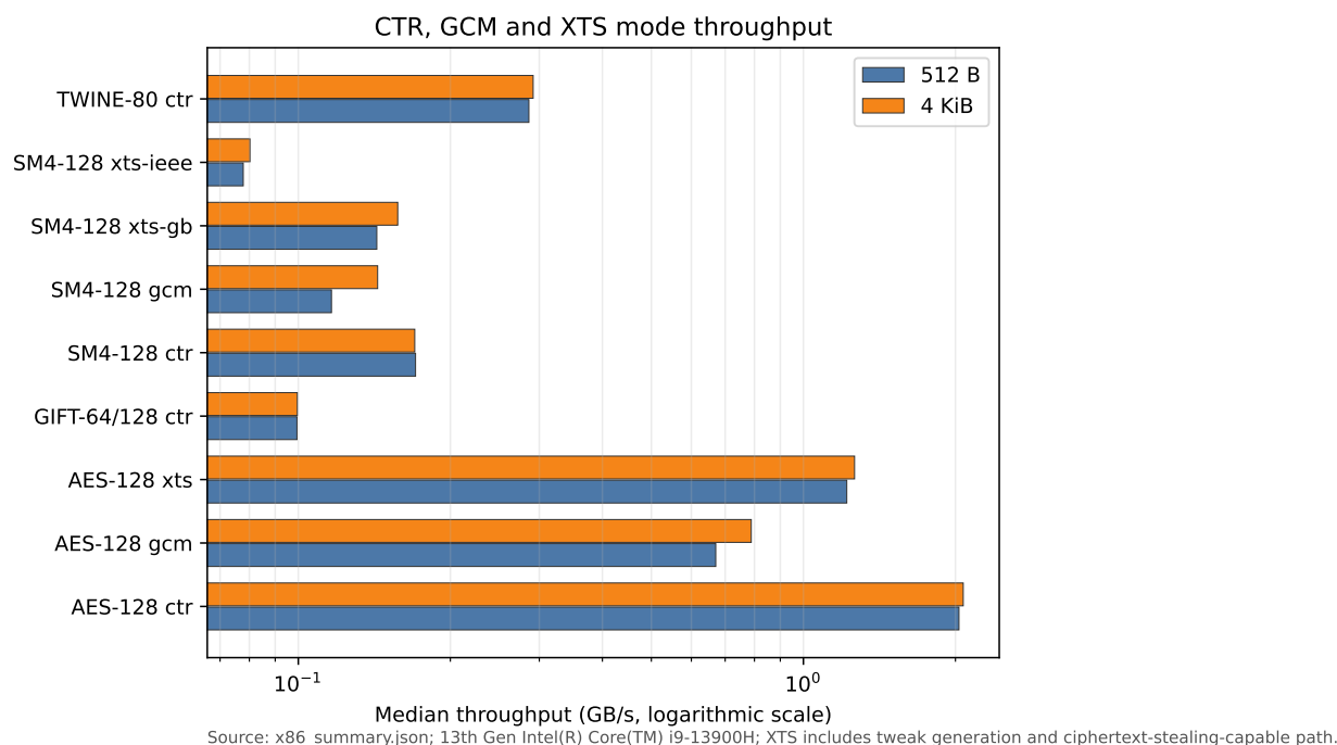
图 6: x86-64 上 CTR、GCM 与 XTS 的 512 B/4 KiB 吞吐率。
