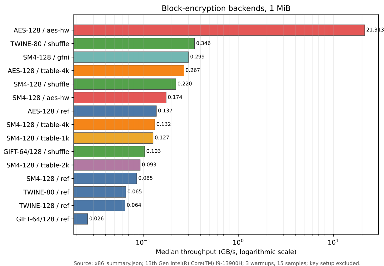
图 4: x86-64 上 1 MiB 分组加密吞吐率；数据来自独立 x86 汇总。
