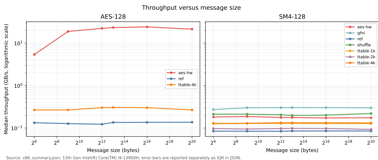
图 5: x86-64 上 AES/SM4 后端随消息长度的吞吐变化。
