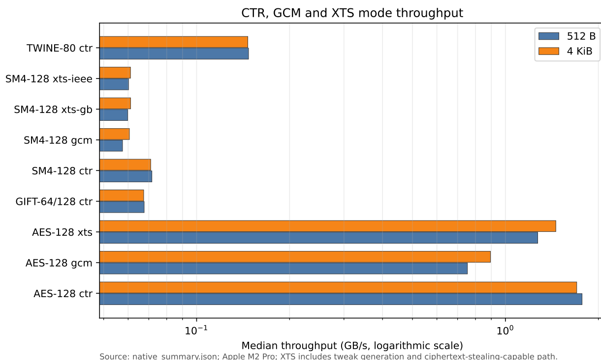
图 3: 512 B 与 4 KiB 的 CTR/GCM/XTS 吞吐率。
