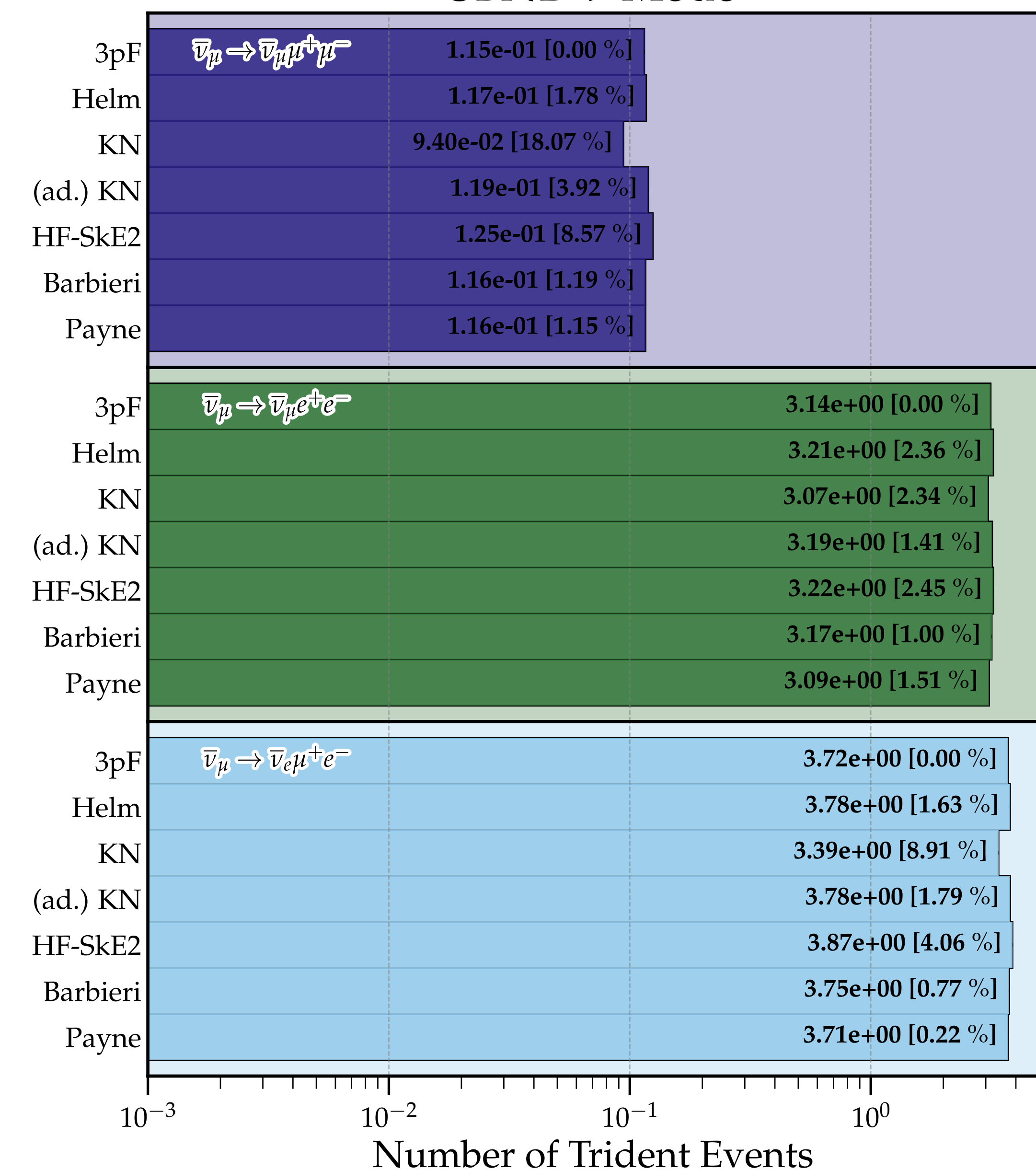
SBND \bar{\nu} -Mode
