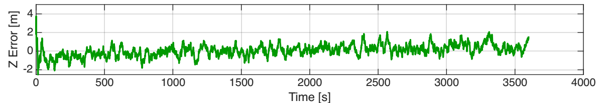
ECEF Position Error — Z
