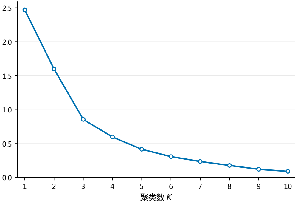
簇内平方和
