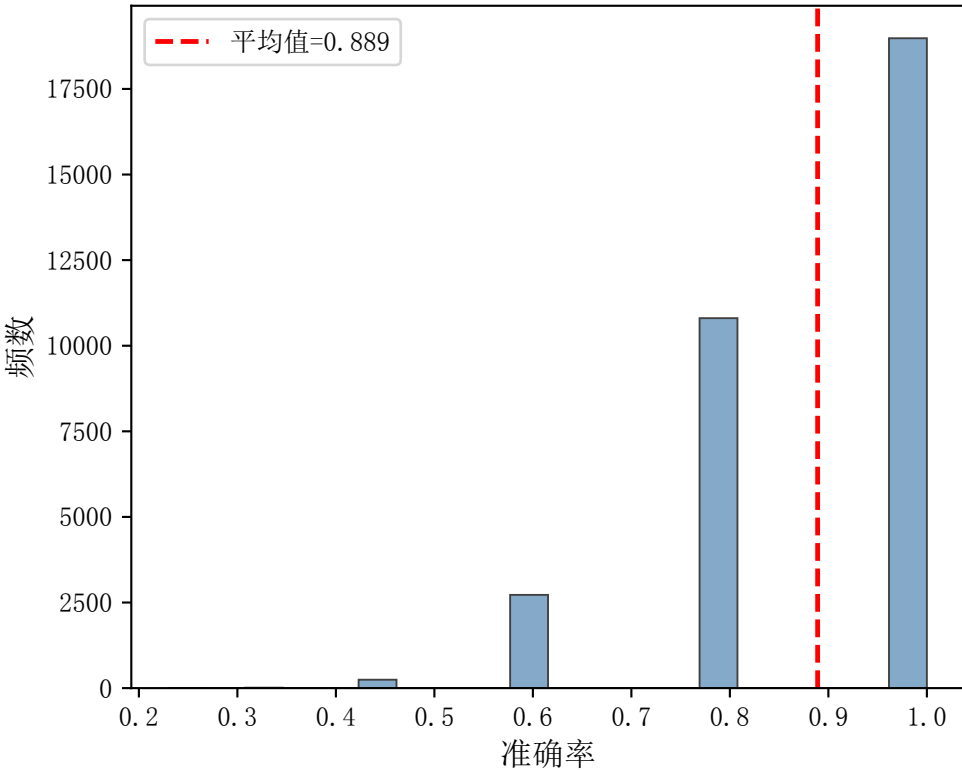
(a) 边类型预测准确率分布
