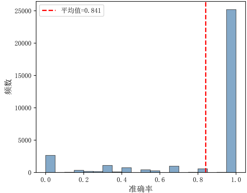
(b) 节点类型预测准确率分布
