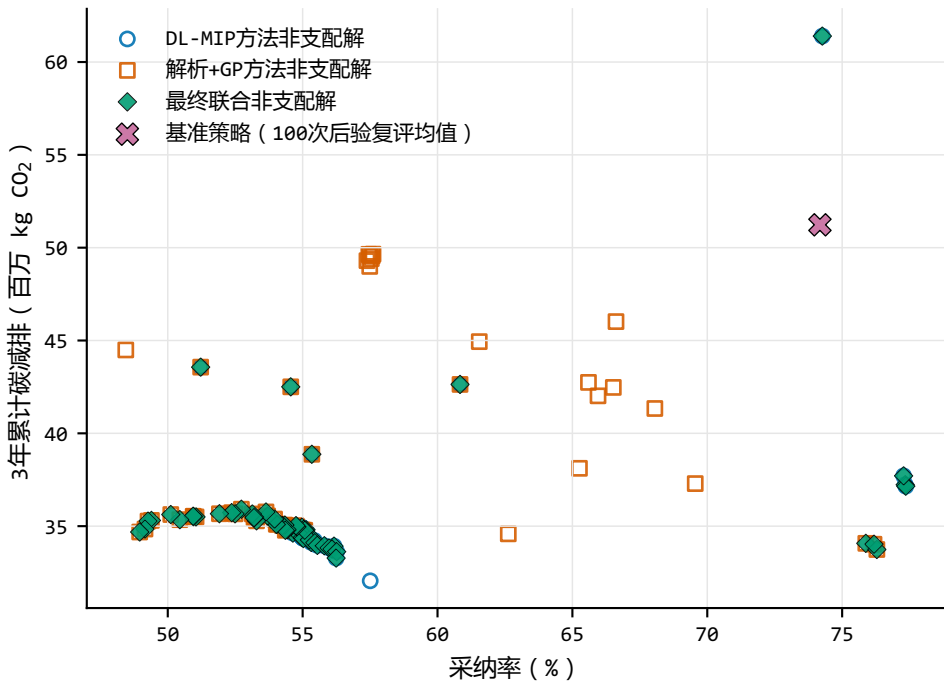
N=1000 的ABM真实Pareto投影
