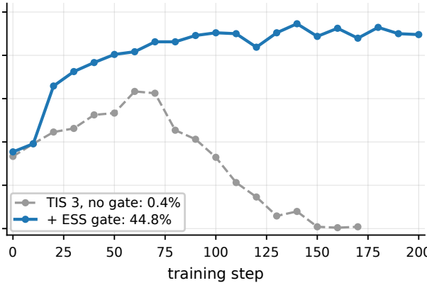
(d) TIS 3
