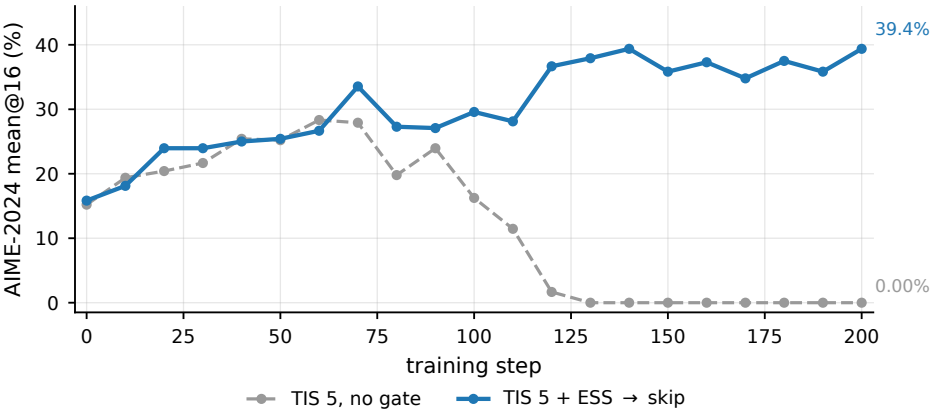
Qwen3-30B-A3B, TIS 5
