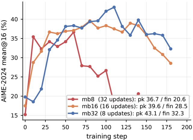
(a) AIME-2024
