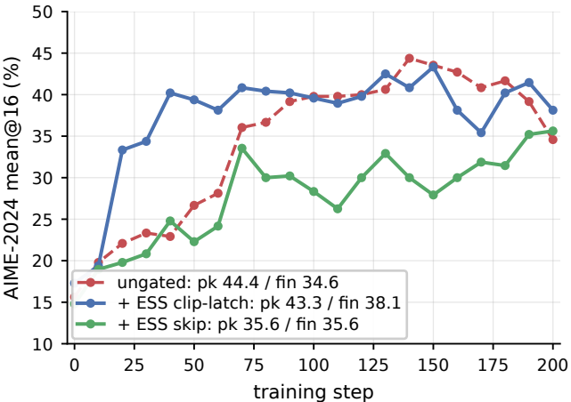
(a) AIME-2024
