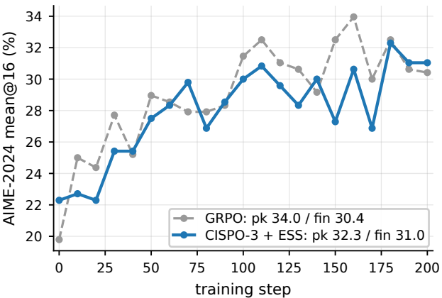
R1-1.5B: AIME-2024
