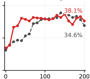
(d) GRPO-no clip
