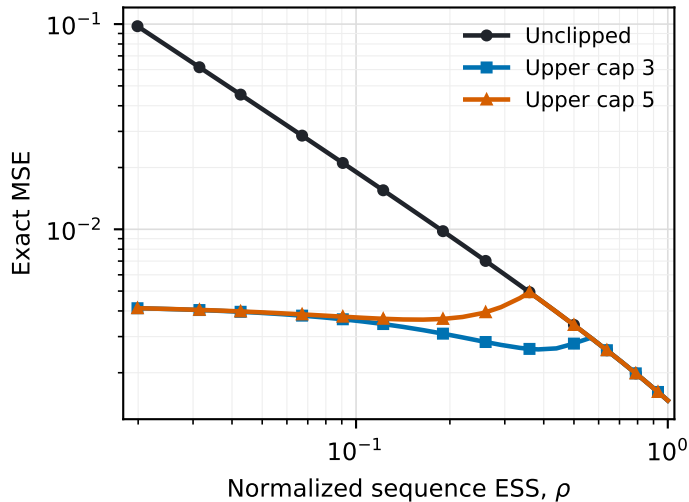
(a) Gradient MSE
